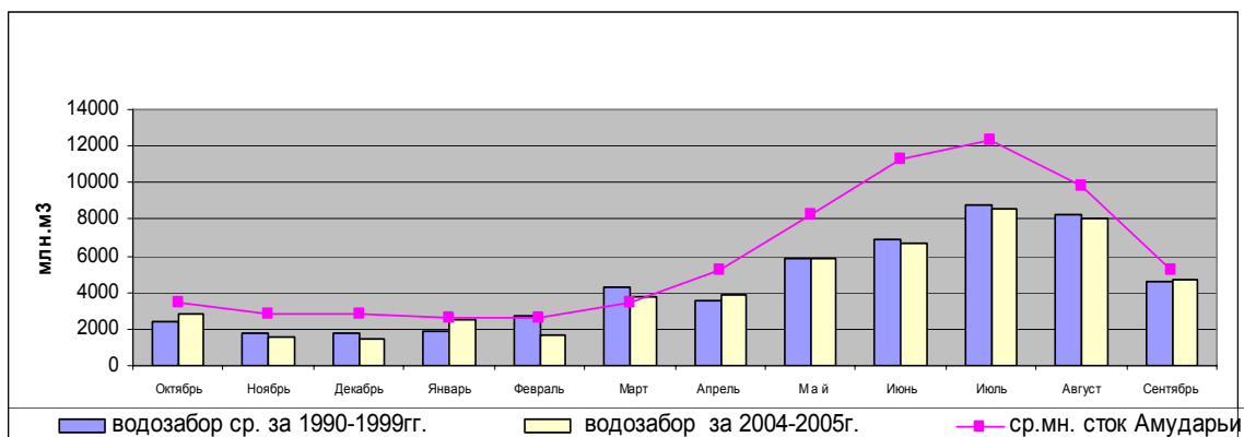
Рис. 1.1. Сравнение естественного стока Амурары с водозаборами из реки
