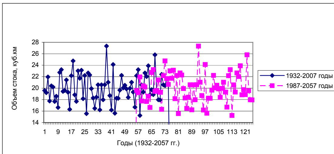
Рис. 3.10 Сравнение рядов годовых объемов стока реки Вахш на входе в Рогунское Водоохранилище: (1932-2007 гг.) факт – прогноз (1987-2057 гг.)
