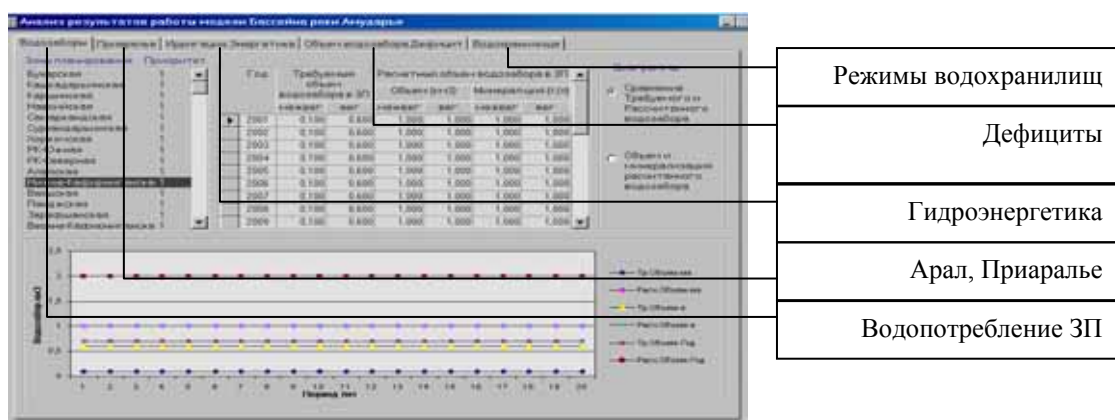
Рис 1.4.1. Главная форма БД МБА
