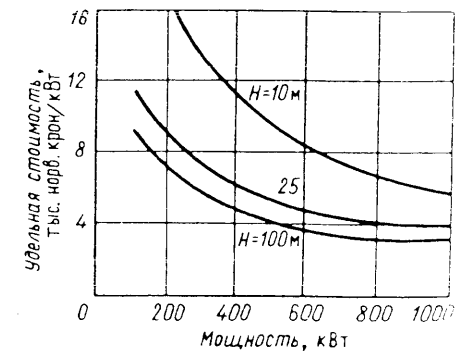
Рис. 7.4. Зависимость удельной стоимости строительства малых ГЭС в Норвегии от напора и мощности ГЭС
