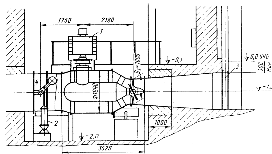
Рис. 4.25. Горизонтальный капсульный гидроагрегат с угловой передачей к генератору:
