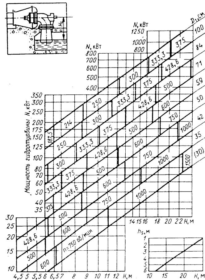
Рис. 4.1. Область применения гидротурбины Ф300-ГФ:
