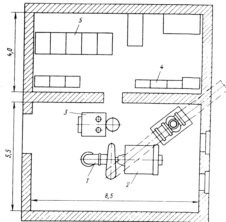
Рис. 4.32. Компоновка оборудования малой ГЭС:
