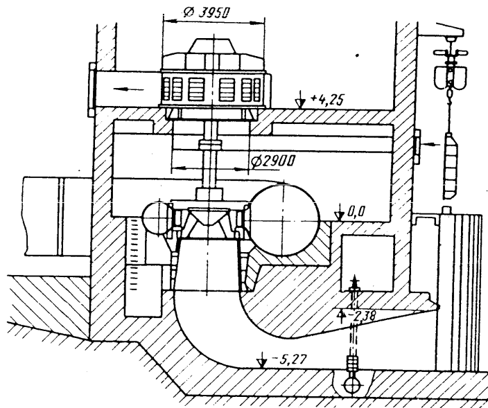
Рис. 4.26. Унифицированный гидроагрегат с РО гидротурбиной D_1 = 1,9 м
