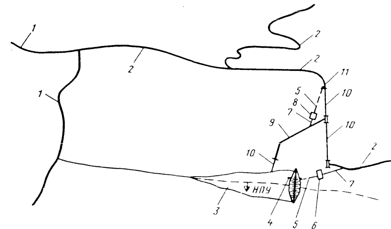
Рис. 3.8. Схема расположения малой ГЭС на переходах наполнения и опорожнения наливного водохранилища:
