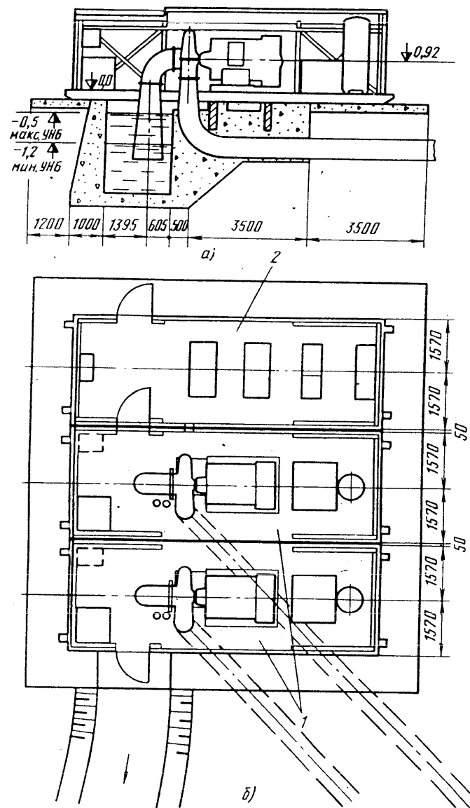
Рис. 3.18. Компонировка здания малой ГЭС из блок-секций: а – разрез; б – план; 1 – агрегатная блок-секция; 2 – секция управления и автоматики
