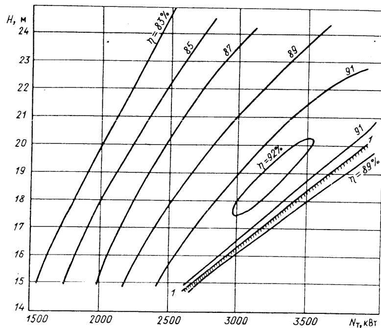
Рис. 4.27. Эксплуатационная характеристика гидротурбины РО 45/820-B-190: 1-1 — линия ограничения мощности
