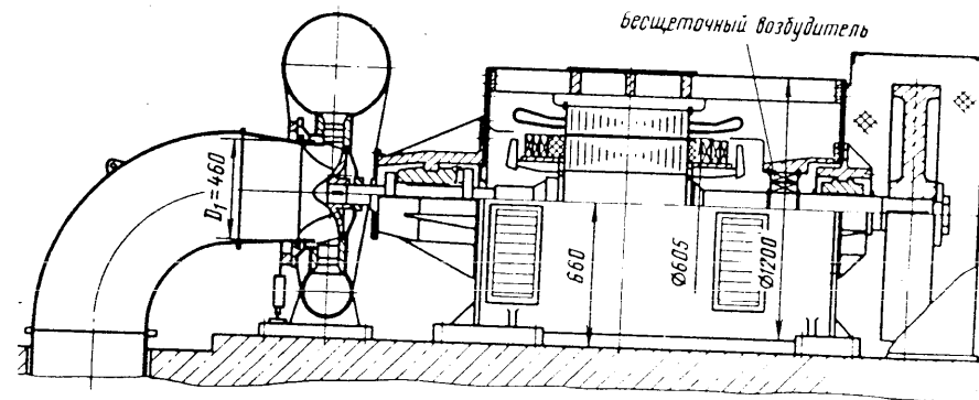
Рис. 4.17. Гидроагрегат с РО гидротурбиной мощностью 500 кВт
