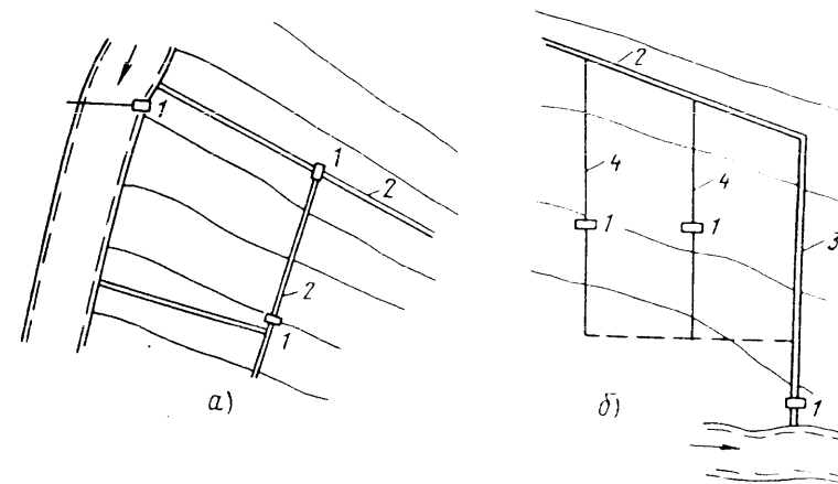
Рис. 3.9. Схемы расположения малой ГЭС на канале орошения:
