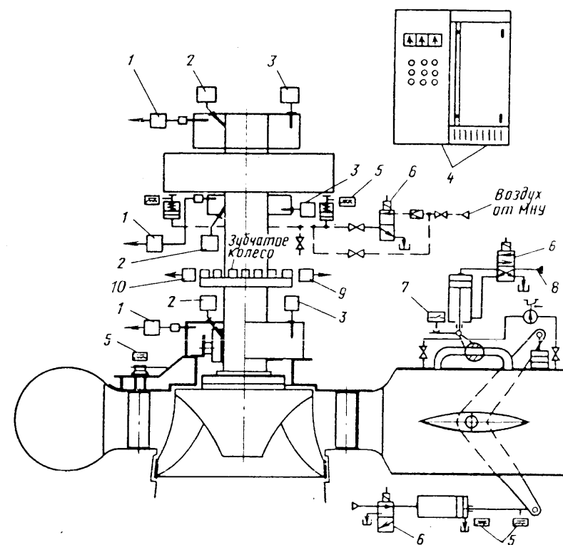
Рис. 4.31. Расположение устройств для управления гидротурбиной:
