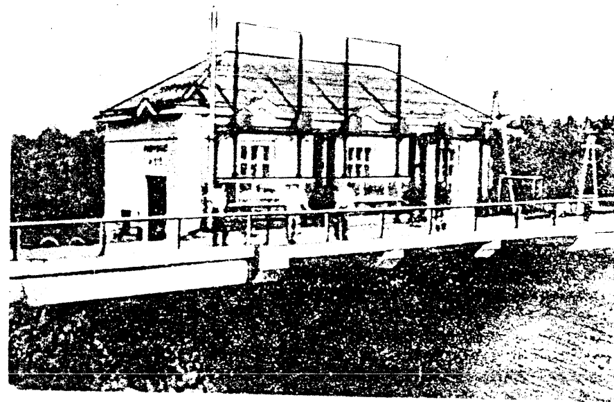
Рис. 1.4. ГЭС Падиснис на р. Дисна. Вид со стороны верхнего бьефа
