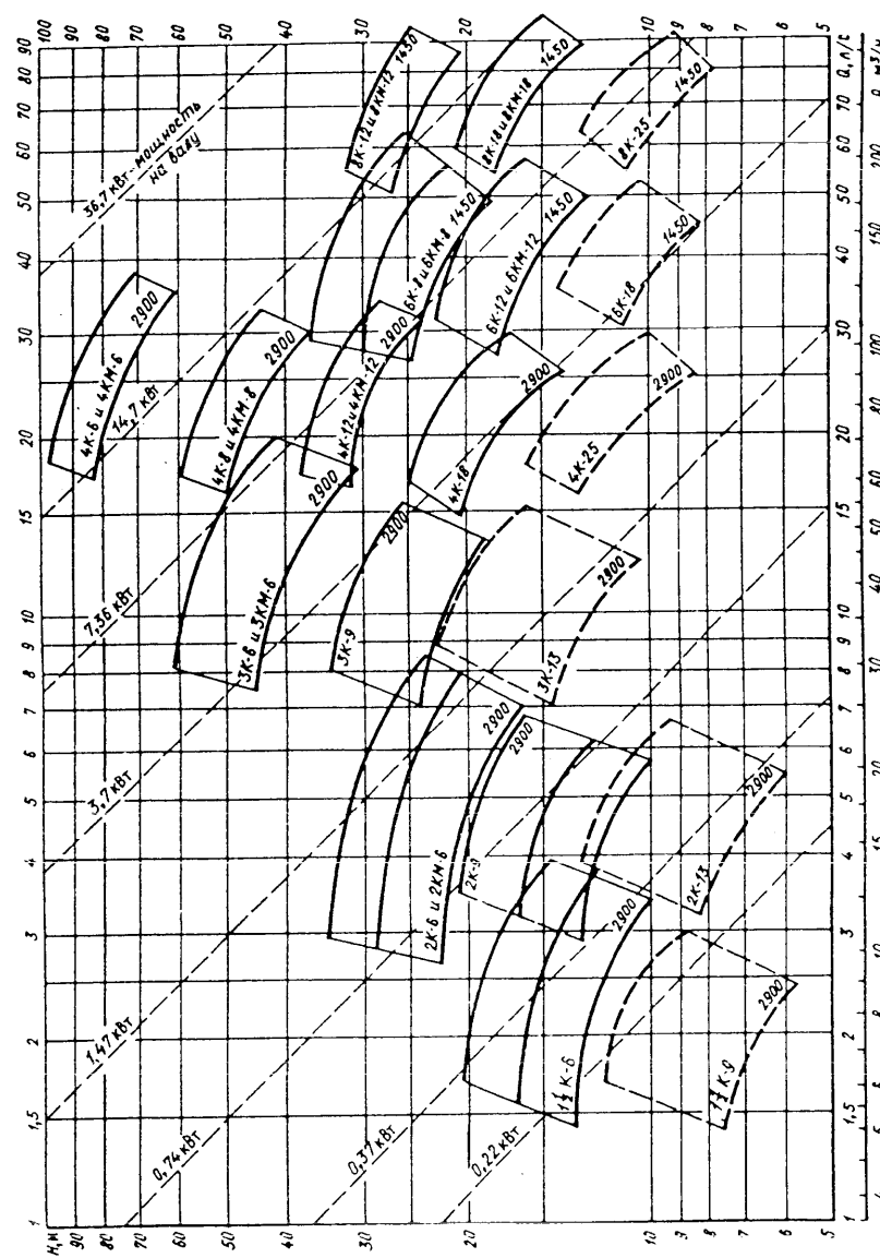
Рис. 4.13. Сводный график подачи и напоров одноступенчатых центробежных насосов типа К и моноблочных насосов типа КМ для чистой воды
