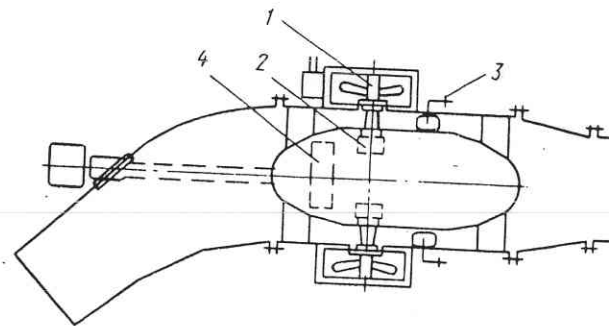
Рис. 7.10. Опытный малый магнитообъединенный гидроагрегат для напора 7,5 м, расчетной мощностью 136,5 кВт и переменной частотой тока от 40 до 80 Гц
