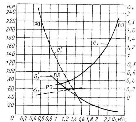
Рис. 4.12. Зависимости расчетного приведенного расхода от максимального напора Q_1' = f(H) и критического коэффициента кавитации от приведенного расчетного расхода \sigma_K = f(Q_1') для РО и ПЛ гидротурбин
