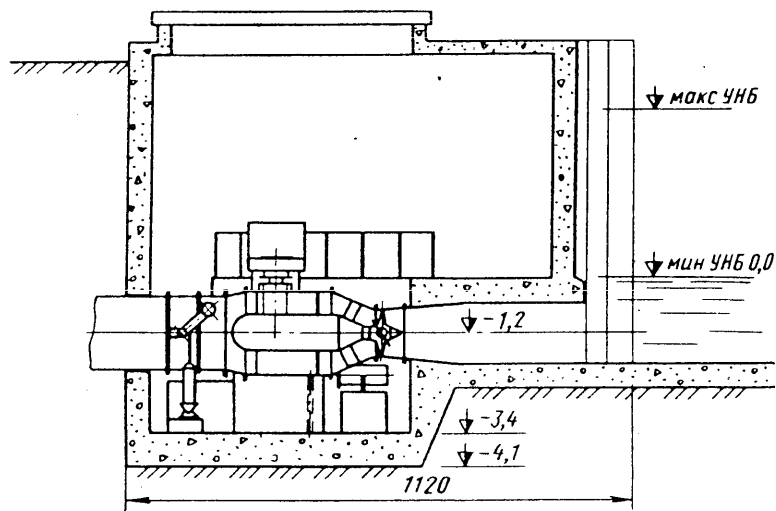
Рис. 3.12. Компоновка здания малой ГЭС с горизонтальной капсульной гидротурбиной и вынесенным в машинный зал вертикальным генератором
