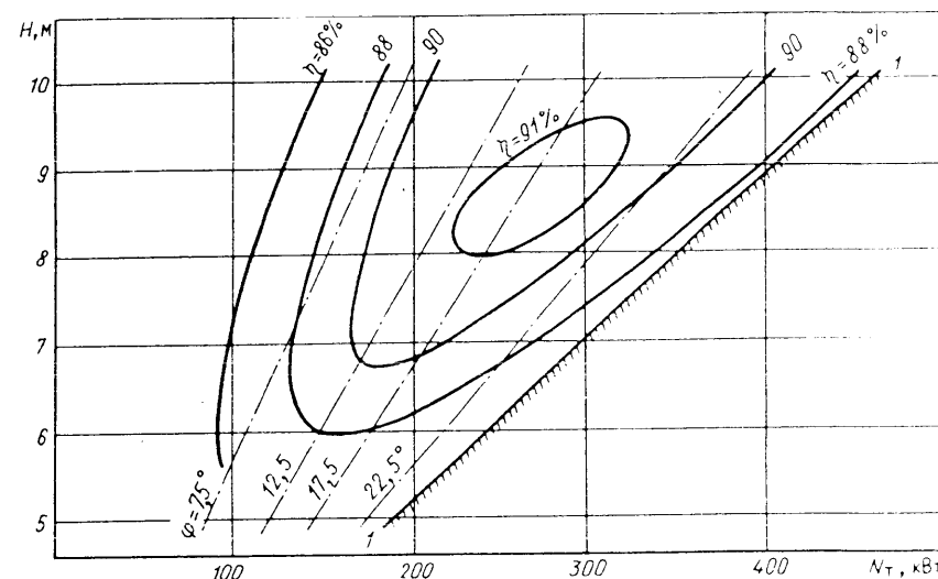
Рис. 4.22. Эксплуатационная характеристика гидротурбины ПЛ 15/811-В-100:
