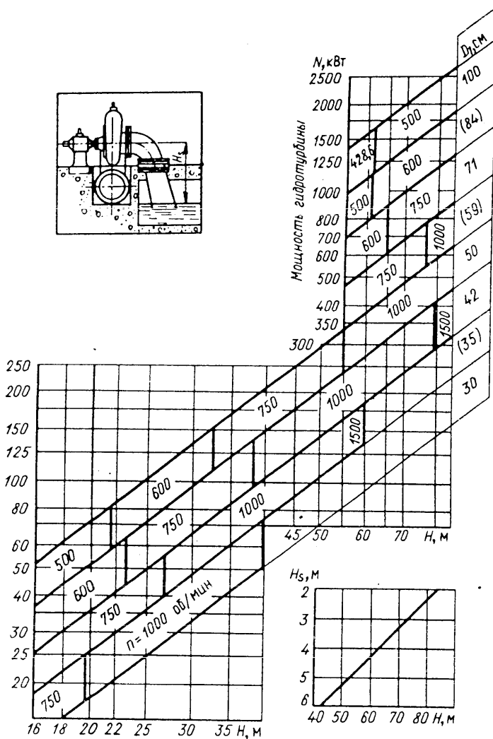
Рис. 4.2. Область применения гидротурбины Φ13-ГМ:
