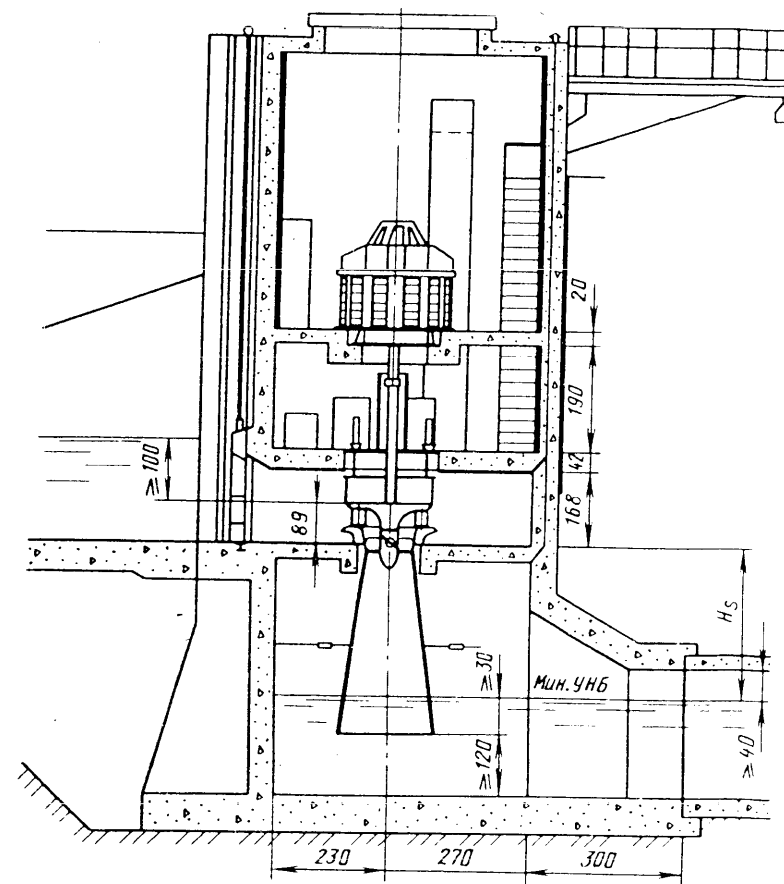
Рис. 3.13. Компоновка здания малой ГЭС с вертикальной осевой гидротурбиной с забором воды непосредственно в турбинную камеру
