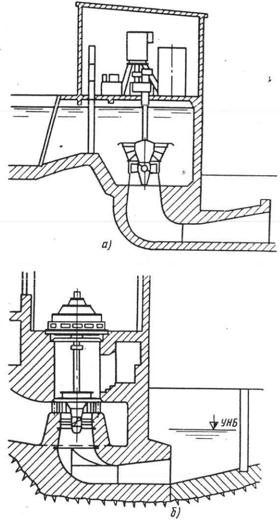
Рис. 7.7. Типовые компоновки агрегатных блоков низко-напорных малых ГЭС:
