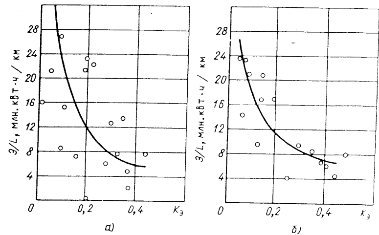
Рис. 2.1. Графики зависимости k_3 = f(E/L) для горных (а) и равнинных (б) рек европейской части СССР мощностью 100–200 тыс.кВт
