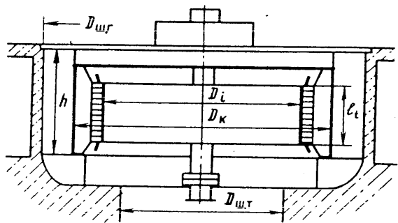
Рис. 4.16. Габариты гидрогенератора
