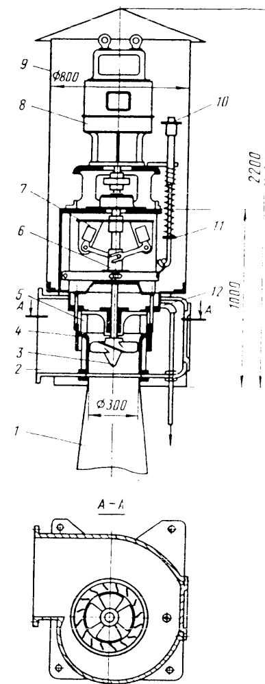
Рис. 4.3. Гидроагрегат микроГЭС конструкции И.В. Котенева:
