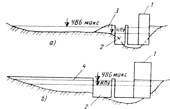
Рис. 3.4. Схема пропуска паводка:
