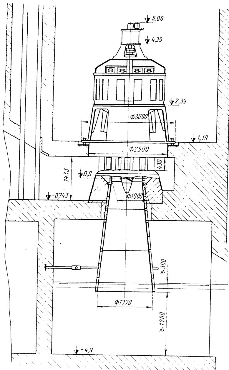
Рис. 4.23. Унифицированный гидроагрегат с пропеллерной гидротурбиной ( H = 10 м, n = 428,6 об/мин, N = 500 кВт)
