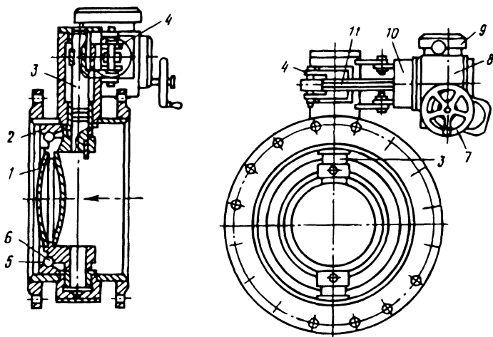
Рис. 3.18. Дискový поворотный затвор:
