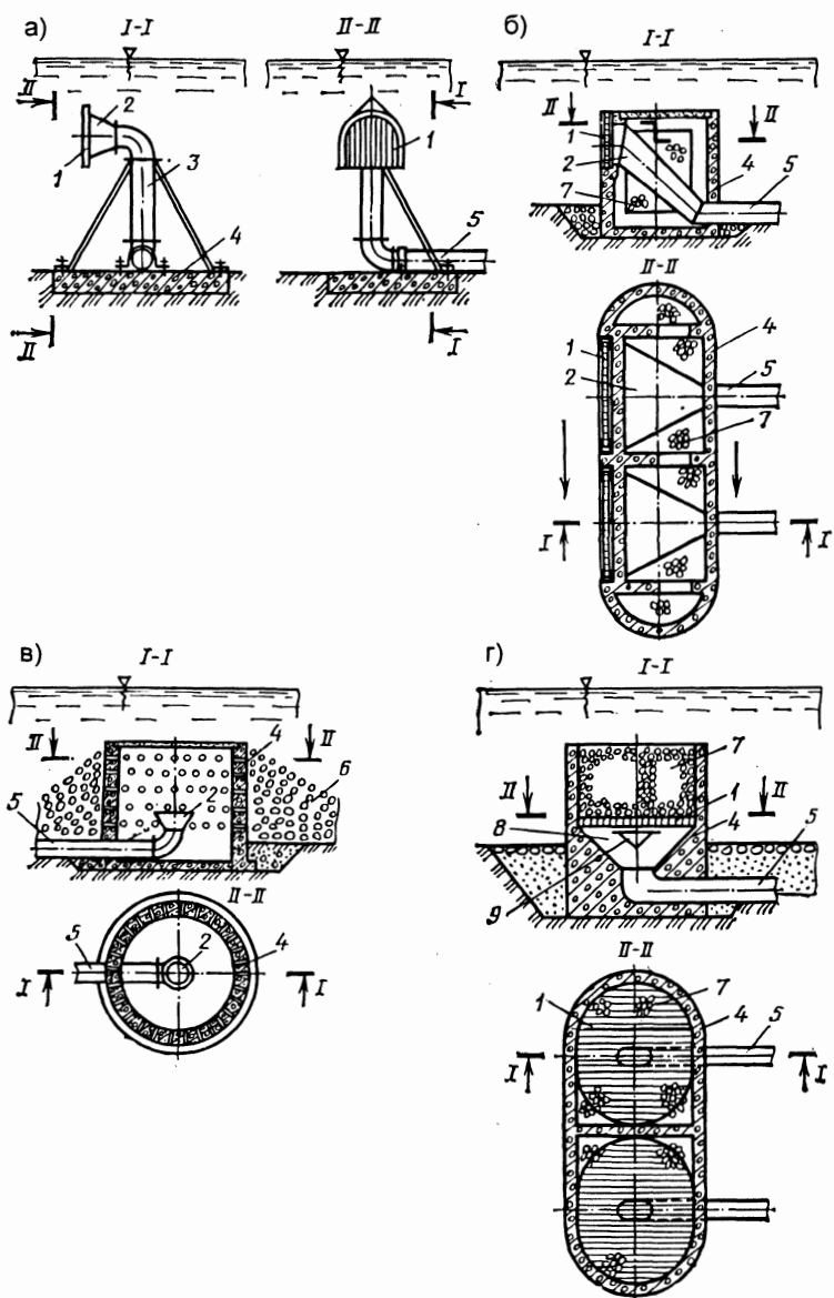
Рис. 4.20. Типы оголовков:
