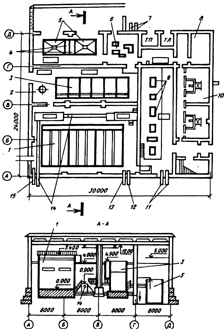
Рис. 5.39. Пример компоновки водоочистных сооружений: 1 — осветлители со взвешенным осадком; 2 — смесители; 3 — скорые фильтры; 4 — расходные баки коагулянта; 5 — растворные баки-хранилища коагулянта; 6 — насосы-дозаторы и воздухоудвки; 7 — подача чистой воды потребителю; 8 — мастерские; 9 — насосная станция II подъема; 10 — бытовые помещения; 11 — всасывающие трубопроводы из резервуаров чистой воды; 12 — отвод чистой воды в резервуары; 13 — сброс осадка из осветлителей; 14 — сброс промывной воды от фильтров; 15 — подача исходной воды
