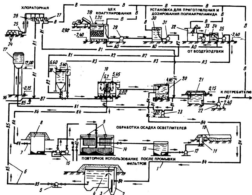
Рис. 5.37. Высотн-технологическая схема водоочистного комплекса: 1 — подача промывной воды от фильтров; 2 — песколовка; 3 — гидроэлеватор; 4 — резервуар-усреднитель промывной воды; 5 — насос перекачки промывной воды; 6 — возврат промывной воды на очистные сооружения; 7 — подача осадка от осветлителей; 8 — резервуар приема осадка; 9 — установка медленного перемешивания осадка; 10 — площадка обезвоживания осадка; 11 — колодец для напуска осадка; 12 — насос перекачки сгущенного осадка; 13 — емкость сгущенного осадка; 14 — осадкоуплотнитель; 15 — насосы перекачки сырого осадка; 16 — подача исходной воды; 17 — башня промывной воды; 18 — вихревой смеситель; 19 — осветлитель со взвешенным осадком; 20 — скорый фильтр; 21 — резервуар чистой воды; 22 — насос II подъема; 23 — насос подкачки промывной воды; 24 — бочки с хлором; 25 — испаритель; 26, 27 — хлораторы первичного и вторичного хлорирования; 28 — растворно-хранилищный бак коагулянта; 29 — насос перекачки раствора коагулянта; 30 — расходный бак коагулянта; 31 — насос-дозатор раствора коагулянта; 32 — мешалка полиакриламида ПАА; 33 — насос для циркуляции и подачи ПАА в расходный бак; 34 — растворный бак раствора ПАА; 35 — насос-дозатор раствора ПАА
