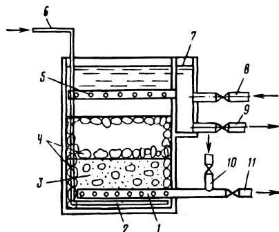
Рис. 5.21. Схема устройства каркасно-засыпного скорого фильтра: 1, 2 — водо- и воздухораспределительные системы; 3 — песчаная за- сыпка в межгравийном пространстве; 4 — гравийный каркас; 5 — труб- чатая перфорированная система распределения исходной и сбора про- мывной воды; 6 — подача воздуха; 7 — боковой карман; 8, 11 — пода- ча исходной и отвод фильтрованной воды; 9, 10 — отвод и подача промывной воды
