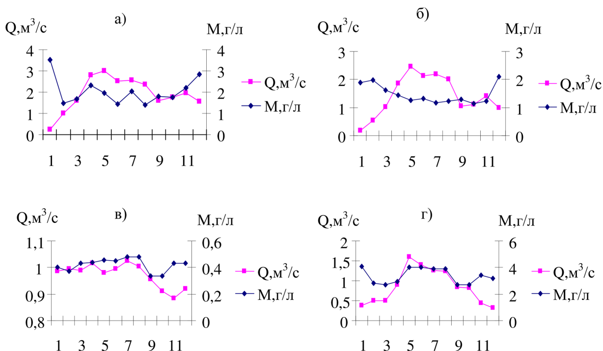
Рис. 3. Внутригодовые изменения расходов воды ( Q , \text{м}^3/\text{с} ) и минерализации ( M , \text{г/л} ) в крупных коллекторах Сурхандарьинской области в среднем за 2003-2006 гг.: а) МС; б) Ангор; в) К-2 Денов; г) К-2 Музрабод.
