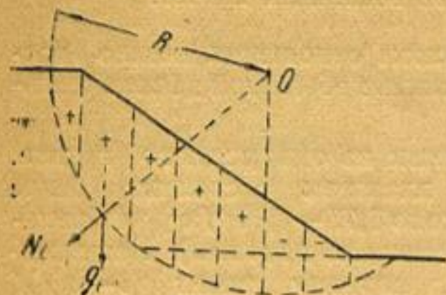
Рис. 15. К расчету устойчивости откоса
