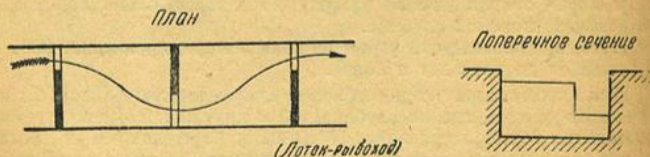
Рис. 188. Лоток-рыбоход
