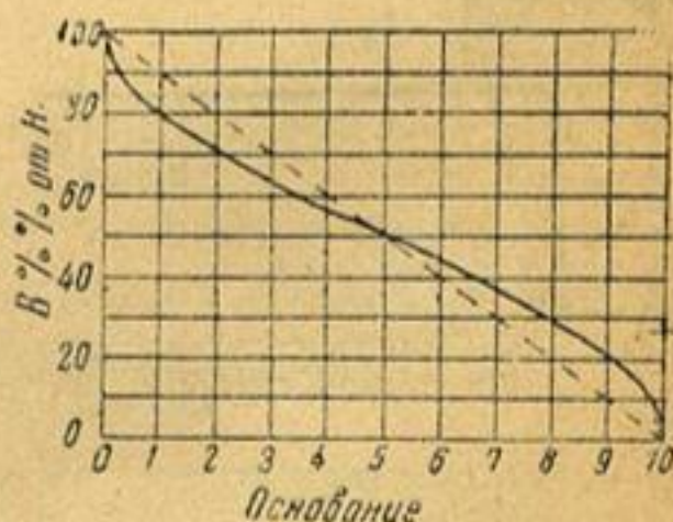
Рис. 141. Эпюра фильтрационного давления для бесшпунтового контура № 1
