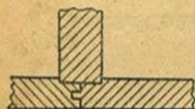
Рис. 96. Вертикальный опорный шов водосливной плиты водослива малой высоты
