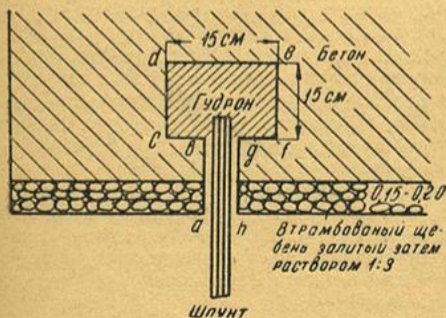
Рис. 157. Заделка шпунта при ожидаемой осадке водослива
