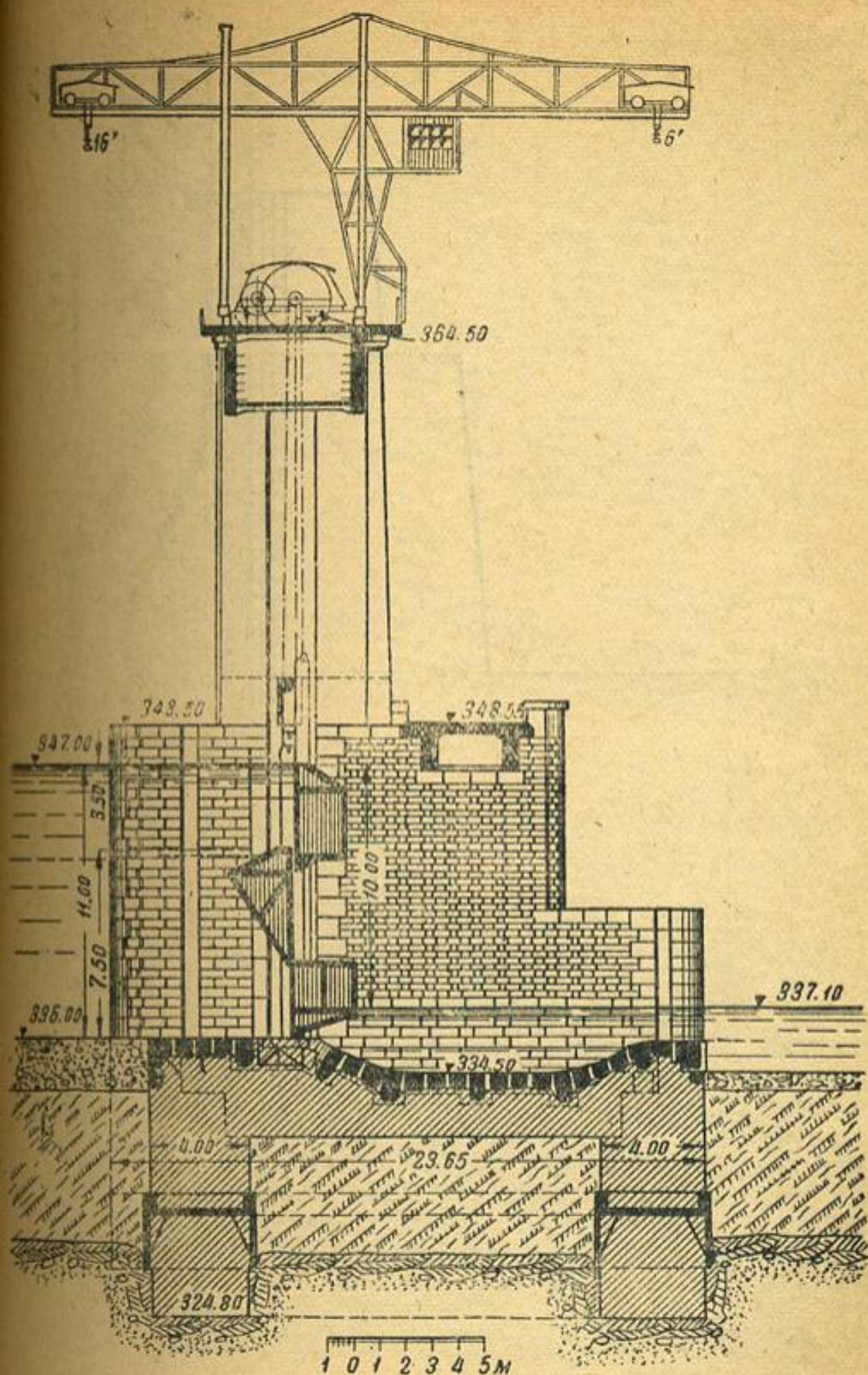
Рис. 68. Водослив с пониженным порогом (Шанси-Пуны)
