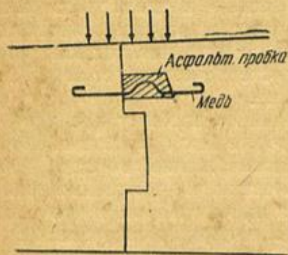
Рис. 101. Шов с замком, асфальтовой шпонкой и медной пластинкой
