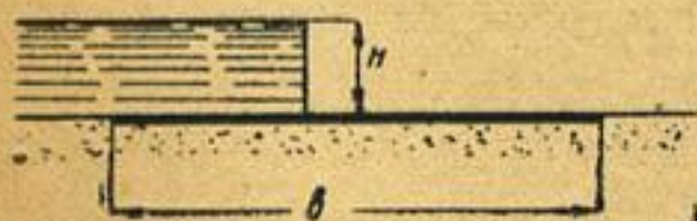
Рис. 132. Бесшпунтовый фильтрационный контур (№ 1)
