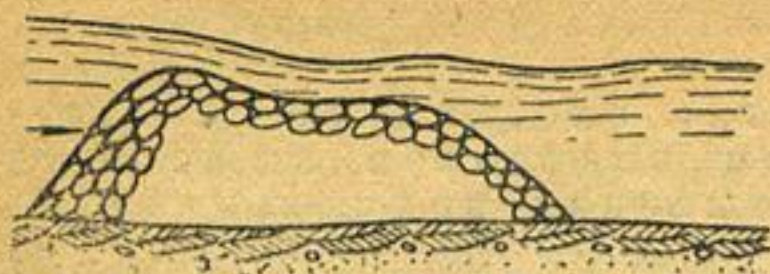
Рис. 197. Третья стадия работы наброски в текущую воду
