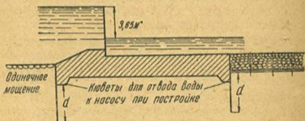
Рис. 154. Профиль Нижне-Куindrючской плотины
