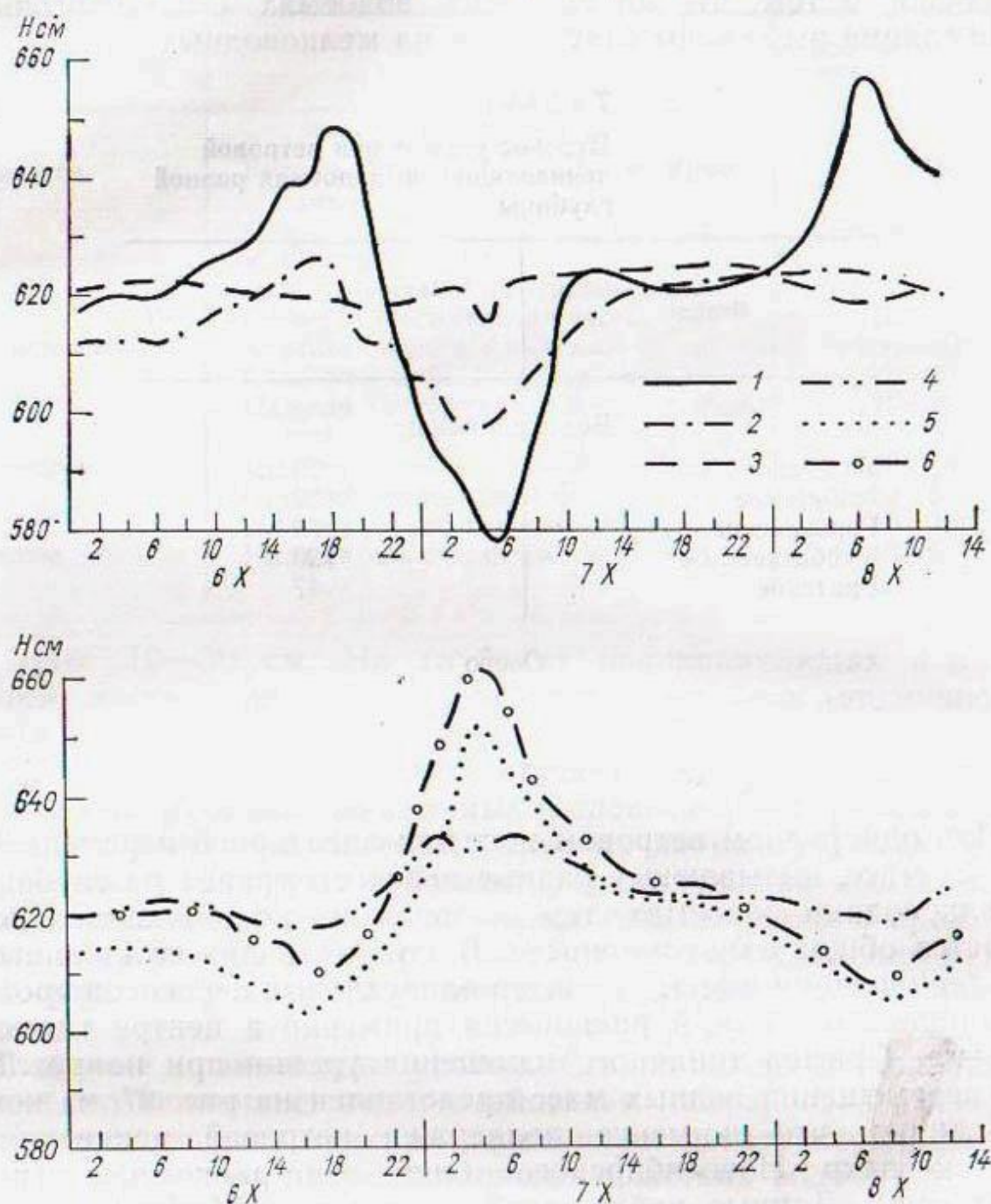
Рис. 27. Ход уровней на постах вдхр Новосибирского при штормовом ветре 6—8/X 1961 г.
