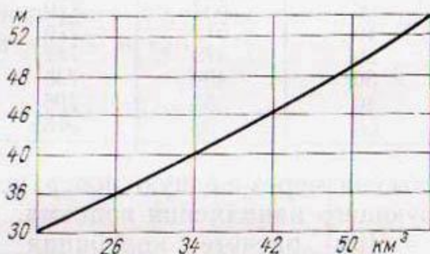
Рис. 29. Зависимость уровня равновесия от поверхности притока в Аральское море (по Б. Д. Зайкову).
