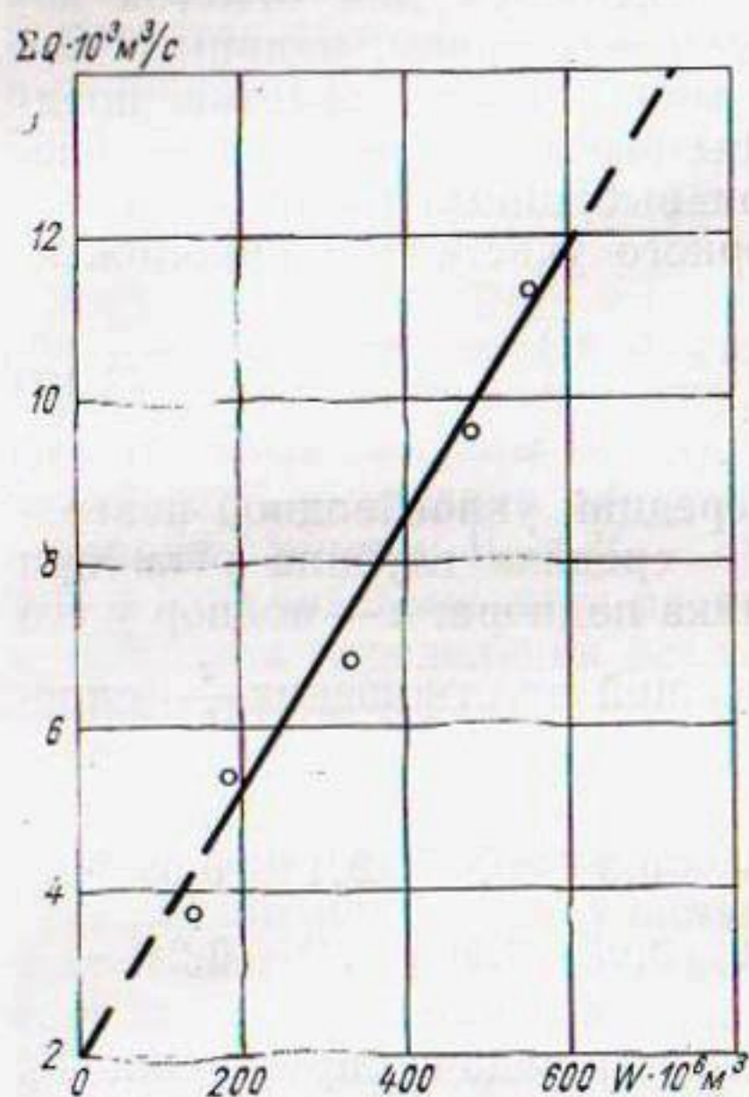
Рис. 7. Зависимость запаса воды в зонах выклинивания подпора главных притоков вдхр Рыбинского от суммарного расхода воды (по Ф. И. Белых).
