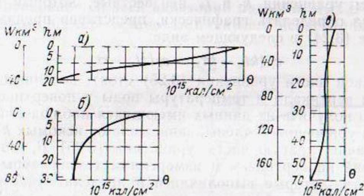
Рис. 15. Пример определения теплозапасов графическим методом с учетом распределения объемов по слоям различной глубины (а, б, в).
