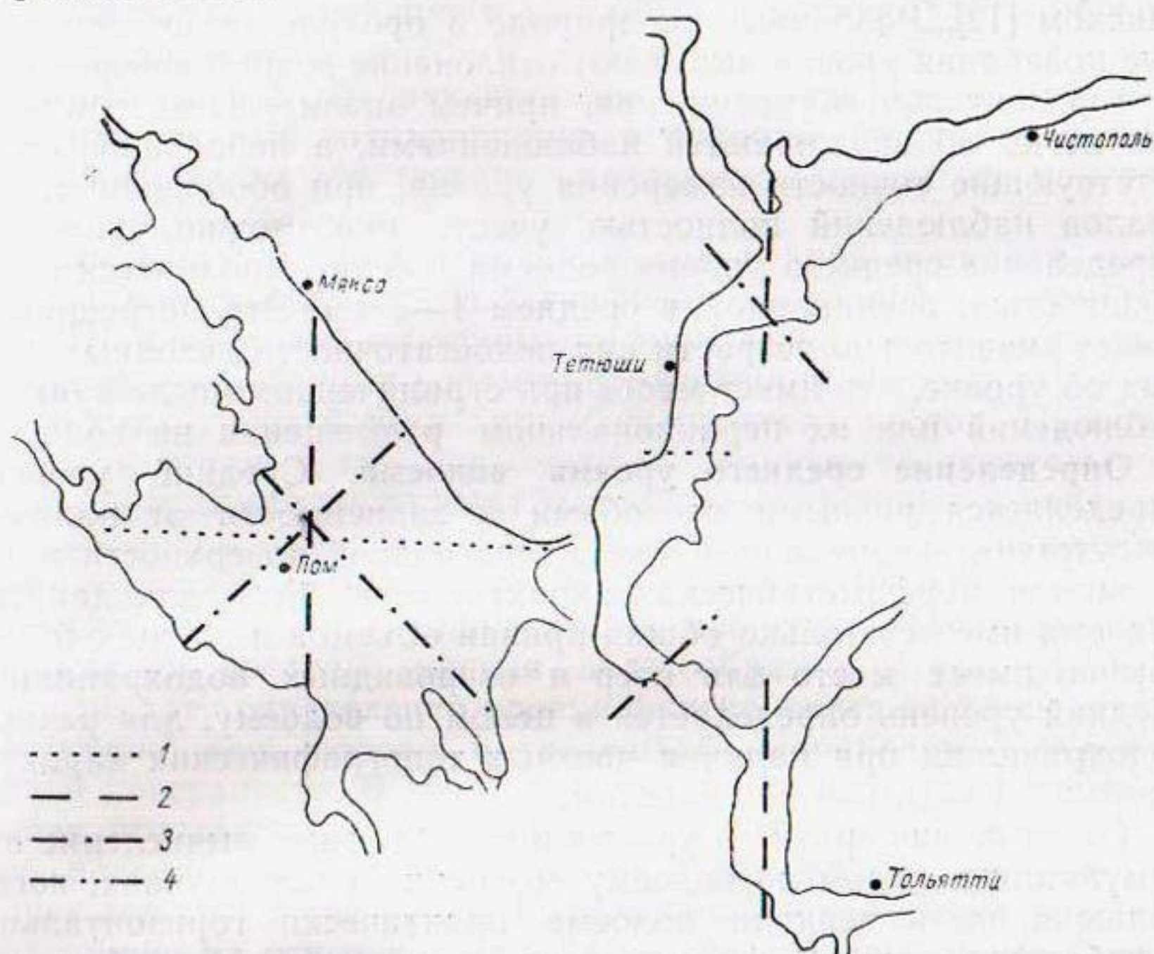
Рис. 28. Расположение осей равновесия на водохранилищах Рыбинском и Куйбышевском при ветре различных направлений.
