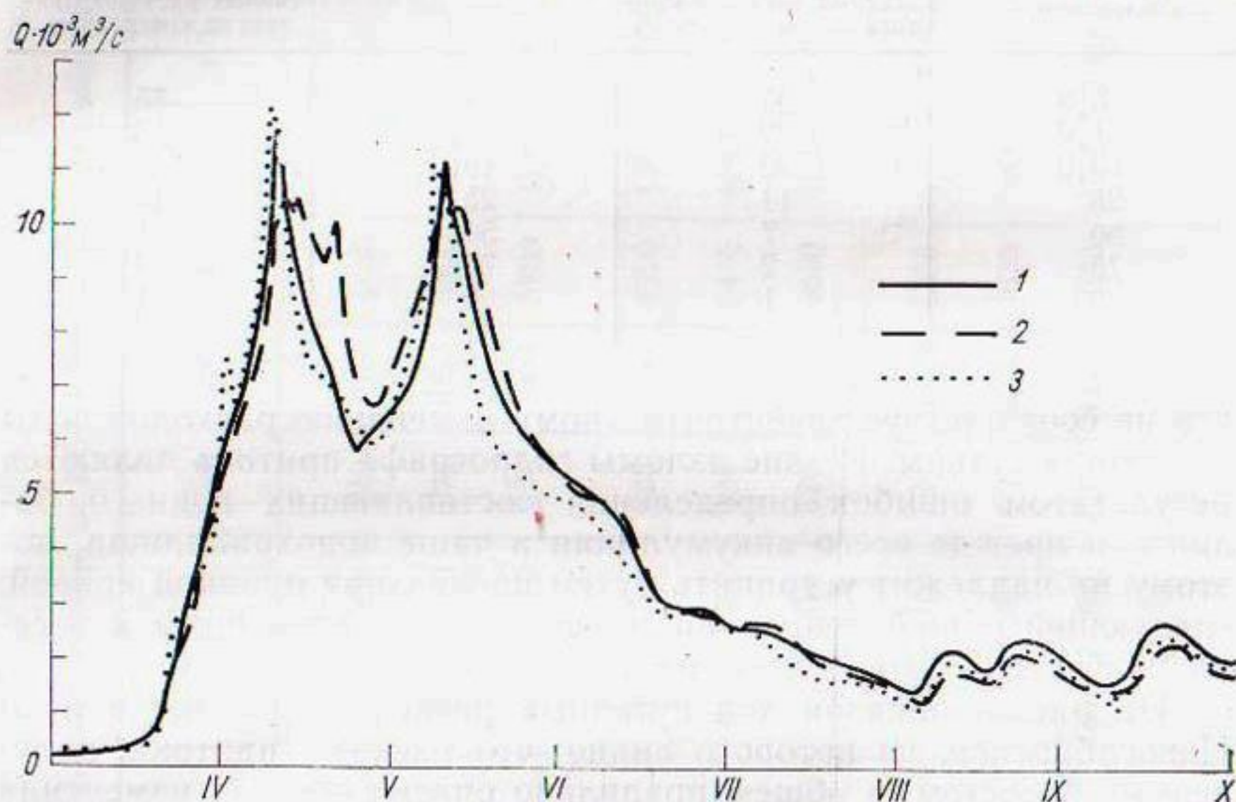
Рис. 8. Приток воды в водхр Новосибирское, 1969 г.
