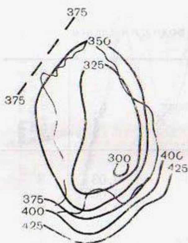
Рис. 9. Распределение средних многолетних жидких осадков (мм) над поверхностью оз. Ладожского (по Е. А. Попову).
