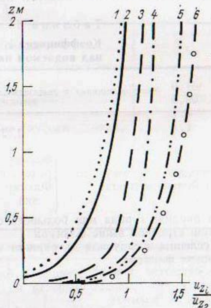
Рис. 12. Профили ветра в различном удалении от уреза берега оз. Валдайского.
