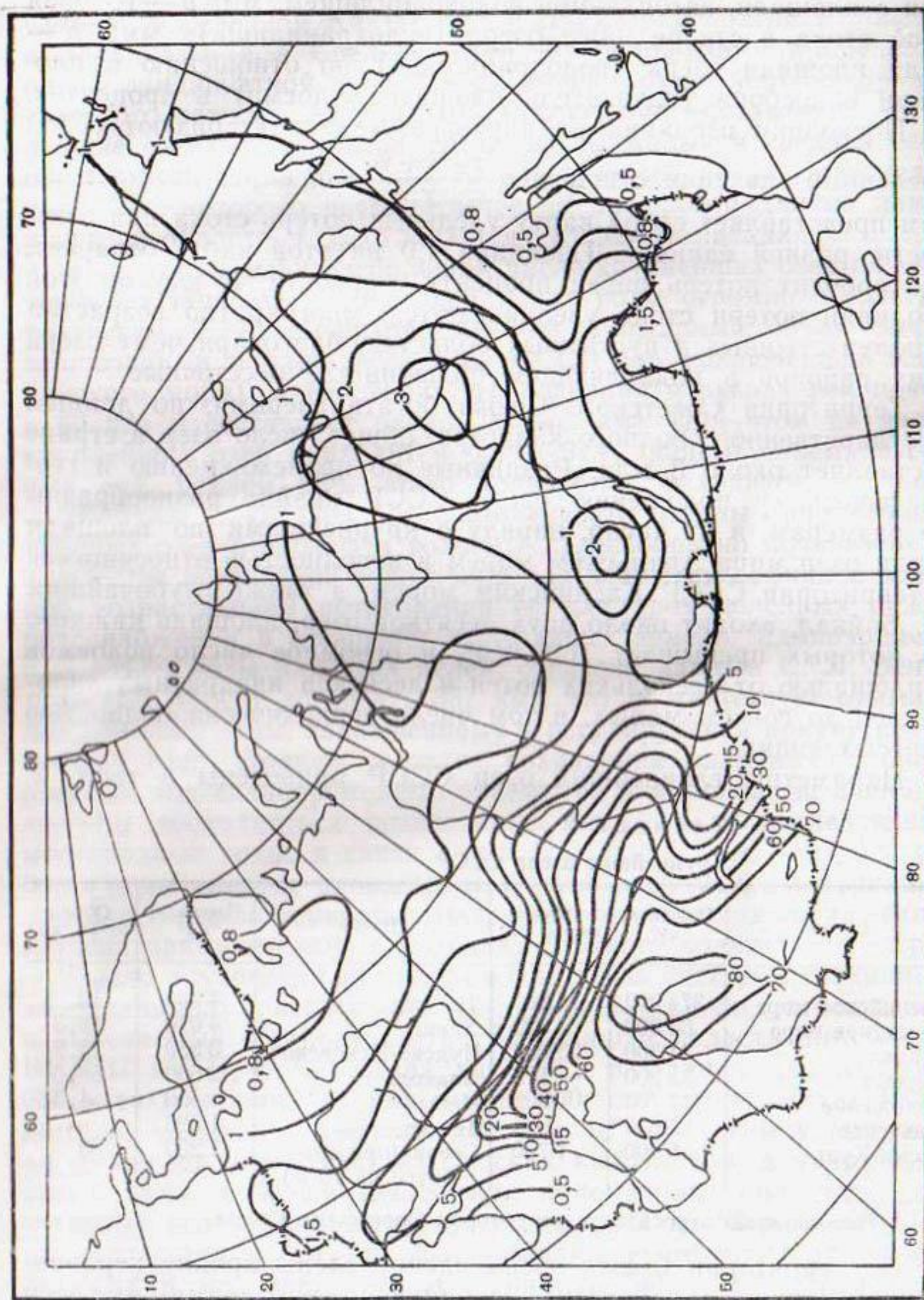
Рис. 1. Карта изолиний параметра a = \frac{z - x + y_1}{y} (по А. А. Соколову).
