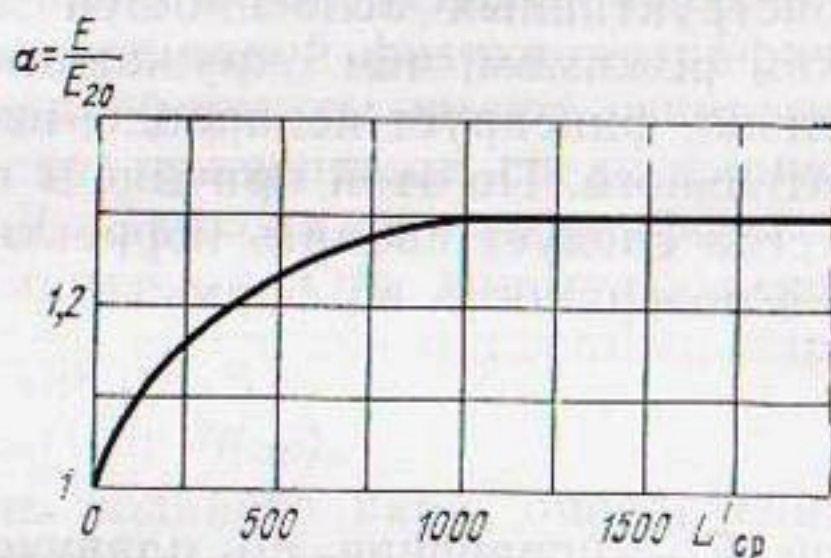
Рис. 16. Зависимость коэффициента \alpha от длины разгона воздушного потока над водоемом L' .
