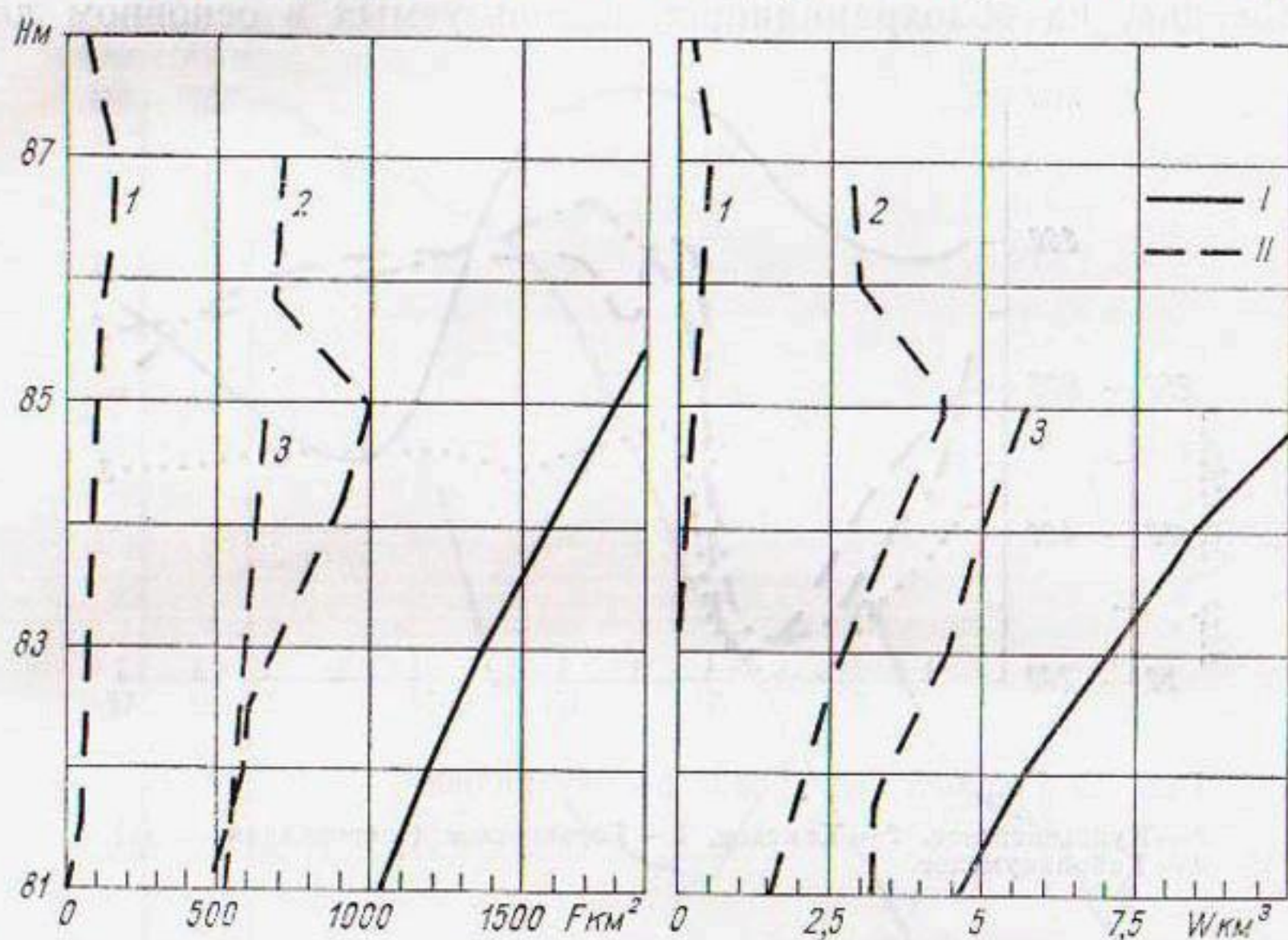
Рис. 24. Кривые площадей и объемов вдхр Горьковского.
