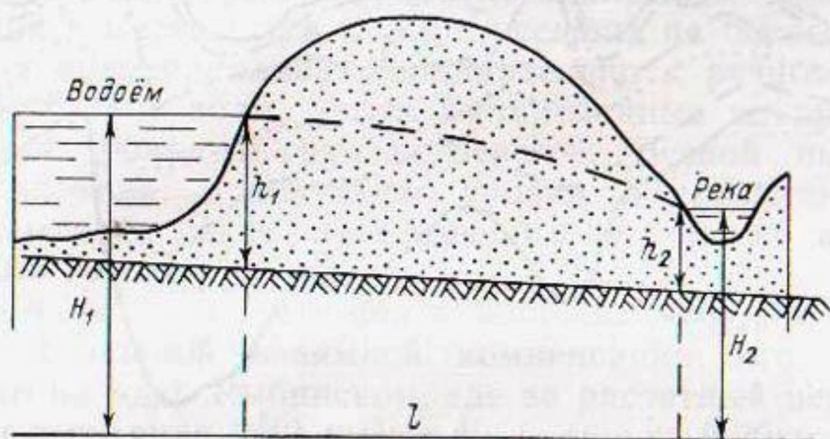
Рис. 20. Схема фильтрации через водораздел.
