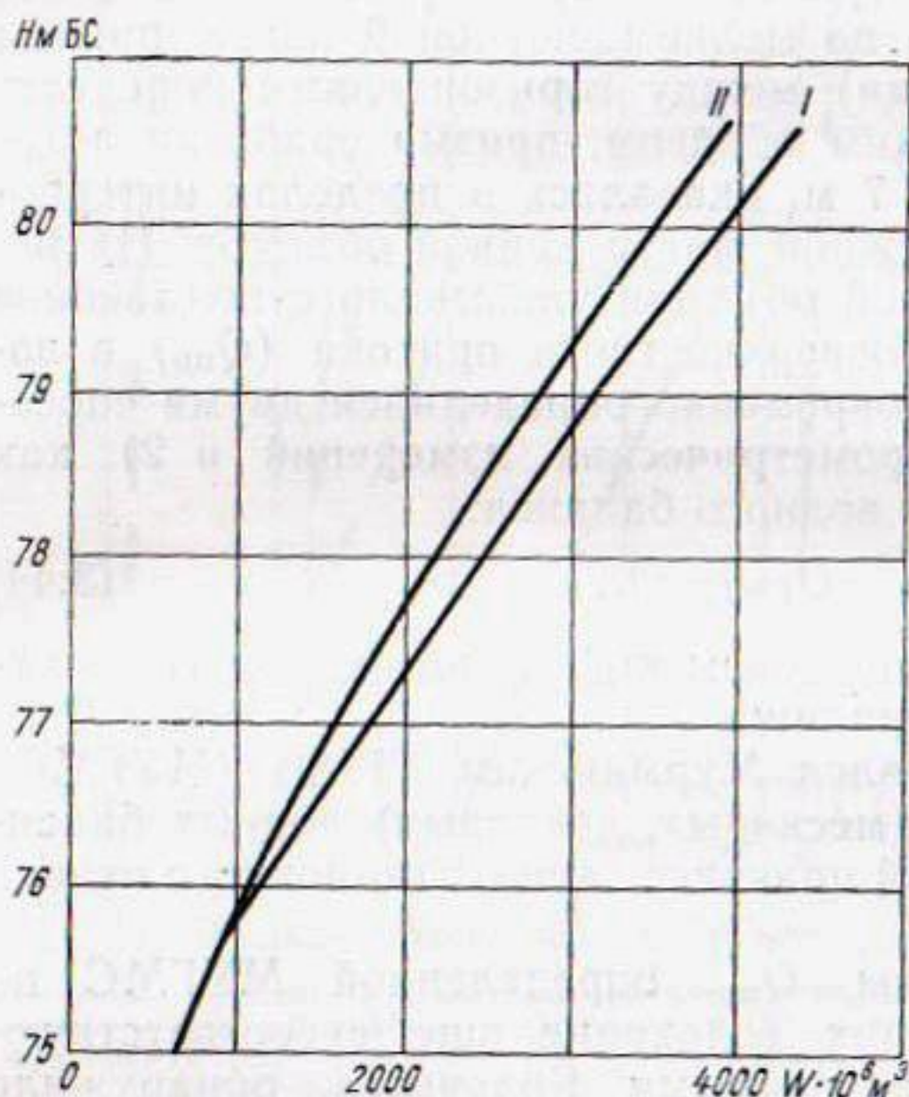
Рис. 25. Кривые объемов вдхр Верхнетуломского.
