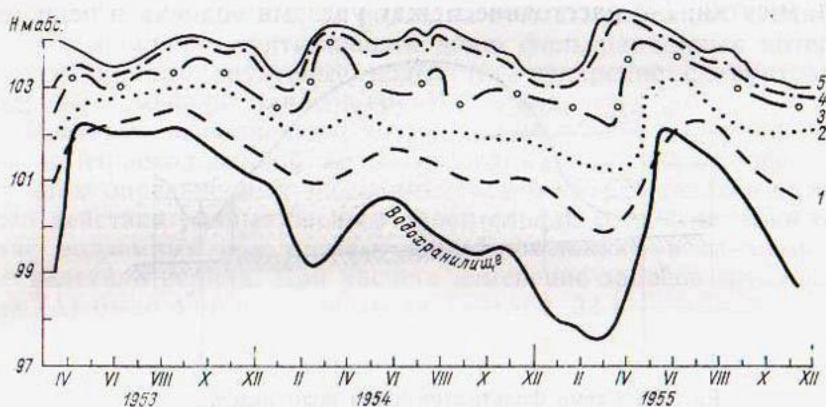
Рис. 21. Изменение уровня грунтовых вод в прибрежной зоне водхр Рыбинского.
