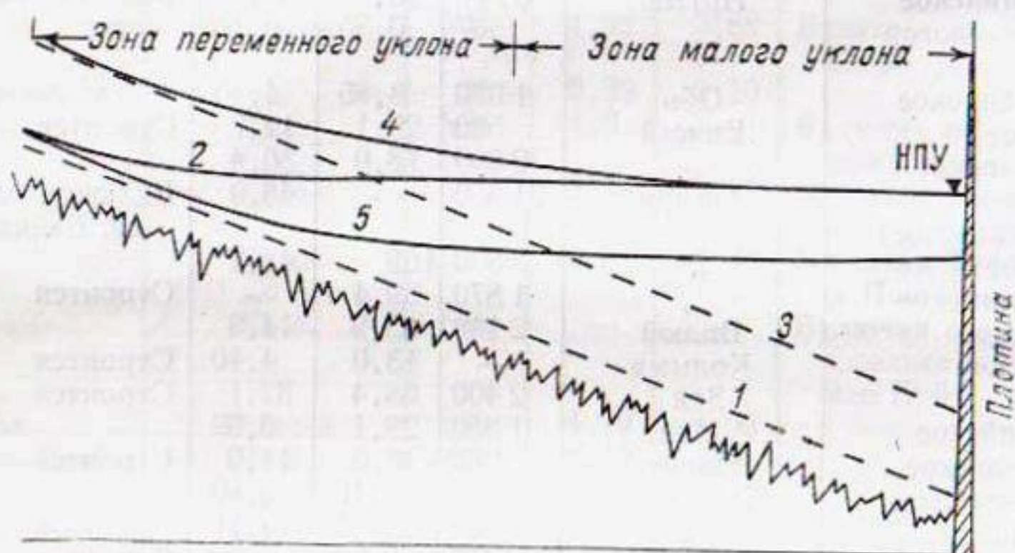
Рис. 2. Схема продольного профиля водохранилища при разном наполнении.
