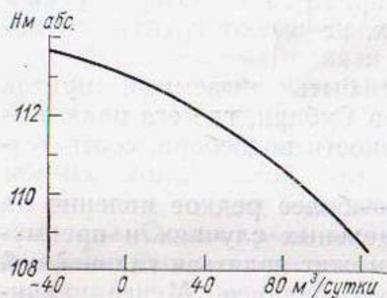
Рис. 19. Зависимость расходов воды, аккумулярованной в грунтах берегов, от уровня водохранилища Новосибирское.
