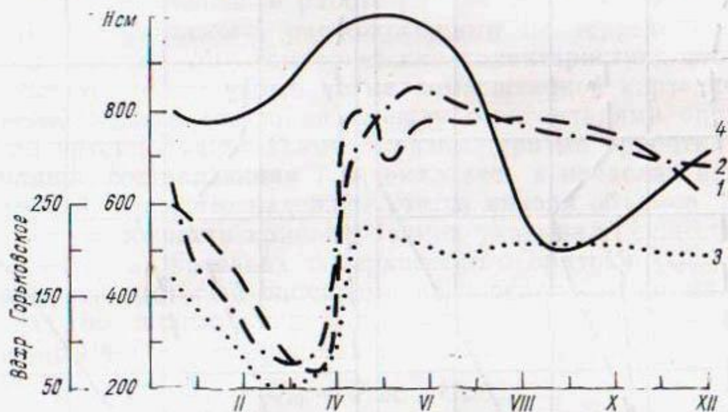
Рис. 23. Годовой ход уровня водохранилищ.
