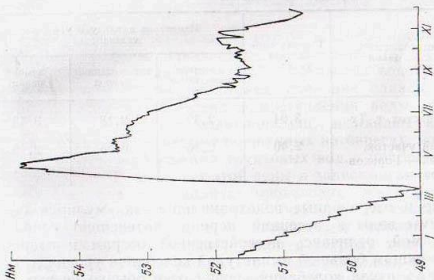
Рис. 3. Ход уровня в зоне выклинивания подпора на изолированном водохранилище.
