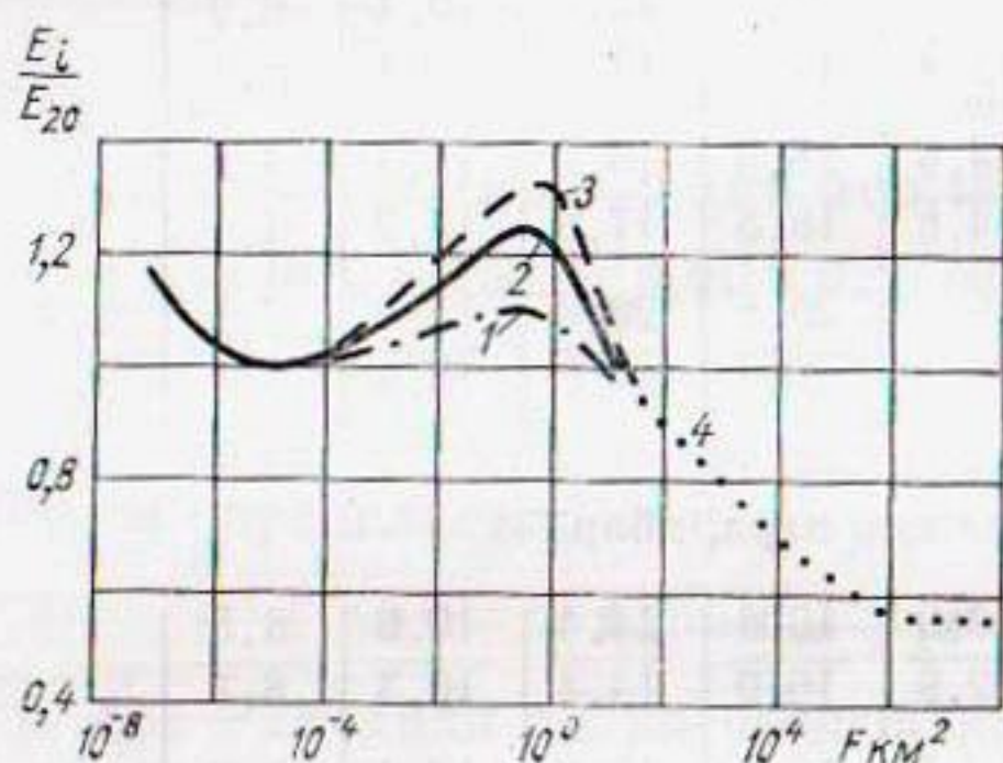
Рис. 14. Зависимость интенсивности испарения от площади водоема (по А. Р. Константинову).
