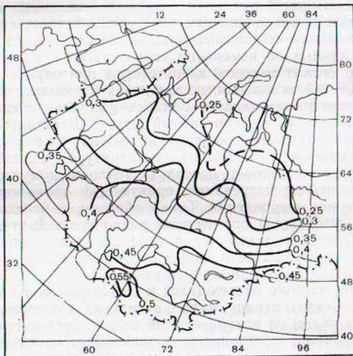
Рис. 17. Картограмма параметра b в уравнении \frac{EL}{B_{\Pi}} = 0,058u_{200} + b .
