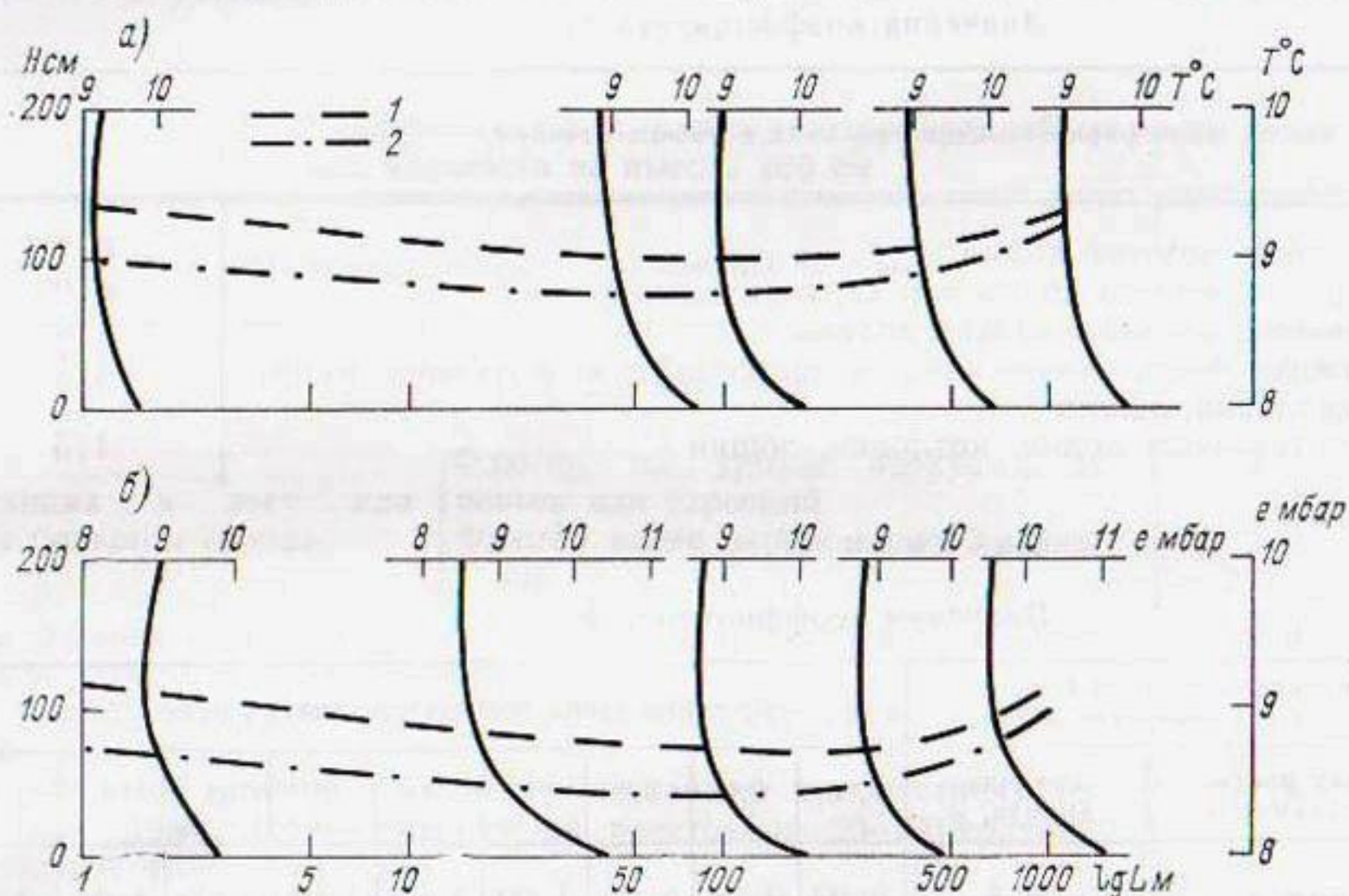
Рис. 13. Трансформация профилей температуры (а) и влажности (б) воздуха над водоемом.
