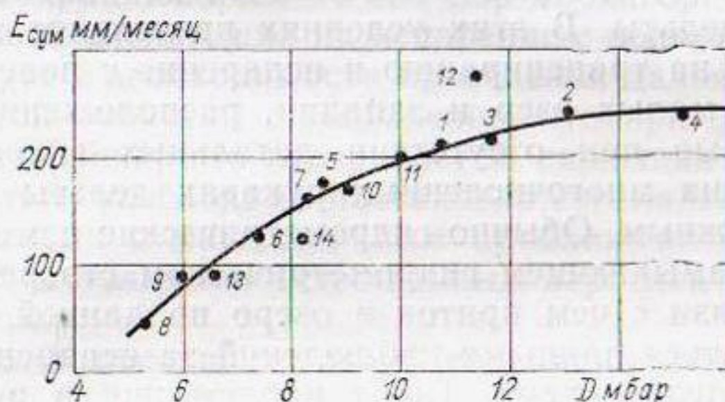
Рис. 18. Зависимость суммарного испарения (транспирация плюс испарение с воды между растениями) от дефицита влажности воздуха (по Т. М. Гельбух).
