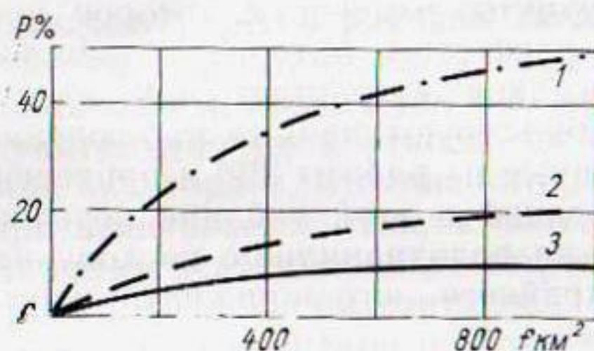
Рис. 11. Зависимость точности определения слоя осадков на площади ( f ), приходящейся на один осадкомер.
