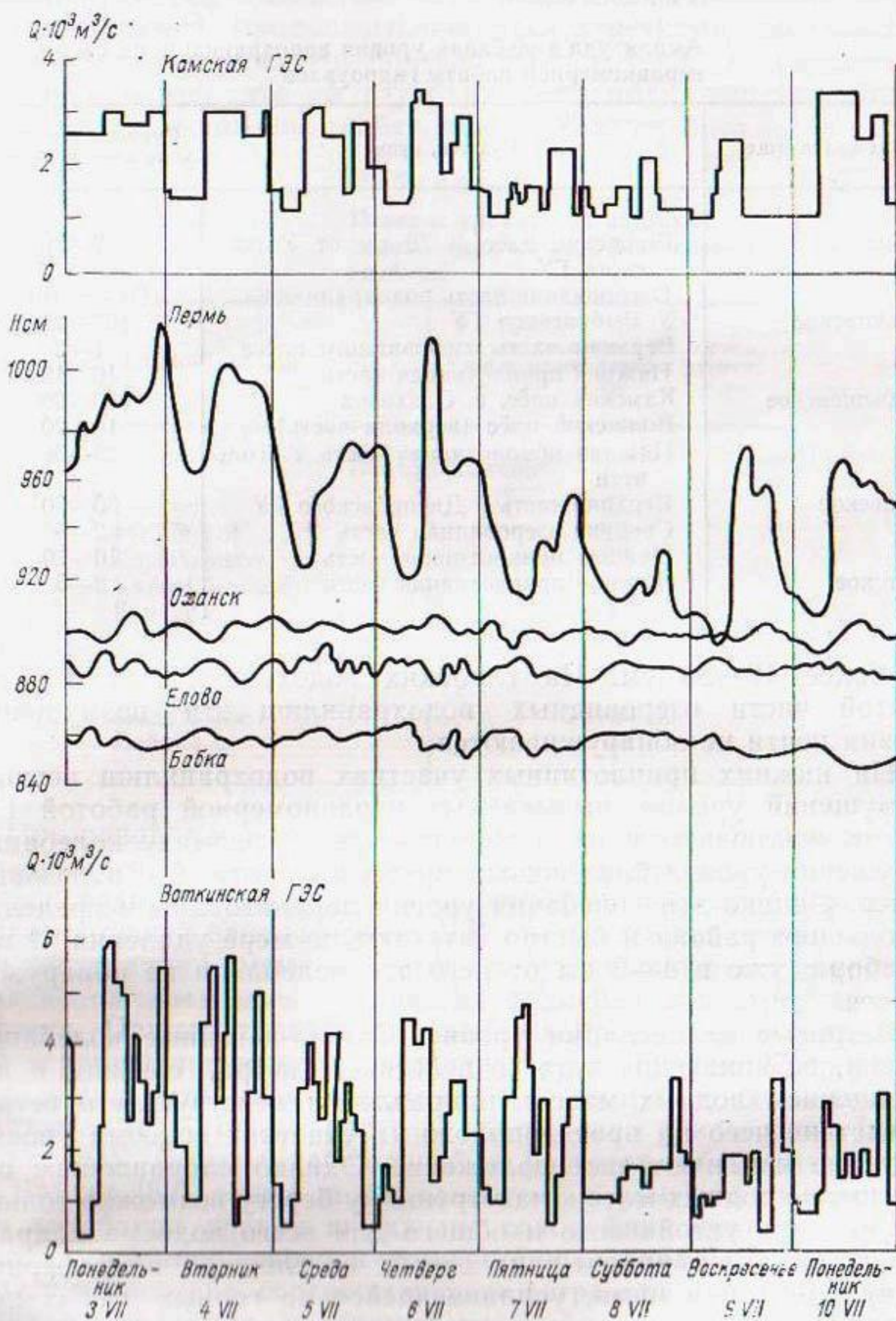
Рис. 26. Совмещенный график хода уровня по водпостам вдхр Воткинского и расходов воды через Камскую и Воткинскую ГЭС 3—10/VII 1972 г.
