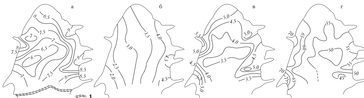
Рис. 32. Распределение слоя стаявшего снега W (а), радиационного баланса (б), турбулентной составляющей ( P+LE ) (в) и отношения (P+LE)/rW (г) на леднике Обручева, 21–25 июля 1977 г. Параметры а, б, в приведены в г/см 2 ·сут. 1 — граница сезонного снега
