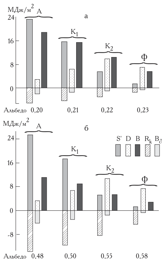
Рис. 10. Структура радиационного баланса за сутки для льда и фирна при различных типах погоды, ледник Марух. а — лед, б — фирн; S' , D , R_k — прямая, рассеянная и отраженная солнечная радиация, B_\lambda — баланс длинноволновой радиации, B — радиационный баланс. Обозначения типов погоды см. в тексте
