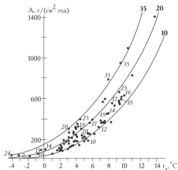
Рис. 41. Связь годовой абляции ледников и снежников A со средней летней температурой воздуха t_{\text{л}} и балансом коротковолновой радиации B_k за июнь — август (числа у точек и на изолиниях, ккал/см 2 ) (Ходаков, 1978)
