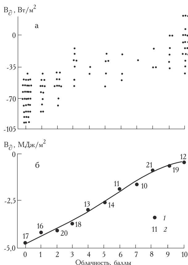
Рис. 9. Связь баланса длинноволновой радиации B_0 с нижней облачностью в отдельные часы (а) и за сутки (б) в фирновой зоне ледника Марух. 1 — среднее для данного балла, 2 — число случаев
