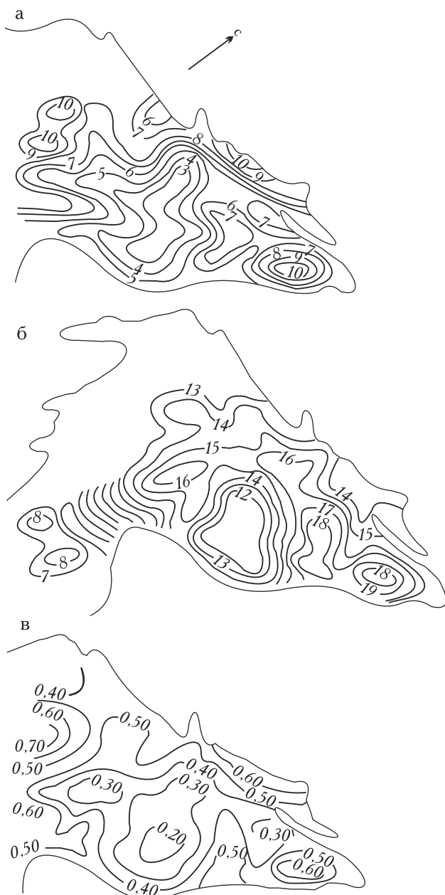
Рис. 31. Приток тепла вследствие турбулентного тепло- и влагообмена (P+LE) (а), затраты тепла на таяние rW (б) и отношение (P+LE)/rW (в) на леднике ИГАН за период с 23 июля по 3 сентября 1959 г., ккал/см 2 (Адаменко, 1968)
