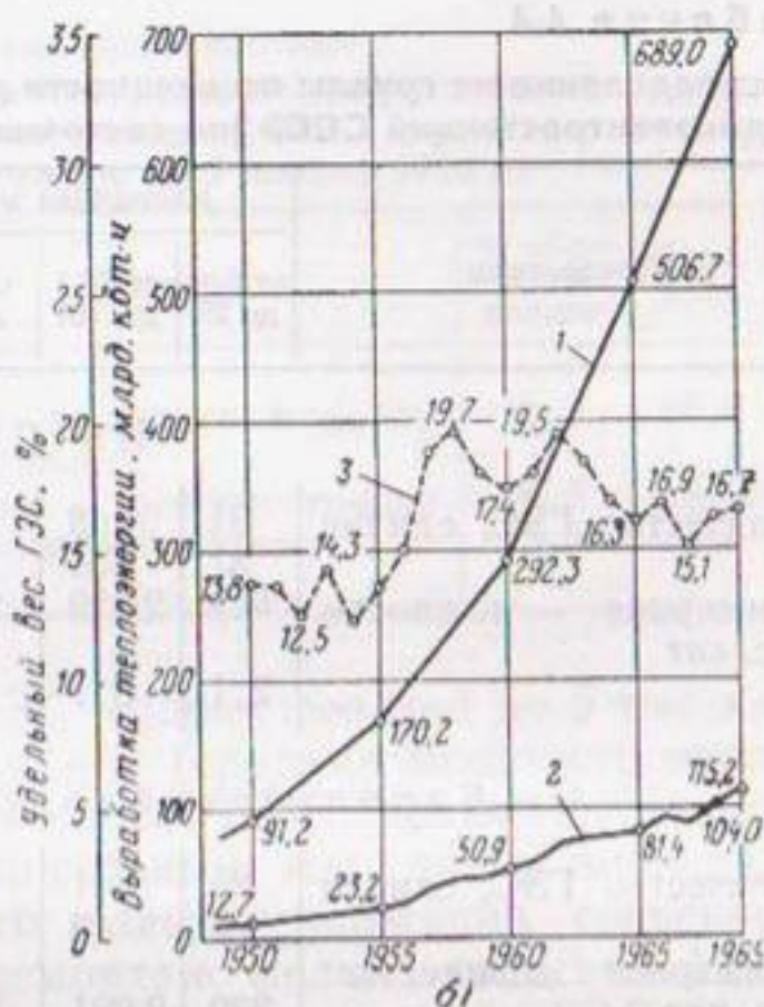
Рис. 4-1. Изменение удельного веса гидроэлектростанций СССР в мощности [а] и в выработке электроэнергии [б].
