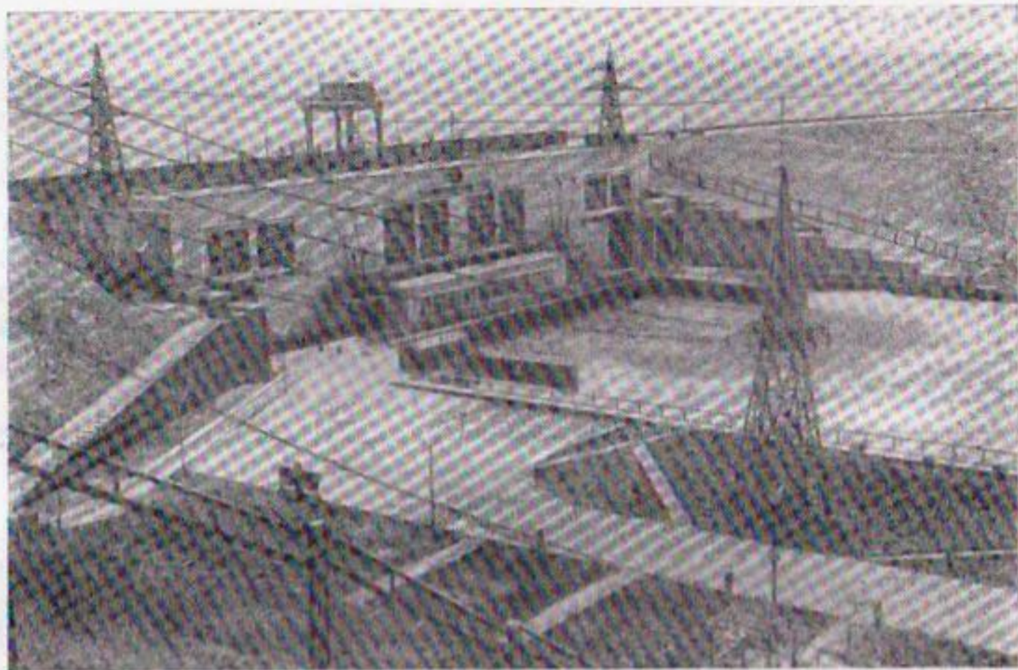
1-12. Чардаринская ГЭС на р. Сырдарье в Узбекистане.
