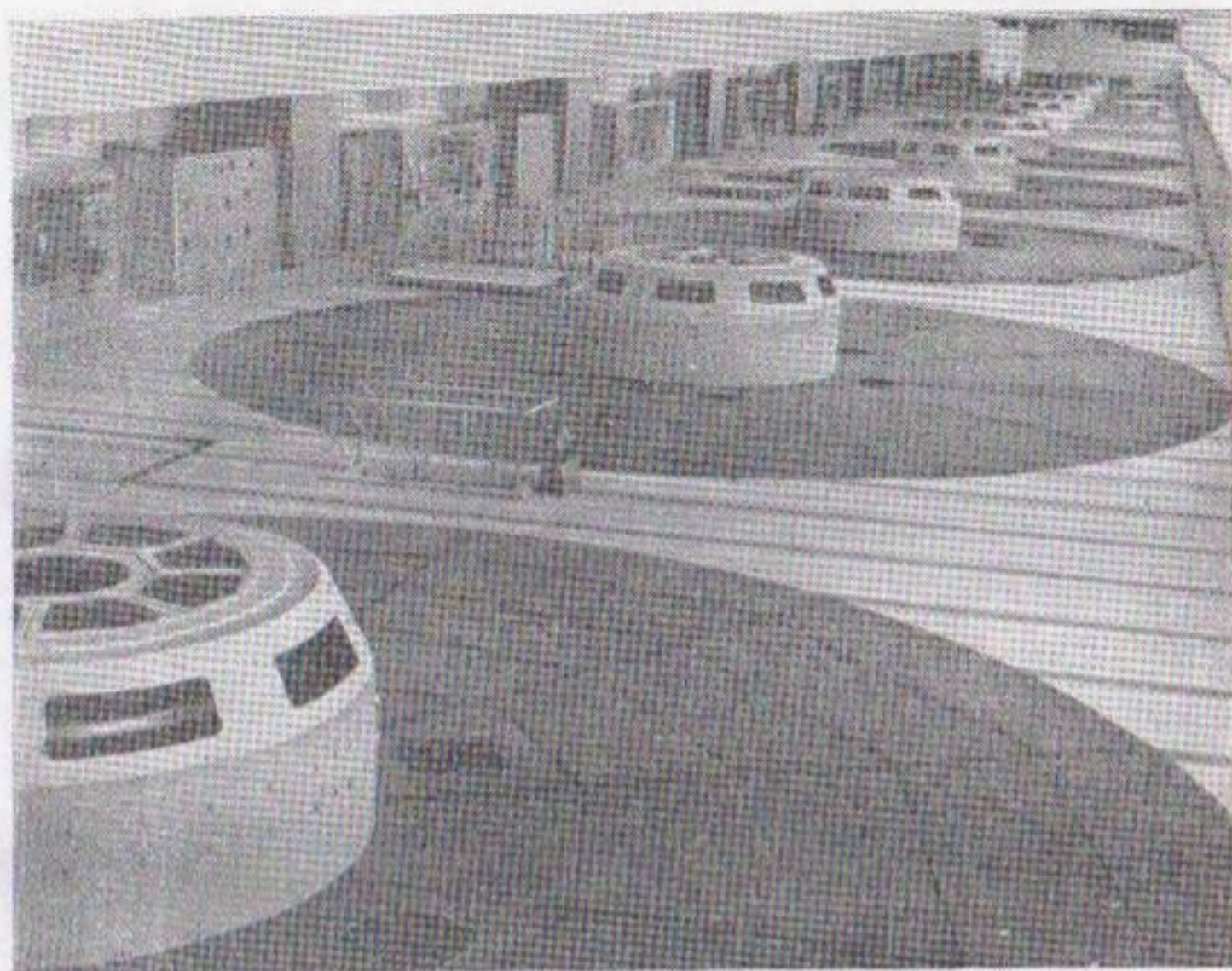
1-15. Машинный зал Плявиньской ГЭС имени В. И. Ленина.
