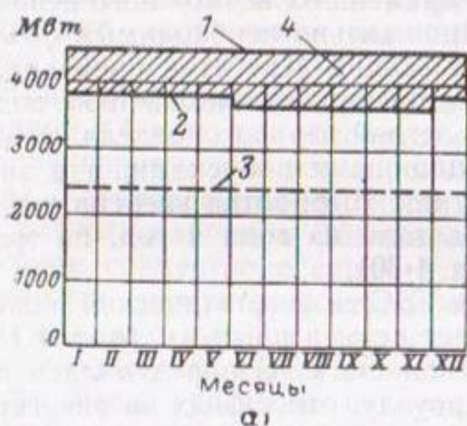
Рис. 4-13. Годовые режимы работы Братской ГЭС.
