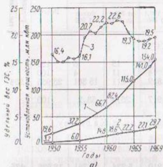
Рис. 4-1. Изменение удельного веса гидроэлектростанций СССР в мощности [а] и в выработке электроэнергии [б].
