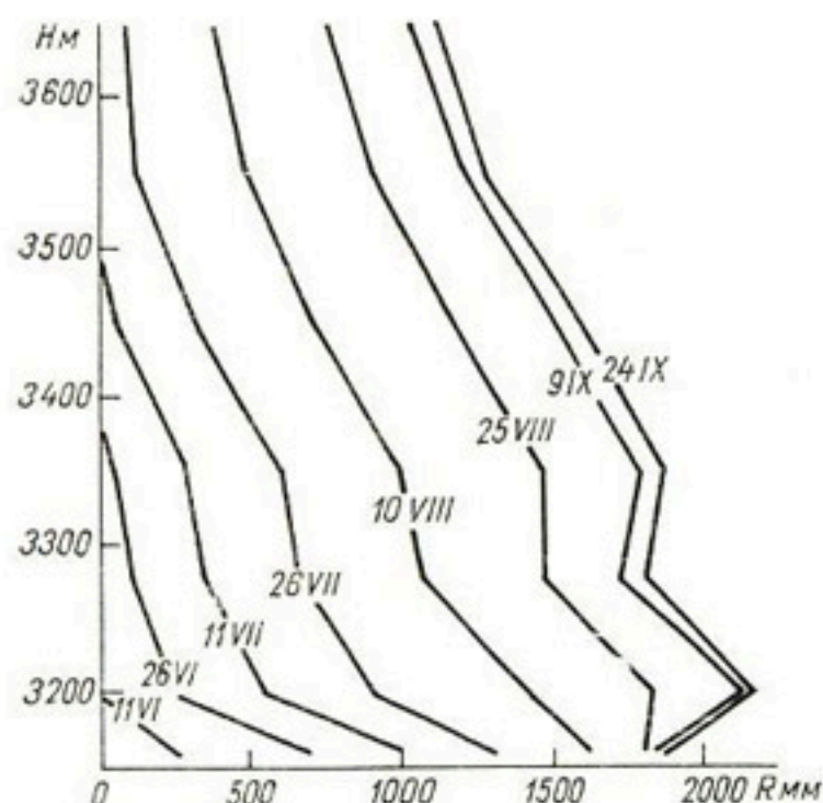
Рис. 17. Изменение слоя стока из снежно-фирновой толщи ледника Джанкуат с высотой в течение сезона абляции 1969 г.
