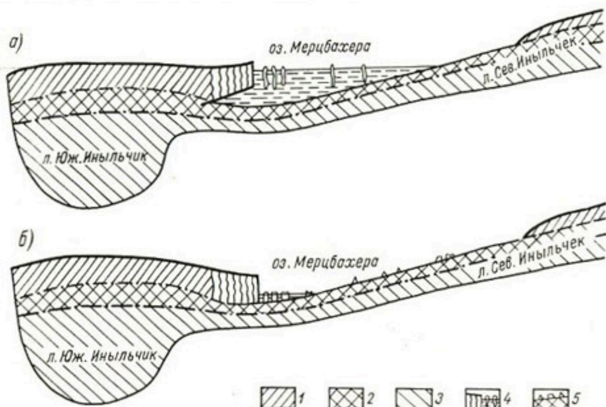
Рис. 62. Гипотетический схематический разрез через ледники Южный и Северный Иньльчек перед прорывом оз. Мерцбахера (а) и после прорыва (б).
