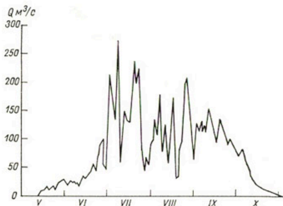
Рис. 45. Гидрограф р. Сельдары в истоке за 1959 г. (площадь бассейна 1380 \text{ км}^2 , площадь оледенения 72\% ) (по данным экспедиции ЛГУ).
