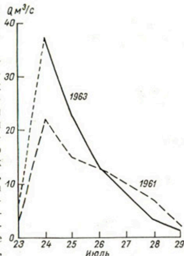
Рис. 59. Паводки, формирующиеся вследствие прорыва озера из-за перелива воды через ледяную плотину (оз. Битвин на о. Аксель Хейберг в Канаде, по данным Х. Маага [194]).
