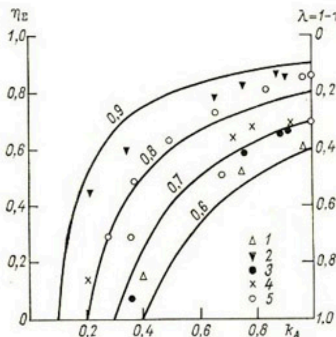
Рис. 13. Зависимость интегрального коэффициента стока \eta_{\Sigma} и коэффициента усвоения \lambda от относительной величины суммы талых и дождевых вод k_A .
