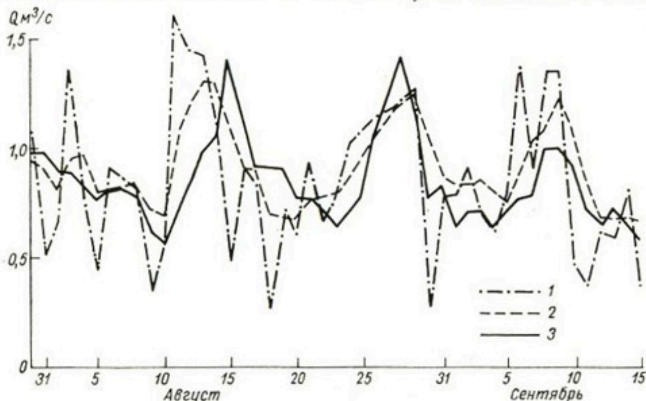
Рис. 51. График поступления воды на поверхность бассейна, наблюдавшийся и вычисленный гидрографы р. Кашкатор (у ледника Карабаткак) в 1959 г.
