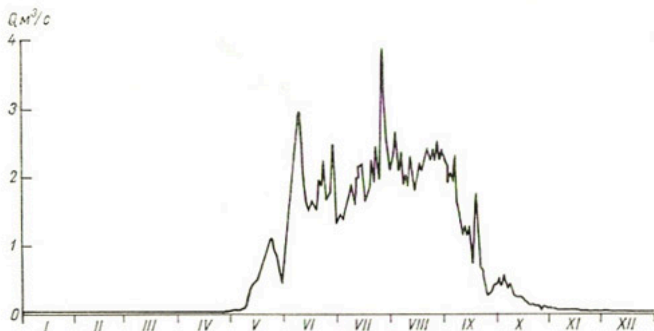
Рис. 43. Гидрограф р. Марухи в источке за 1969 г. (площадь бассейна 7,8 км 2 , площадь оледенения 42%).
