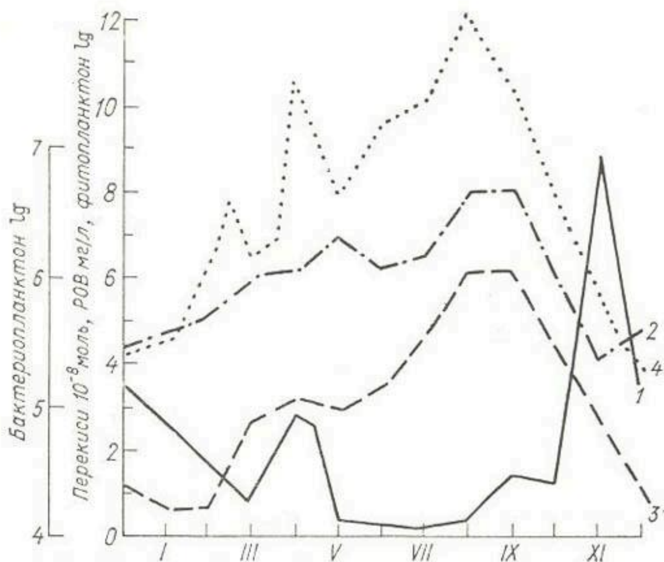
Рис. 1. Сезонная динамика численности водорослей и бактерий, концентраций POV и липоперекисей в пруду. 1 — перекиси, 2 — бактериопланктон, 3 — фитопланктон, 4 — POV.
