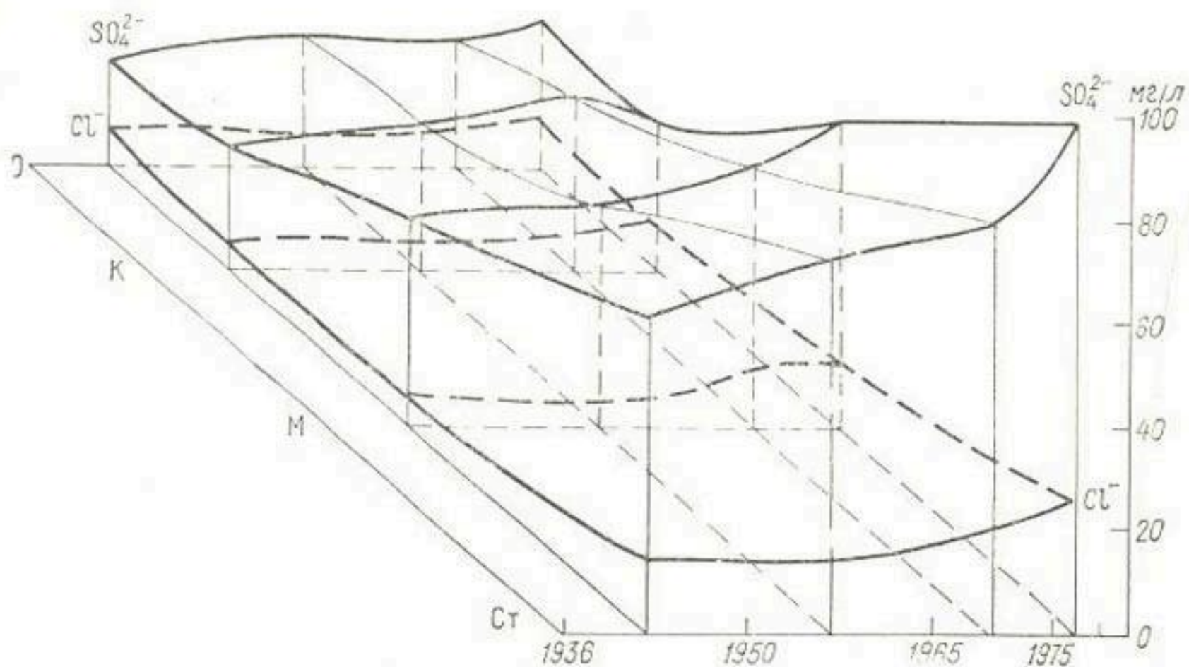
Рис. 1. Пространственно-временная блок-диаграмма изменения концентраций \text{SO}_4^{2-} и \text{Cl}^- по р. Терек.
