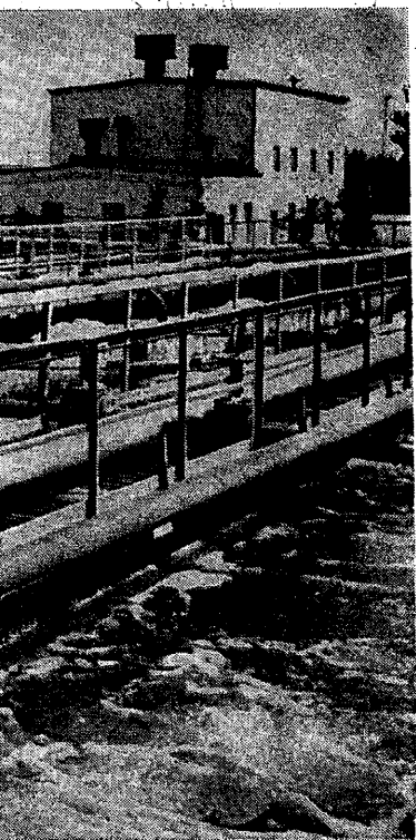
Рис. 8. Очистные соору- жения Северодонецко- го химического комби- ната. На переднем пла- не — усреднители.
