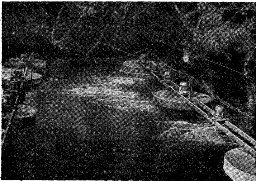
Рис. 9. Механическая аэрация речной воды в реке Невежис, Литовская ССР.
