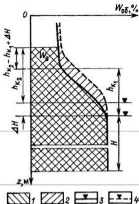
Рис. 14. Сопоставление нижних частей эиур влажности грунтов в зоне аэрации и в грунтовом потоке:
