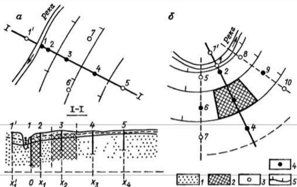
Рис. 31. Схемы расположения наблюдательных скважин в створах по потоку при одномерном в плане (а) и двухмерном (б) движении вод: 1—водопроницаемые и водоносные отложения; 2—расчетный элемент потока; 3—4—скважины (3—наблюдательная, 4—расчетная наблюдательная); 5—гидроизогины
