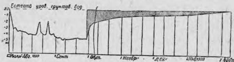
Рис. 200. Кривая депрессий и отбора воды в опытном колодце города Штендаль.
