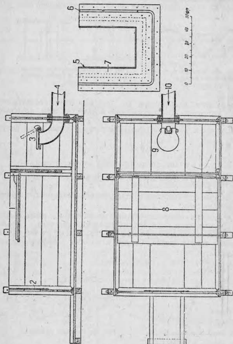
Рис. 45. Водослив Понселе.
