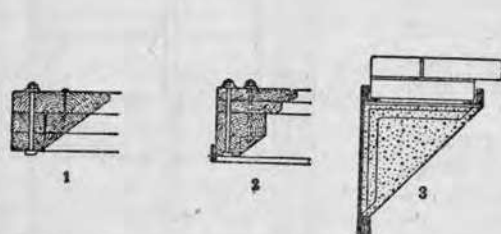
Рис. 244. Деревянные (1, 2) и железные (3) венцы колодцев.
