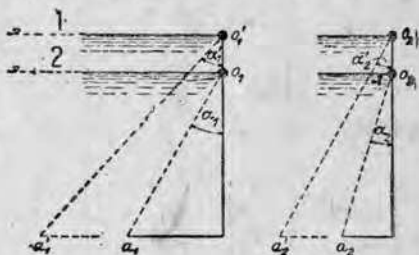
Рис. 310. Линии дебита колодца.
