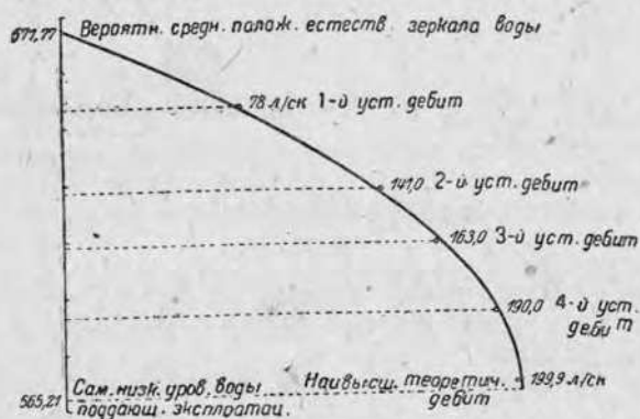
Рис. 132. Парабола дебита опытного колодца в Глейзентале близ Мюнхена (по А. Тиму).
