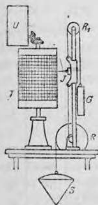
Рис. 49. Самопишущий футштог (по Будау).
