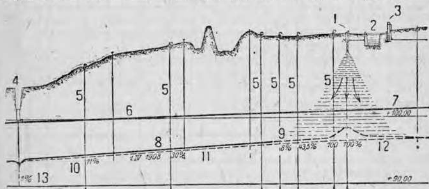
Рис. 320. Сооружение для образования грунтовой воды в городе Франкфурте-на-Майне (по Шельгзе).
