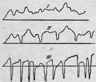
Рис. 63. Кривая хода уровня в неэксплуатируемых колодцах (I), в эксплуатируемых водонепроницаемых (II) и в эксплуатируемых слабоводопроницаемых колодцах (III).
