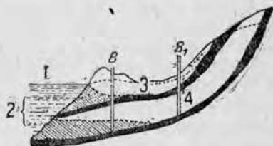
Рис. 184. Схема залегания водоносных пластов, содержащих пресную и соленую воду, если между ними имеется водонепроницаемый пласт (по д'Андримон).
