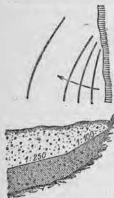
Рис. 91. Уменьшение падения грунтовой воды по направлению к центру потока грунтовой воды.
