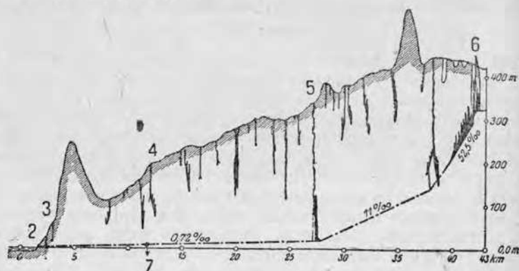
Рис. 157. Продольный разрез подземного течения реки Тимаво между гротом Сен-Калциан и Дуино (по Бегану).
