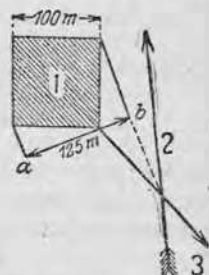
Рис. 140. Четырехугольный каптаж водопровода города Лютиха (по Дегинне).
