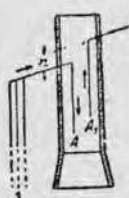
Рис. 294 и 295. Неправильное присоединение подъемного и всасывающего трубопровода.
