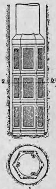
Рис. 271. Фильтр со стеклянными пластинками (по Путзейсу).
