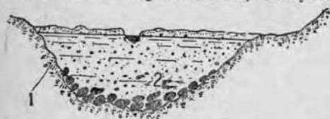
Рис. 21. Разрез водоносного пласта с выстланной камнем постелью.
