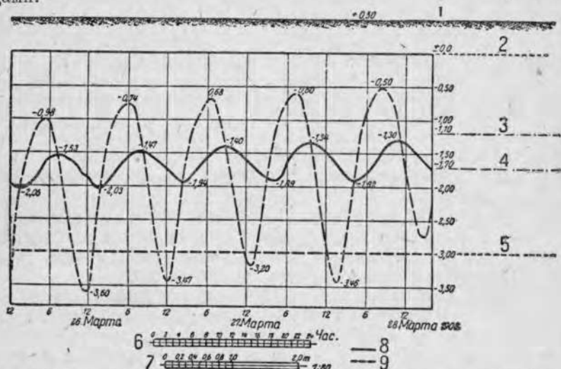
Рис. 71. Колебания зеркала грунтовой воды близ Эмденских морских плезов.
