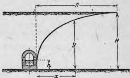
Рис. 130. Инфильтрационная штольня.
