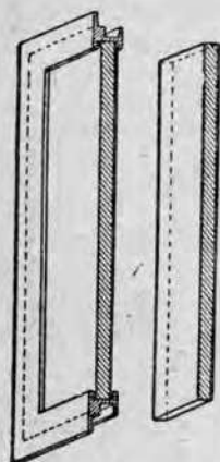
Рис. 272. Стекло- вые пластинки для каптажа воды в мел- ких песках (по Пут- зейсу).
