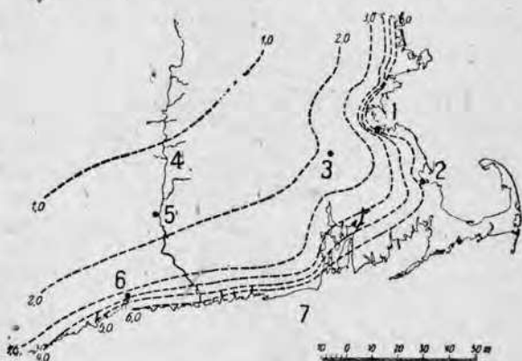
Рис. 180. Линии одинакового содержания хлора (изохалы) (миллионные доли) в штате Нью-Йорк (по Джек-сону).
