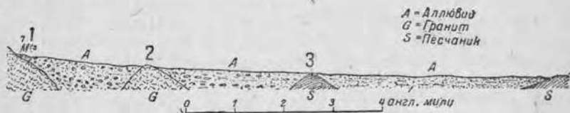
Рис. 33. Распадение сплошного потока грунтовой воды на отдельные потоки (по Менденгалю).
