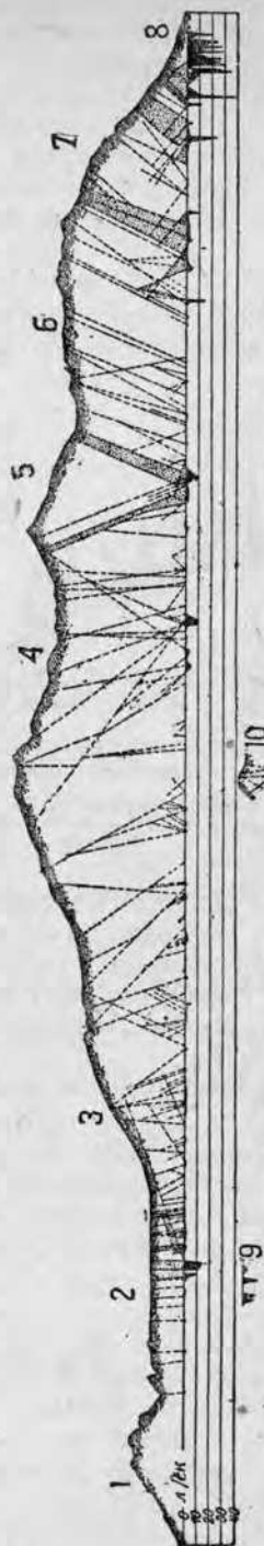
Рис. 150. Трещины, водною которых питается С.-Готтардский тоннель (по Штапфу).
