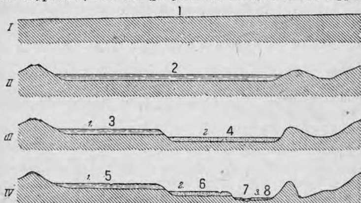
Рис. 36. Последовательное развитие террас Гаронны близ Тулузы (по Мандоулю) 1 — первоначальная поверхность земли; 2 — ложе потока глетчерных вод; 3 — терраса; 4 — терраса 5 — терраса; 6 — терраса; 7 — Гаронна; 8 — терраса.
