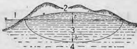
Рис. 182. Пресная вода дюн, плавающая на соленой воде (по Герцбергу).
