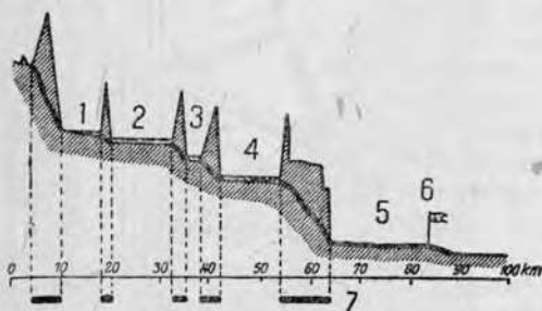
Рис. 151. Продольный разрез реки Лайбаха с временными озерами по Шенкелю.
