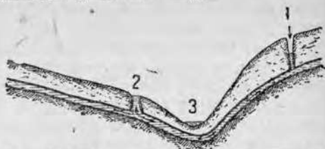
Рис. 164. Пересечение долины реки Ванны подземным водотоком (по Динерту).
