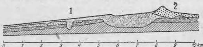
Рис. 81. Профиль долины Изера между Полахом и Шефтларном, изображающий переход морены (2) в флювиогляциальные отложения (по Пенку).
