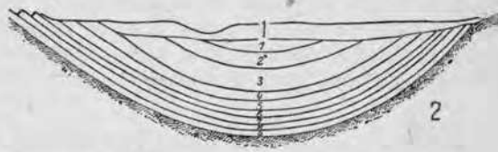
Рис. 30. Разрез артезианского бассейна в Вайоминге (по Найту).
