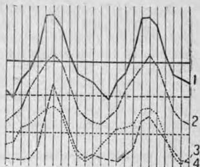
Рис. 69. Двухгодовые периоды осадков, дефицита насыщения и уровня грунтовой воды в Мюнхене (по Сойка).
