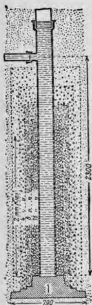
Рис. 270. Трубчатый колодец с засышкой из гравия в мелких песках первоначального каптажа города Нюрнберга (по Тиму).
