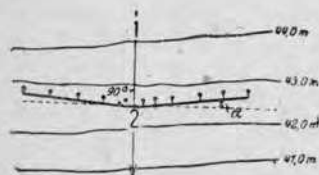
Рис. 203. Схематическое расположение каптажа с двумя отводами, отклоняющегося вверх по течению.
