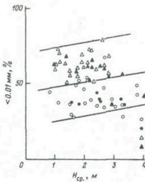
Рис.16. Связь среднего содержания частиц < 0,01 мм в донных отложениях со средней глубиной прудов Курской области (1), междуречья Хопер-Медведица (2), Азово-Кубанской равнины (3) и Ставропольского плато (4).
