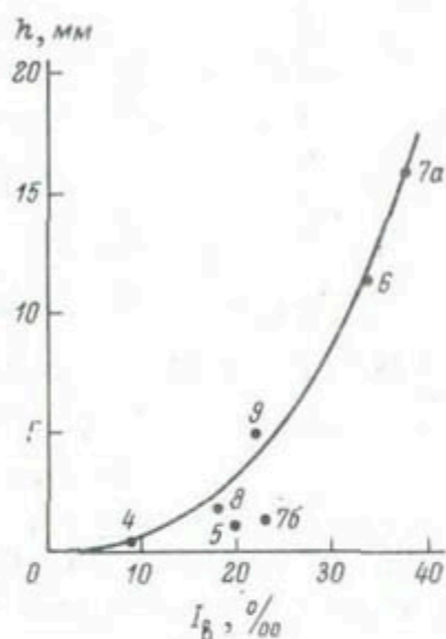
Рис.9. Связь среднего годового (1973–1976 гг.) склонового стока с частным водосбора прудов на б.Каракубанской с уклоном водосбора.
