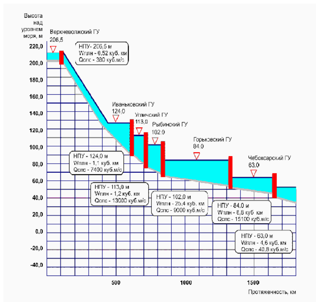
Рис.1. Схема продольного профиля верхнего участка реки Волга.
