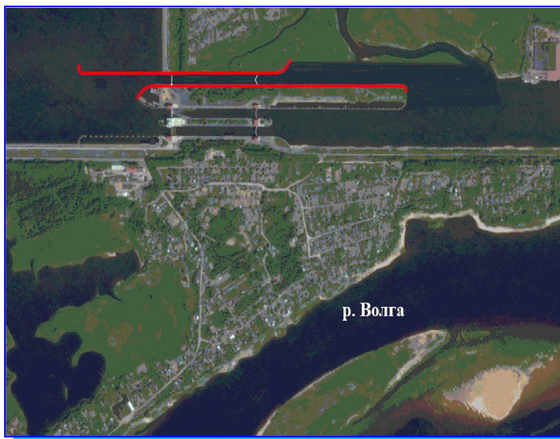
Рис. 3. Схема расположения третьей нитки Городецкого шлюза.
