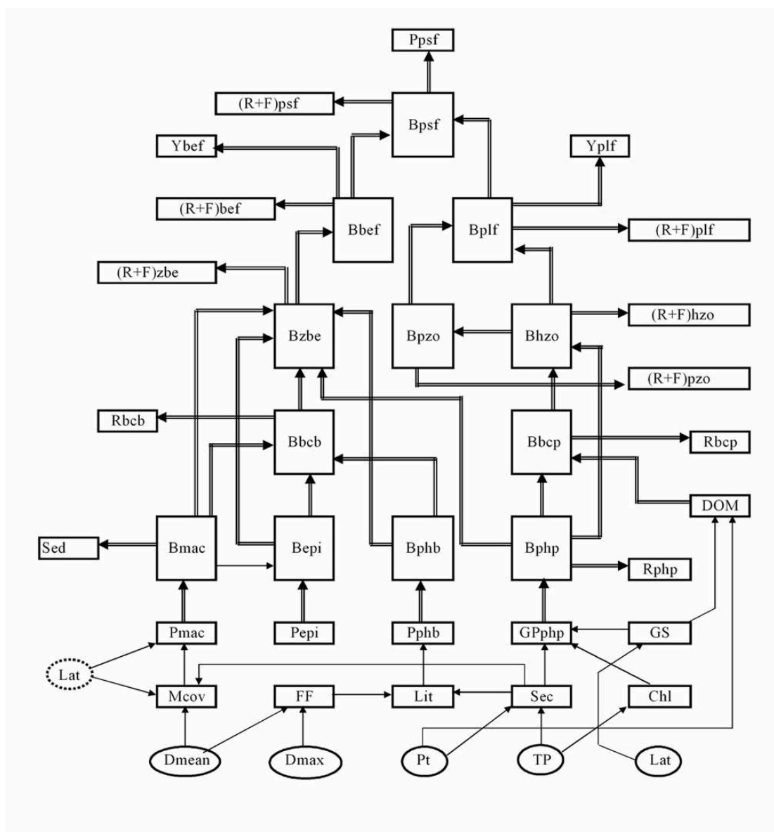
Рисунок 1 - Схема модели для прогнозирования биомассы и потоков энергии для ключевых групп автотрофных и гетеротрофных организмов. Объяснение в тексте.
