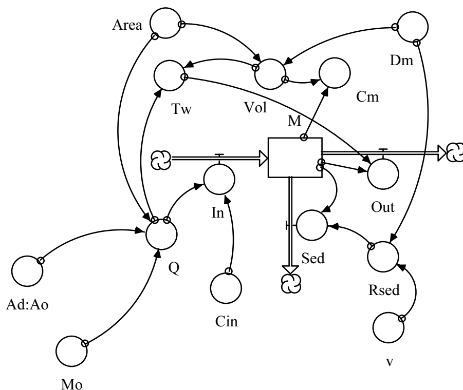
Рисунок 2 - Масс-балансовая модель для прогнозирования концентрации фосфора и цветности воды как показателя содержания гуминовых веществ. M – содержание вещества в объеме воды, In – приток вещества, Q – приток воды, Sed – седиментация вещества, Out – сток вещества, Rsed – скорость седиментации, Tw – время водообмена, Vol – объем воды, Cm – концентрация вещества в воде, Cin – концентрация вещества в притоке, Ad – площадь водосбора, Mo – модуль стока, v – линейная скорость седиментации вещества, Dm – средняя глубина водоема, Area – площадь зеркала водоема.
