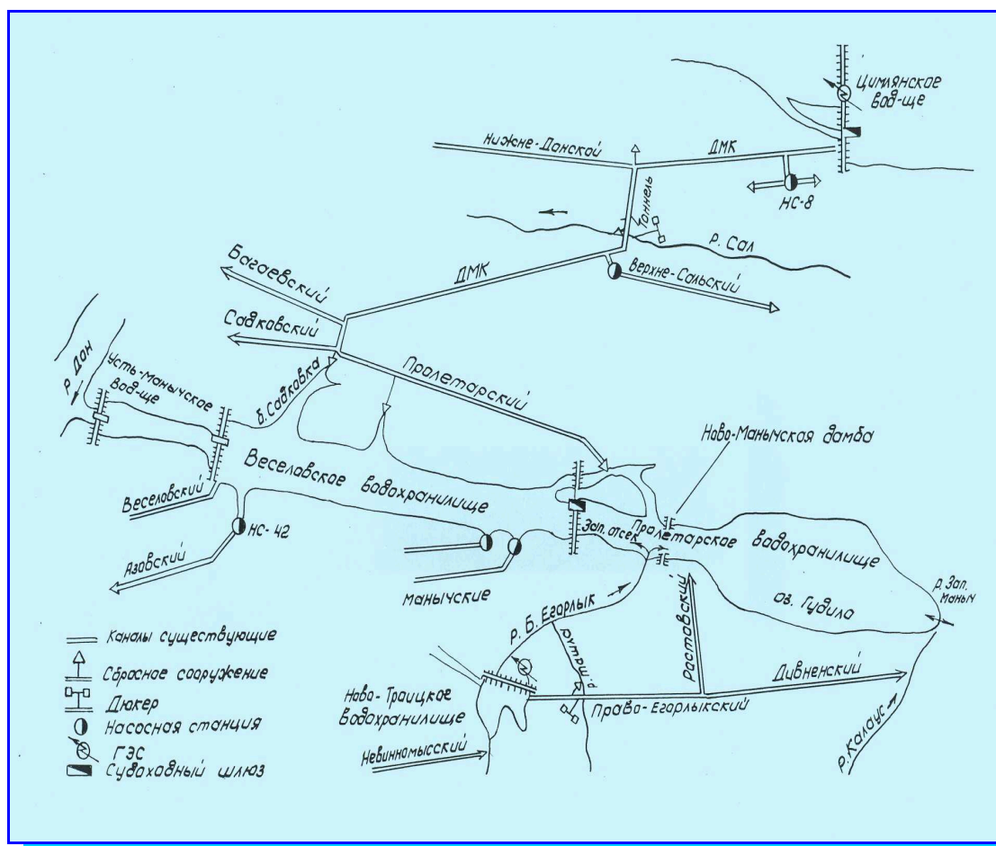
Рисунок 10- Схема Манычских водохранилищ
