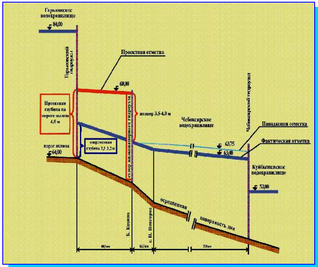
Рис. 2 Схема строительства низконапорного гидроузла, совмещенного с автодорогой.
