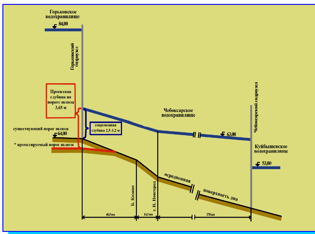
Рис.4 Схема строительства
