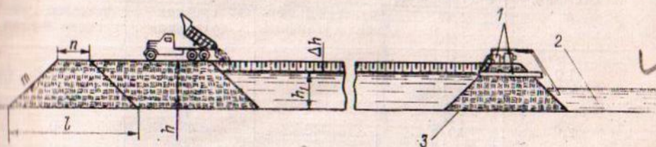
Рис. 3. Схема отсыпки грунтов в воду
