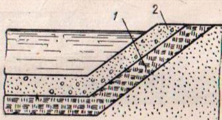
Рис. 10. Бассейн с глиняным экраном
