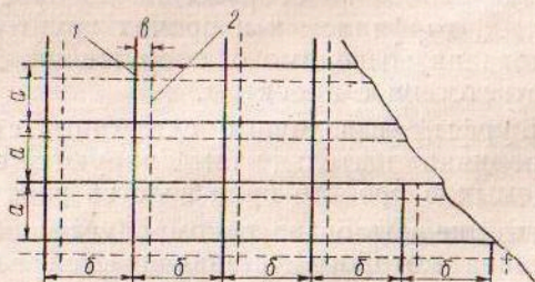
Рис. 1. Схема разбивки основания укладки слоя на отдельные карты
