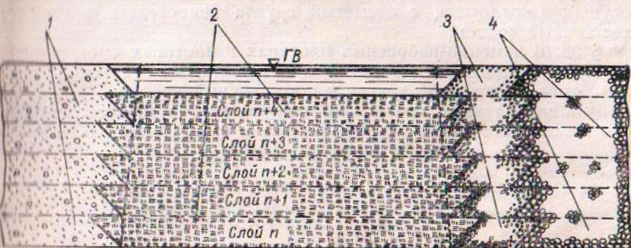
Рис. 15. Последовательность возведения глиняного ядра плотины 1 — упорная призма со стороны верхнего бьефа; 2 — слои глиняного ядра; 3 — слой обратного фильтра; 4 — слой каменной наброски.
