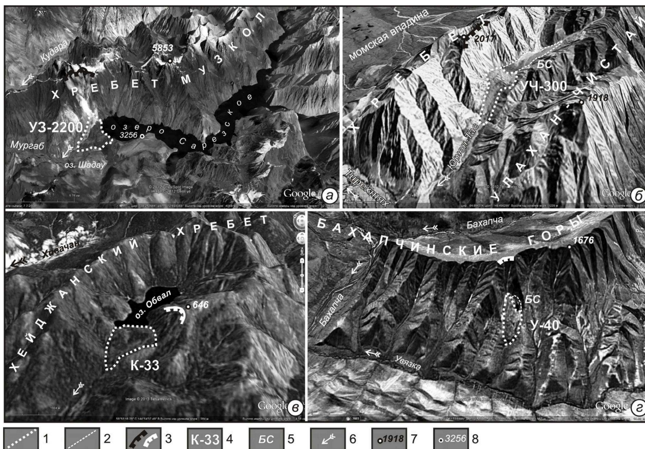
Рис. 1. Обвалные и оползневые плотины в горных долинах: а – на Памире, б – в горах Черского, в, г – в Северном Приохотье. 1 – контуры крупных (объемами свыше 1 млн м 3 ) скальных обвалов и оползней; 2 – контуры подпрудных бассейнов седиментации; 3 – бровки стенок срыва и ниш отрыва крупных обвалов и оползней; 4 – индексы обвалов и оползней, где буквы означают их названия: УЗ – Усойский завал, УЧ – Улахан-Чистай, К – Кумалкан, У – Увязка, а числа – их объемы в млн м 3 ; 5 – подпрудные бассейны седиментации; б – здесь и далее – направления поверхностного стока вод; 7 – здесь и далее – абсолютные отметки горных вершин в метрах; 8 – здесь и далее – абсолютные отметки уреза вод в метрах
