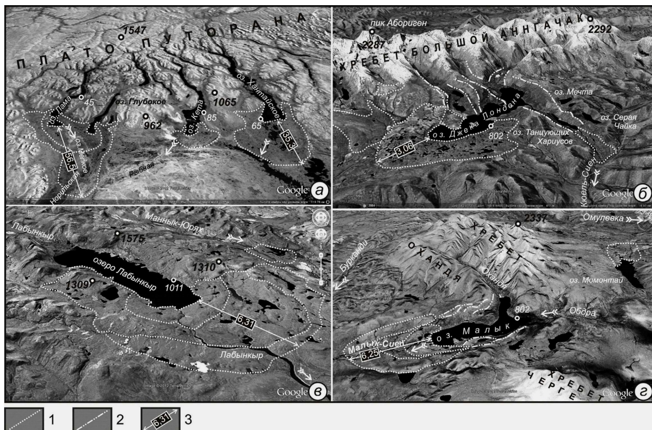
Рис. 5. Запруды горных долин реликтовыми моренами позднеледниковых ледников: а – на плато Пutorана; б, в – в горах Черского; в – в хр. Сунтар-Хаята. 1 – контуры конечно-моренных комплексов; 2 – хорошо выраженные в рельефе валы береговых морен; 3 – ширина конечно-моренных комплексов в километрах
