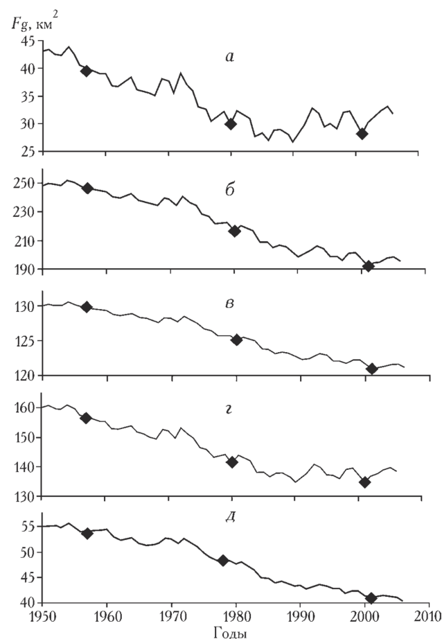
Рис. 1. Изменения площади оледенения F_g в бассейнах рек Шхимрудн (а), Сох (б), Исфар (в), Зеравшан (г), Ойгинг (д) за 1950—2006 гг.
