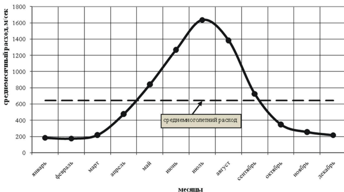
Рис. 3. Среднегодовой гидрограф р. Вахи.
