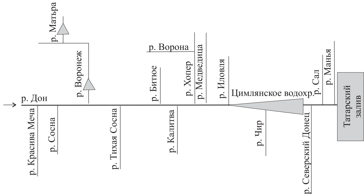
Рис. 4. Линейная расчетная схема реки Дон:
