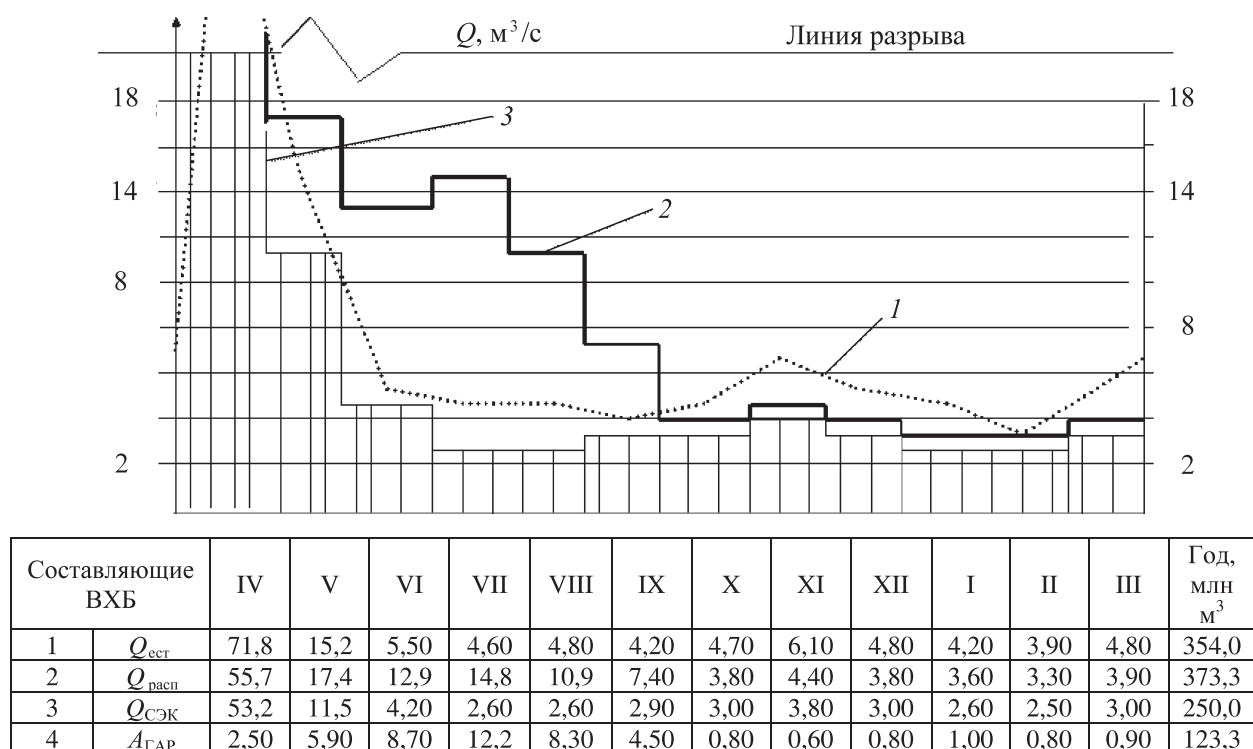
Рис. 5. Схема иллюстративного водохозяйственного баланса (к проектной перспективе 2005 года): Q_{\text{ест}} – естественный сток в створе гидроузла; Q_{\text{расп}} – зарегулированные располагаемые ВР с учетом дотации из внешнего речного бассейна; Q_{\text{СЭК}} – санитарно-экологический попуск; A_{\text{ГАР}} – гарантированное водопотребление брутто в расчетном сырье
