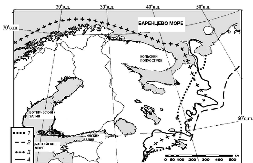
Рис. 2. Распространение оледенения в Европе в эпоху позднеледникового кризиса по данным реконструкций: 1 — А.А. Величко [2], 2 — Д.Д. Квасов [7], 3 — К.К. Марков [14], 4 — проект QUEEN [24]
