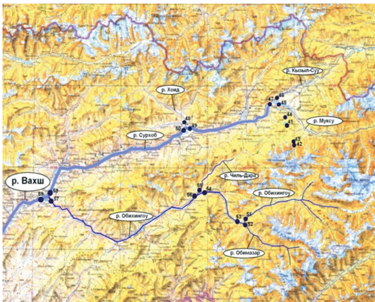
Рис.2 Схема формирования стока бассейна р. Вахи с основными местами опробования вод на изотопный состав урана
