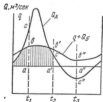
Рис. 86. Расчетная схема одностороннего компенсирующего водохранилища.
