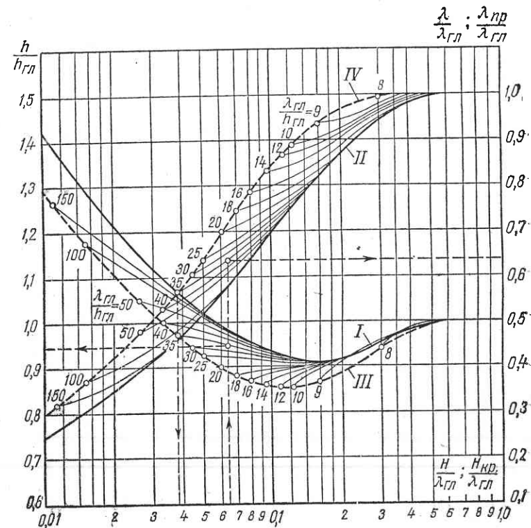
Рис. 62. График для определения относительной высоты волн \frac{h}{h_{гЛ}} (кривые I), относительной длины волн \frac{\lambda}{\lambda_{гЛ}} (кривые II), относительной критической глубины водоема \frac{H_{кр}}{\lambda_{гЛ}} .
