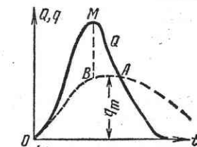
Рис. 89. Схема приближенного расчета донного водоспуска.
