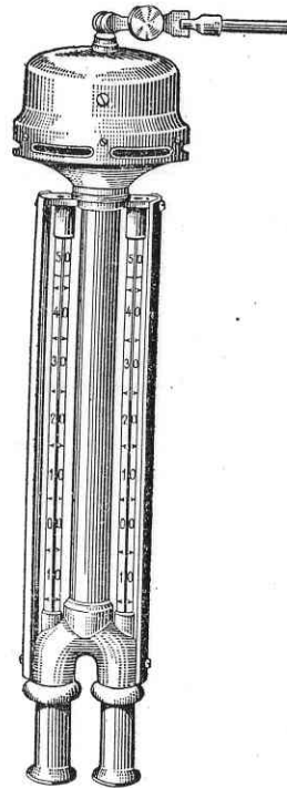
Рис. 35. Переносный психрометр Асмана.
