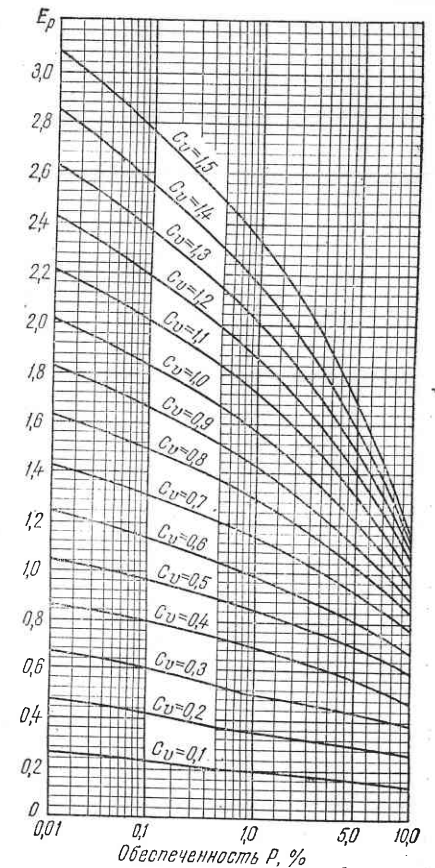
Рис. 27. Номограмма для определения E_p .
