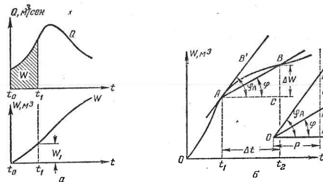
Рис. 72. Гидрограф стока и полная суммарная кривая (а); полная суммарная кривая и лучевой масштаб (б).
