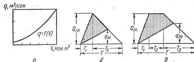
Рис. 87. К расчету емкости форсировки и схематизации паводка: а — график q = f(V) ; б — треугольник; в — трапеция.
