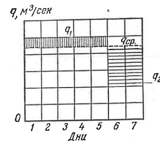
Рис. 56. Недельное регулирование стока.
