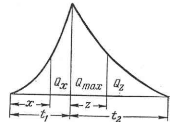
Рис. 31. Схема гидрографа паводка.
