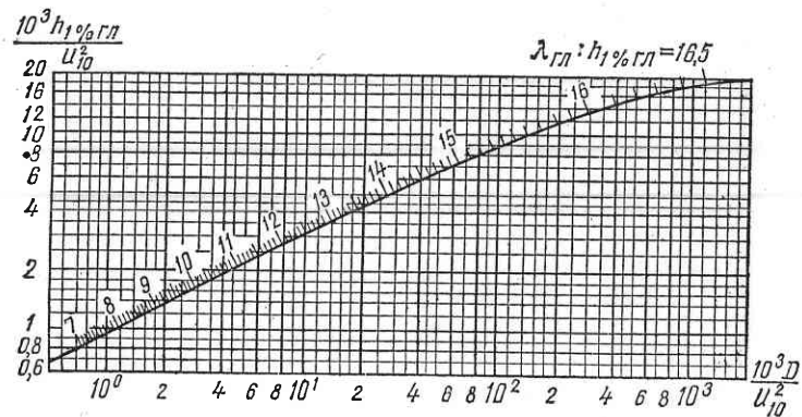
Рис. 61. График для определения параметров развитого волнения ( h_{1\%} , гЛ, м; \lambda_{гЛ} , м; u_{10} , м/сек).
