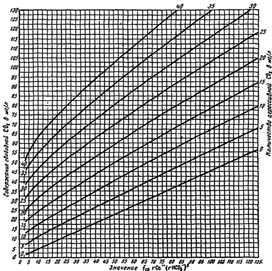
Рис. 2. График для вычисления агрессивной углекислоты при f_{\text{ср}} rCa^{++} (rHCO_3^-)^2 \leq 125
