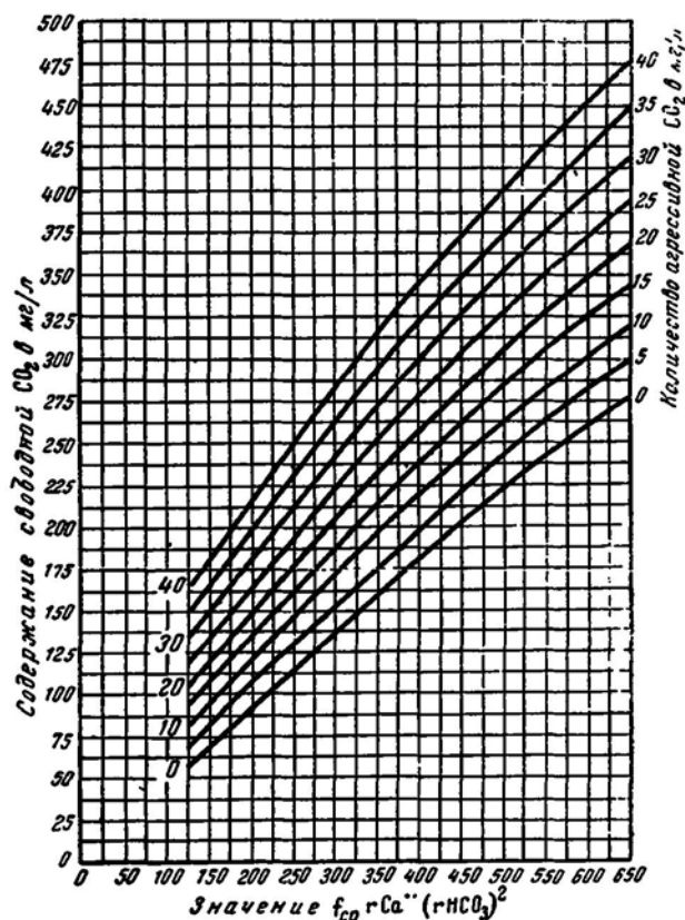
Рис. 3. График для вычисления агрессивной углекислоты при f_{cp} \cdot r\text{Ca}^{2+} \cdot (\text{rHCO}_3)^2 \geq 125
