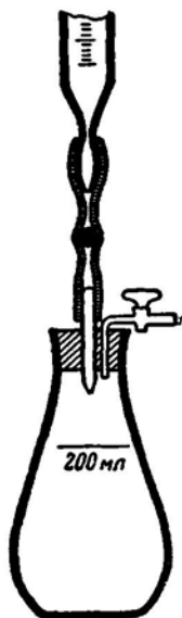
Рис. 8. Колба для определения свободной \text{CO}_2
