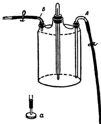
Рис. 4. Псевдобатометр конструкции Г. Ю. Верещагина
