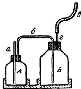
Рис. 5. Склянки для отбора проб воды
