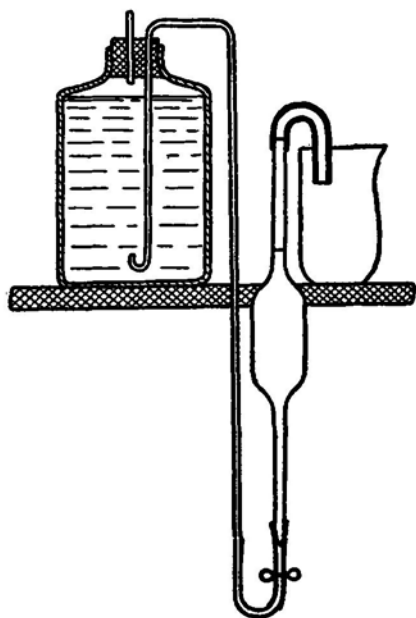
Рис. 9. Отбор пробы воды для определения свободной \text{CO}_2 с помощью обычной пипетки
