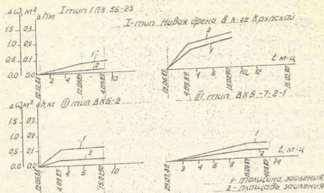
Рис 2. Интенсивность заиления дрена
