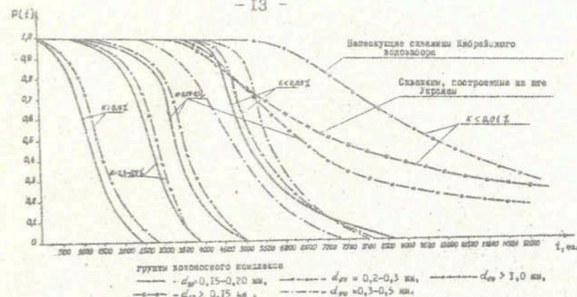
Рис.1. Вероятность безотказной работы электронасосов в водоносных грунтах при разной степени пескования скважин ВД
