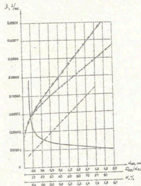
Рис.2. Зависимость интенсивности отказов электронасосов от литологии, состава гравийной обсыпки и пескования скважин в момент пуска. — d_{50} , — d_{50} < 0,20 , — d_{50} > 1,0 , — d_{50} = 0,3-0,5 мм.
