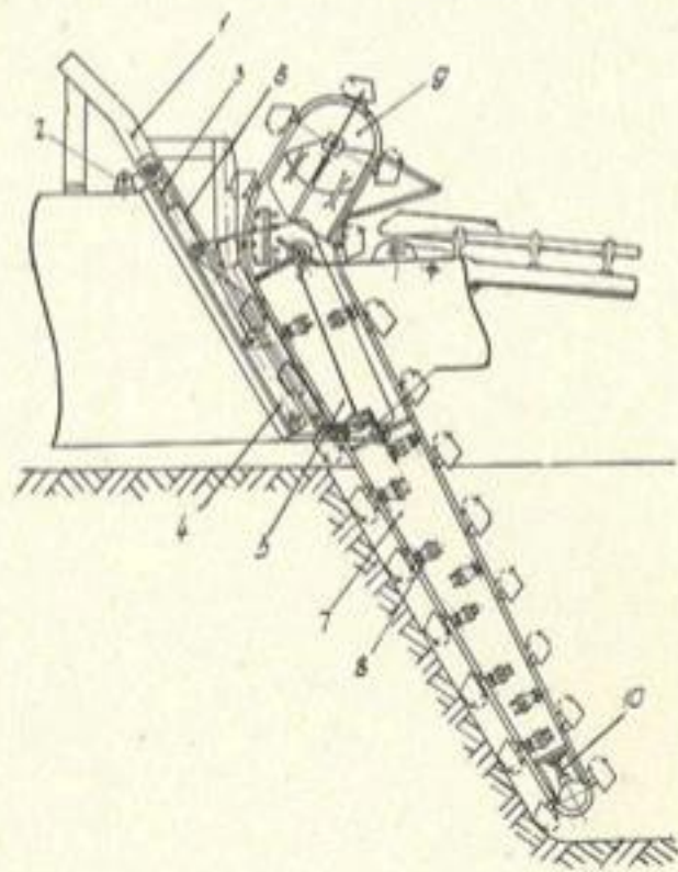
Рис. 58. Копаящий орган:
