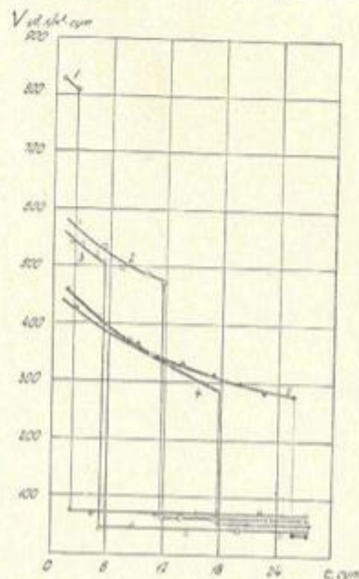
Рис. 39. Удельное подпоглощение из выемок до взрыва (кривые вверх) и после взрыва (прямые вниз)
