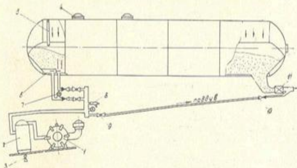
Рис. 53. Схема аэропневматической цистерны: 1 — ротационный компрессор; 2 — маслоотделитель; 3 — кран; 4 — люк; 5 — уравнительная труба; 6 — аэролоток; 7 — манометр; 8 — предохранительный клапан; 9 — муфтовый кран; 10 — обратный клапан; 11 — разгрузочное устройство
