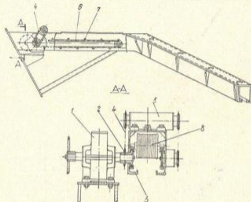
Рис. 63. Механизм автоматического выведения детонирующего шнура на поверхность грунта: 1 — редуктор; 2 — звездочки; 3 — цепь транспортера; 4 — цепи; 5 — синхронизирующий узел; 6 — цепь транспортера; 7 — ложемент; 8 — бобина с детонирующим узлом
