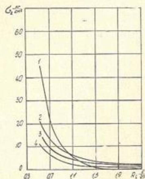
Рис. 2. Изменение радиальных напряжений от относительного расстояния при взрывании сосредоточенных камуфлетных зарядов гексогена (1), аммонита (2), тротила (3) и алюмотола (4).
