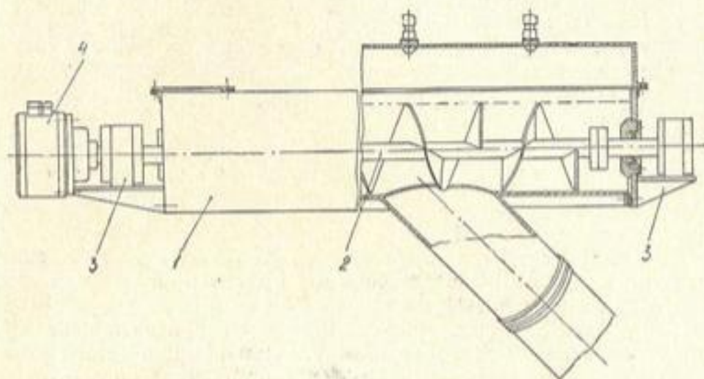
Рис. 60. Транспортер винтовой для подачи и смешивания аммиачной селитры и дизельного топлива:
