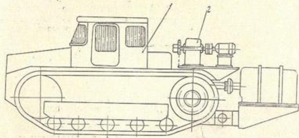
Рис. 54. Агрегат силовой: 1 — трактор ДЭТ-250М; 2 — ходоуменьшитель
