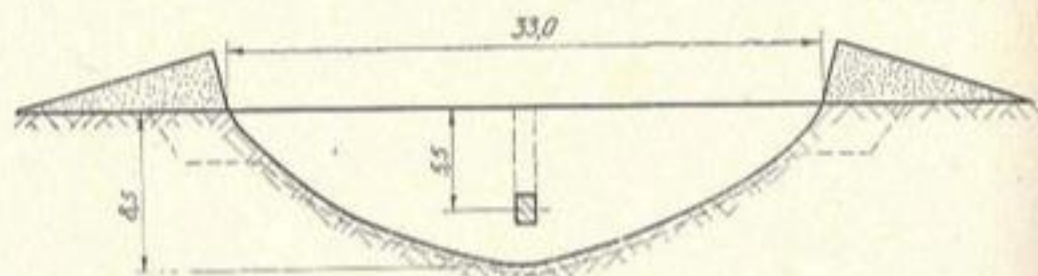
Рис. 28. Поперечный профиль выемки, образованной взрывом (пунктир — проектный профиль, сплошная линия — фактический профиль).
