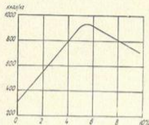
Рис. 3. Изменение теплоты взрыва (ккал/кг) игданита от содержания дизельного топлива (%).
