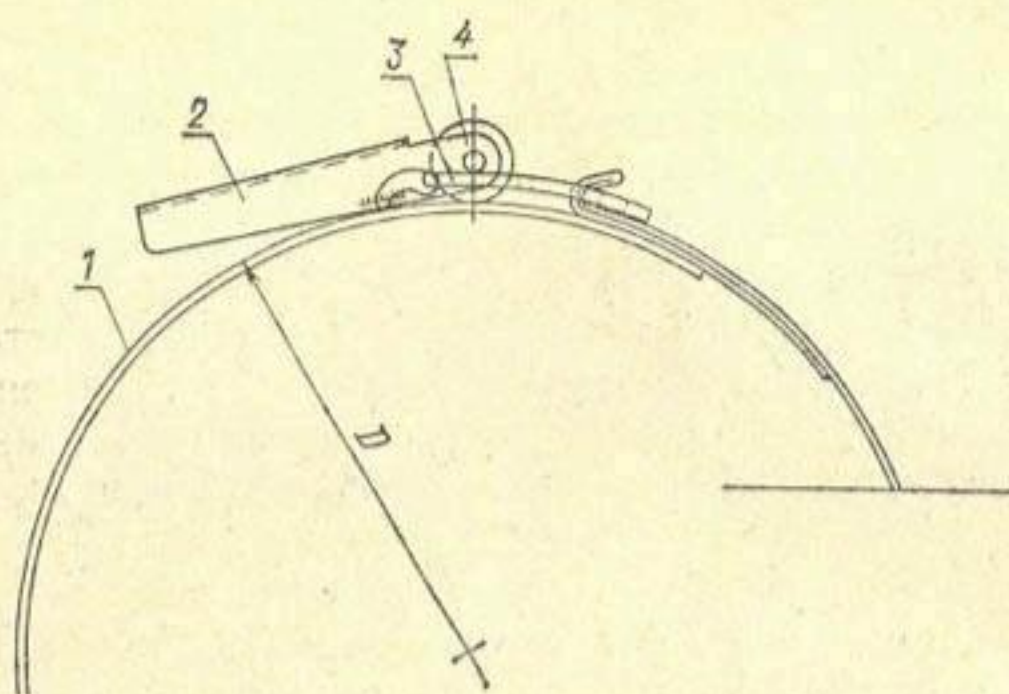
Рис. 31. Хомут с эксцентриковым замком: 1 — ленты хомута; 2 — рукоятка; 3 — планка; 4 — осевой ролик.
