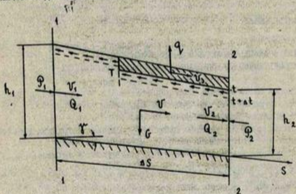
Расчетная схема неустановившегося движения.
