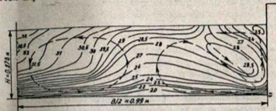
Рис. 3. Поперечное сечение русла с изотактами скорости течения и поперечные размеры вихрей, полученные в опыте № 3 первой серии.
