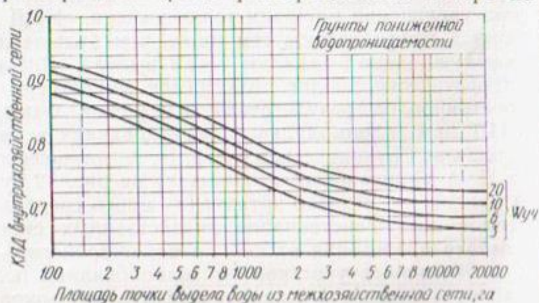
Рис. 14. Нормативные значения КПД хозяйственной сети в зависимости от площади точки выдела и средней площади поливного участка при грунтах пониженной водопроницаемости.
