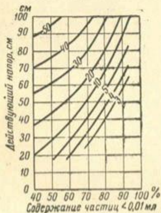
Рис. 40. Фильтрационный отток с затопленного рисового поля (в л/сек на 1 км картона) в зависимости от действующего напора и механического состава грунта.
