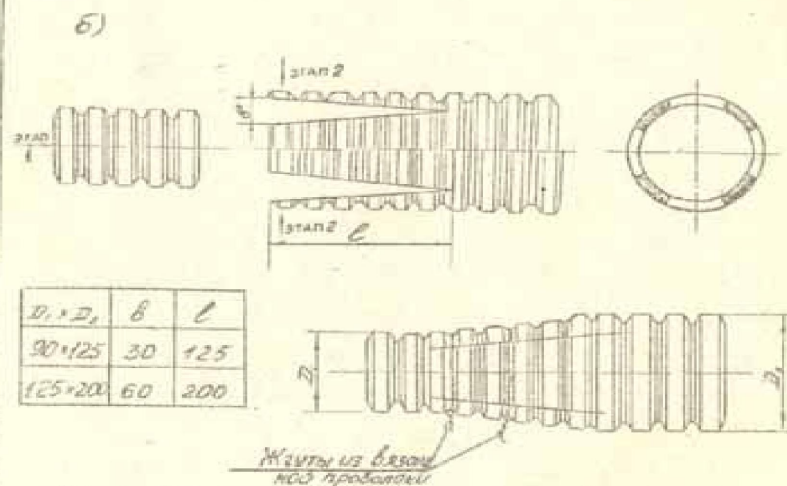
Рис.2-б. Схема соединения гофрированных труб, разных по диаметру Этап 1 - вдвижение меньшей трубы в большую Этап 2 - обвязка большей трубы по меньшей с помощью жгутов
