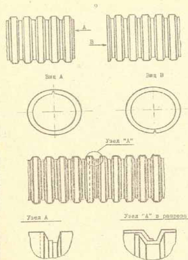
Рис. 3 Соединение плоскостных гофрированных труб, одинаковых по диаметру
