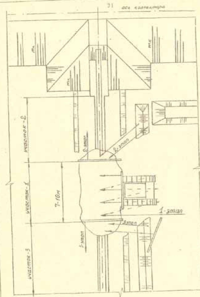
Рис. 9-а. Схема засылки траншеи дрена поперечно-продольным способом.
