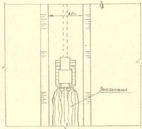
Рис. 9-г. Схема засыпки траншеи дрены с продольным рытанием грунта по трассе.
