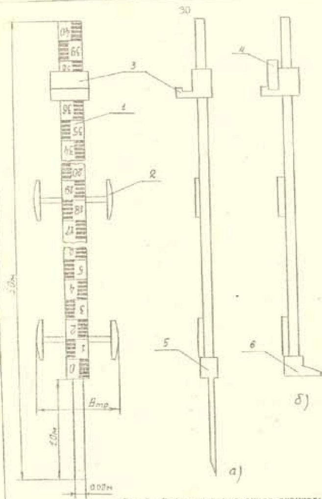
Рис. 8 Рейка нивелировочная специальная
