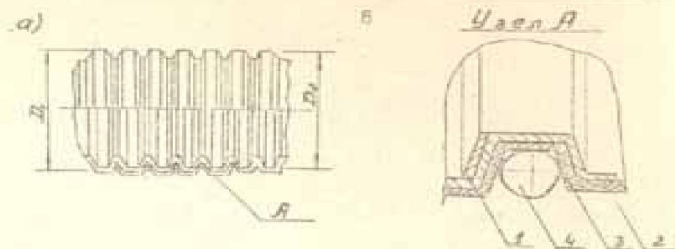
Рис.2-а. Схема соединения гофрированных труб, одинаковых по диаметру 1. Верхняя труба 2. Нижняя труба 3. Муфта из гофрированной трубы длиной 30-40 см 4. Жгут из базальтовой проволоки
