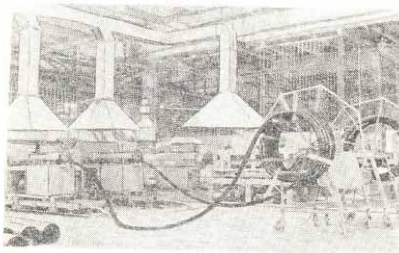
Технологическая линия по производству гофрированных полиэтиленовых дренажных труб ЛГДТ-75
