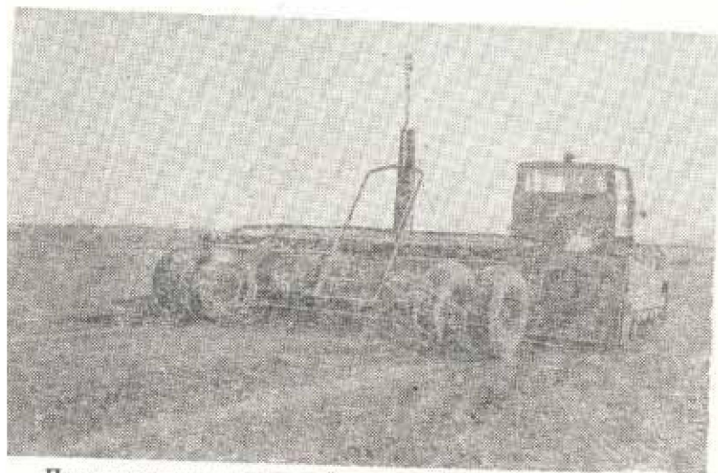
Планировщик с лазерной системой управления ПЛ-5
