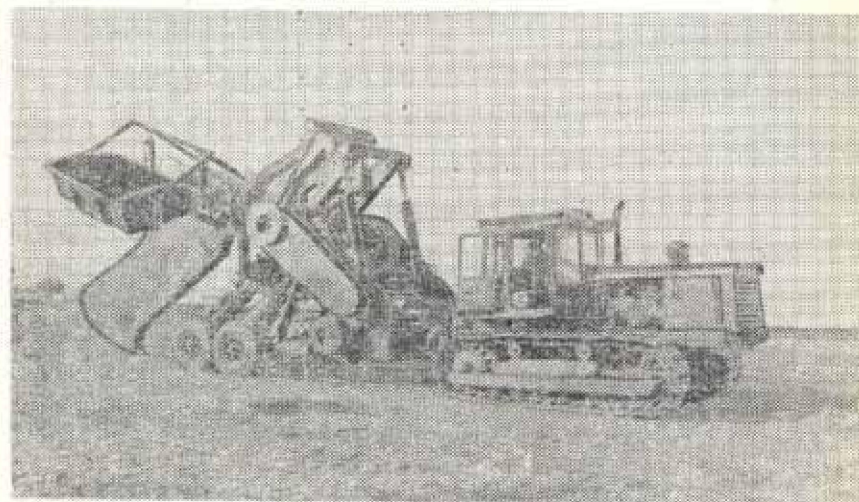
Дреноукладчик траншейный прицепной ДТП-4,0
