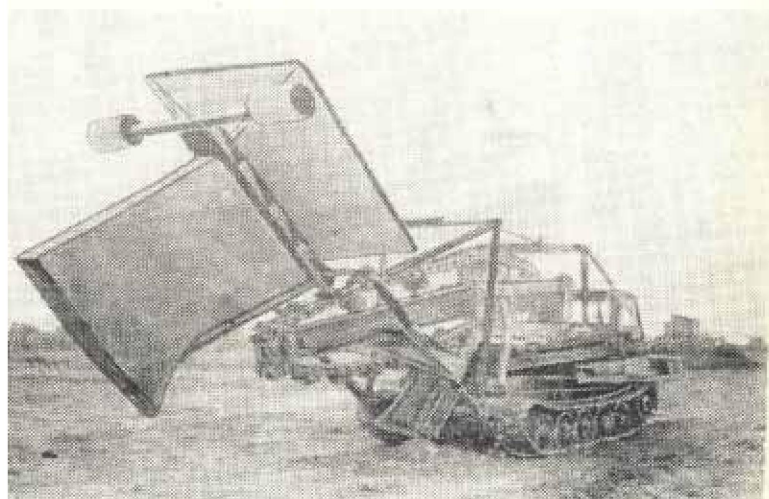
Дреноукладчик узкотраншейный ДУ-251
