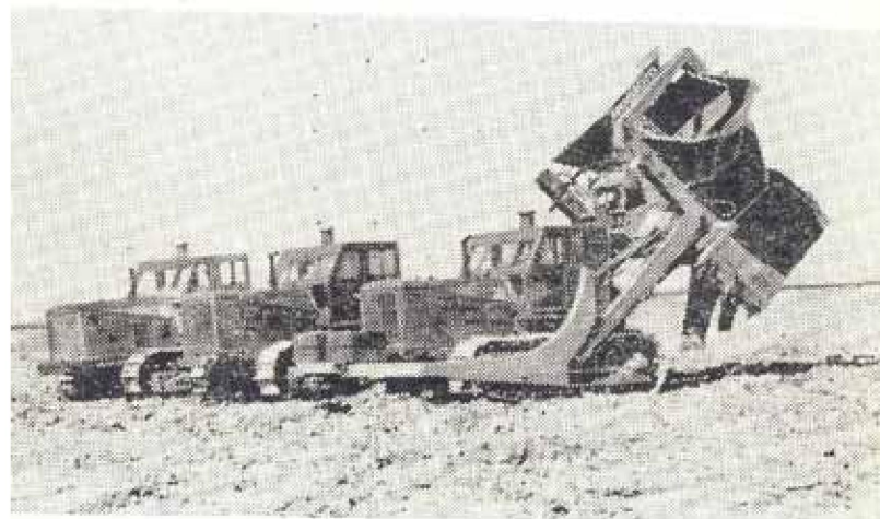
Дреноукладчик бестраншейный ДБ-2,0
