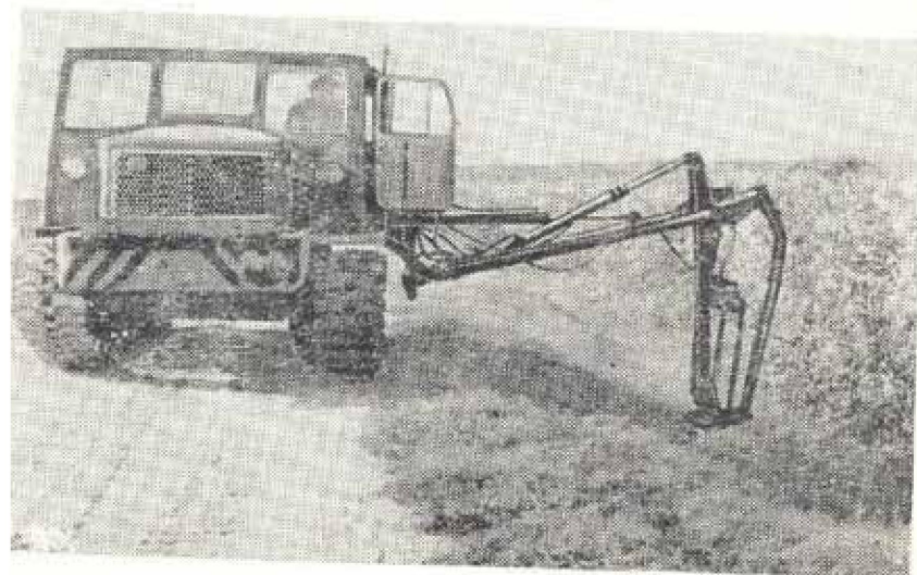
Косилка откосов коллекторов КОК-6
