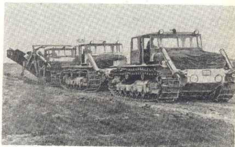
Дреноукладчик бестраншейный ДБ-251
