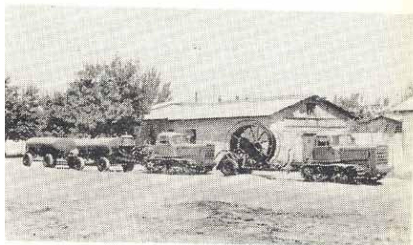
Промывщик дренажных труб ПДТ-125
