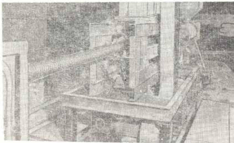
Технологическая линия по производству гофрированных полиэтиленовых дренажных труб ЛГДТ-110
