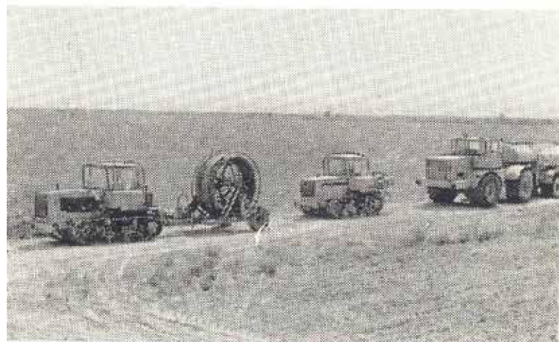
Промывщик коллекторов ПК-0,8
