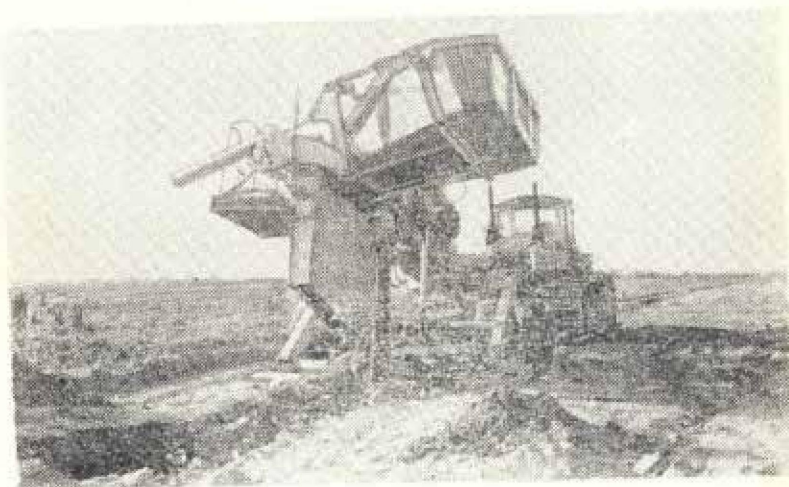
Дреноукладчик прицепной бестраншейный ДПБ-2,5
