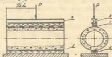
Рис. II, 1. Схема испытания пористой трубы:
