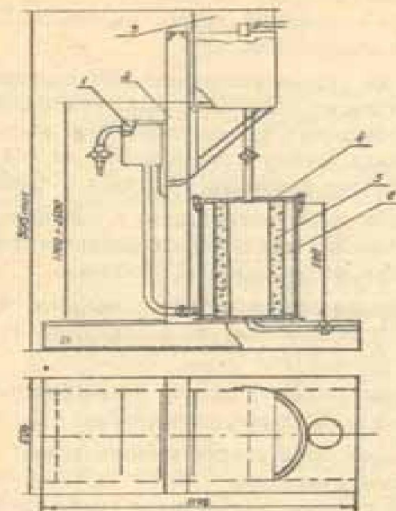
Рис. II, 2. Установка для определения фильтрационных характеристик пористых труб:
