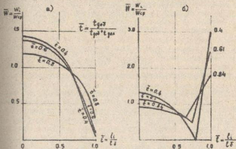
Графики отклонений от среднего инфильтрационного питания по длине борозды для гидроморфного и полугидроморфного режимов а) со сорохом в конце борозды; б) "тупиковые" борозды
