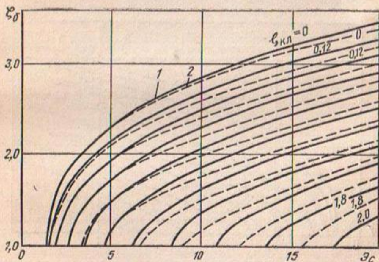
Рис. 8.7. Зависимость \zeta_6 от \mathcal{E}_c и \zeta_{кл} призматических русл прямоугольного и трапецидального сечений: 1— y_k=0 ; 2— y_k=0,025 (кривые даны через 0,2).
