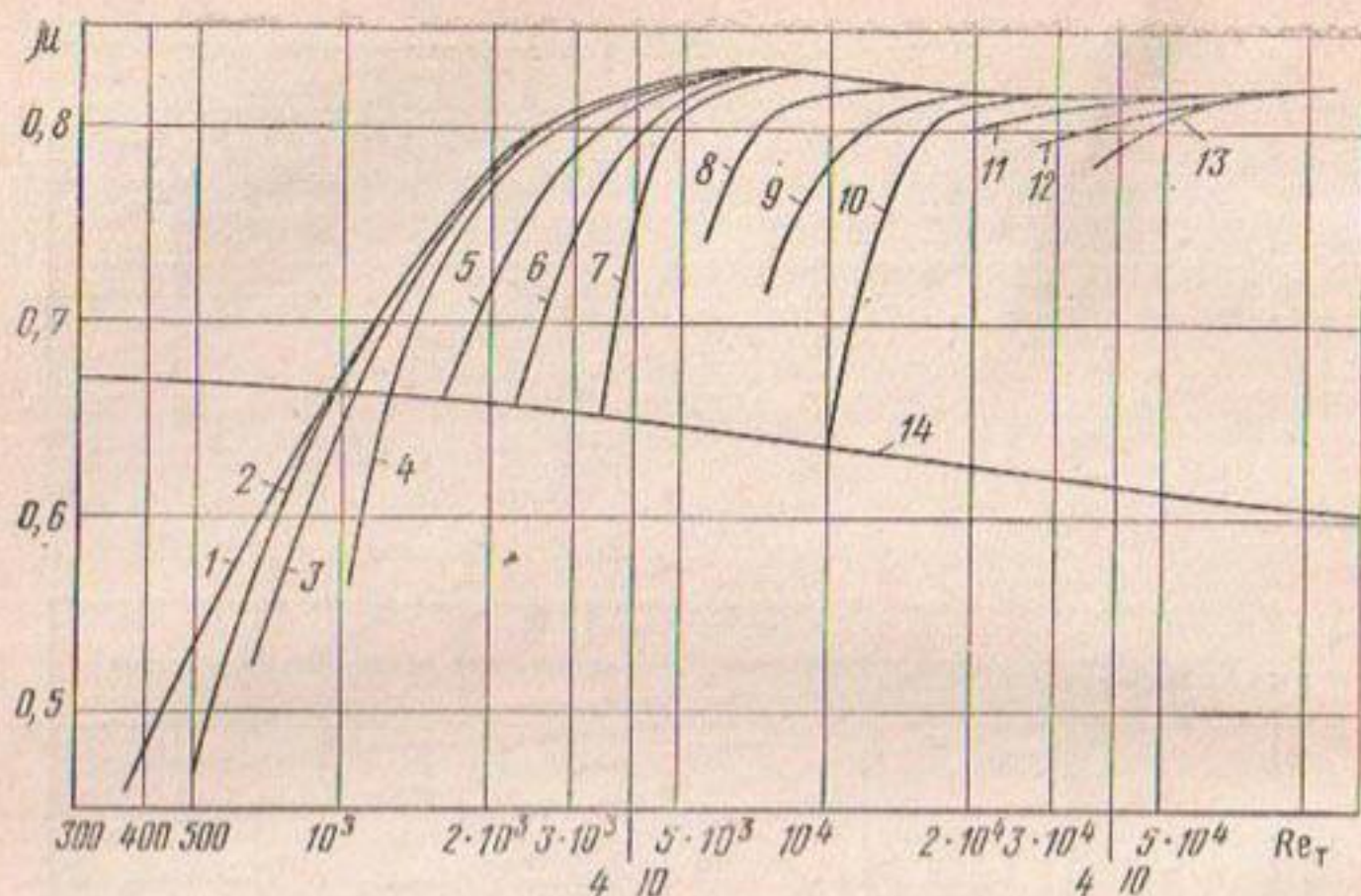
Рис. 5.27. Зависимость \mu от d , H_{ж} , Re_{\tau} при n_{в}=1 ; f=40 Гц: d — 1...4—0,3 мм; 5...7—1; 8...10—4; 11...13—10; H_{ж} —2, 5, 8, 11 — 100 мм; 3, 6, 9, 12—200; 4, 7, 10, 13—400; 1— n_{в}=0 .
