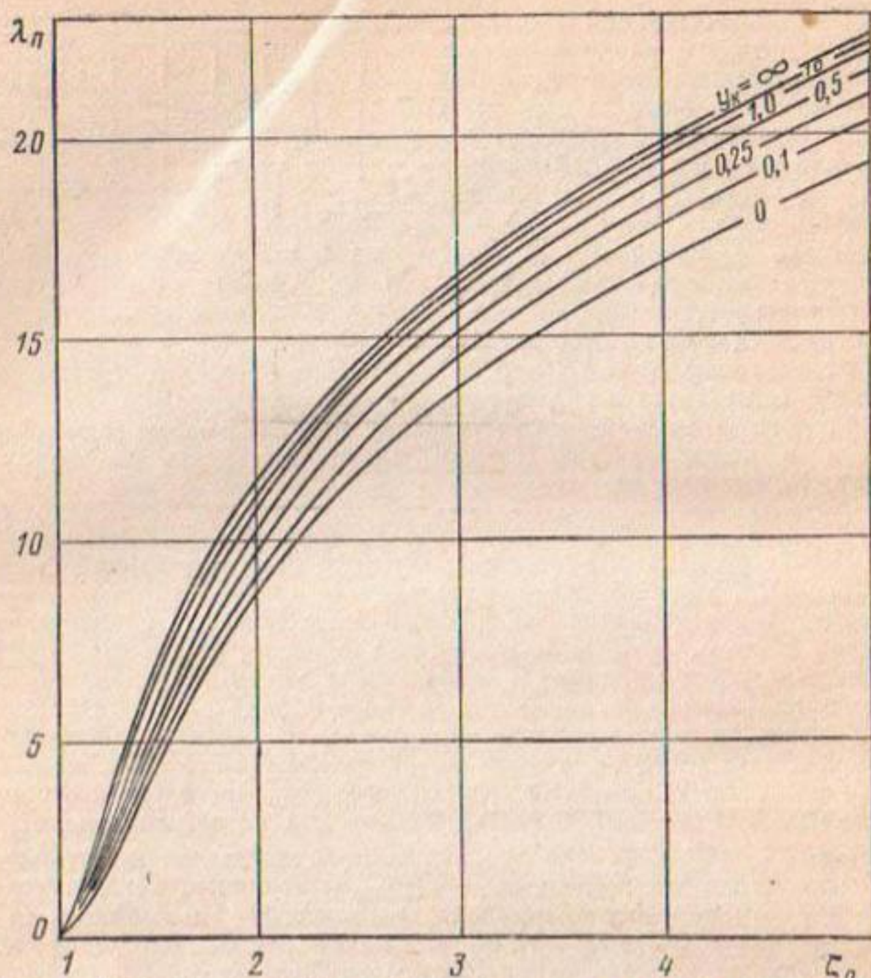
Рис. 8.5. Зависимость \lambda_{\text{п}} от \zeta_{\text{в}} и y_{\text{к}} для призматических русел, прямоугольного, трапецидального и треугольного сечения с горизонтальным дном.
