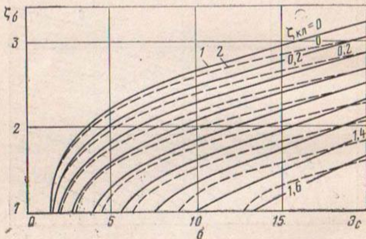
Рис. 8.8. Зависимость |\zeta_\delta| от \Delta_c и \zeta_{\kappa\lambda} для призматических русл трапецидального сечения: а— y_\kappa = 0,05 и 0,1 ; б— y_\kappa = 0,15 и 0,25 (кривые даны через 0,2 ).
