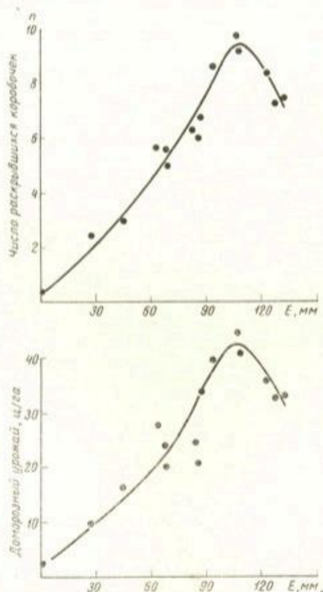
Рис. 1. Зависимость числа раскрывшихся коробочек и доморозней урожая хлопка-сырца от суммарного испарения ( E , мм) за период раскрытия первых коробочек—заморозок.
