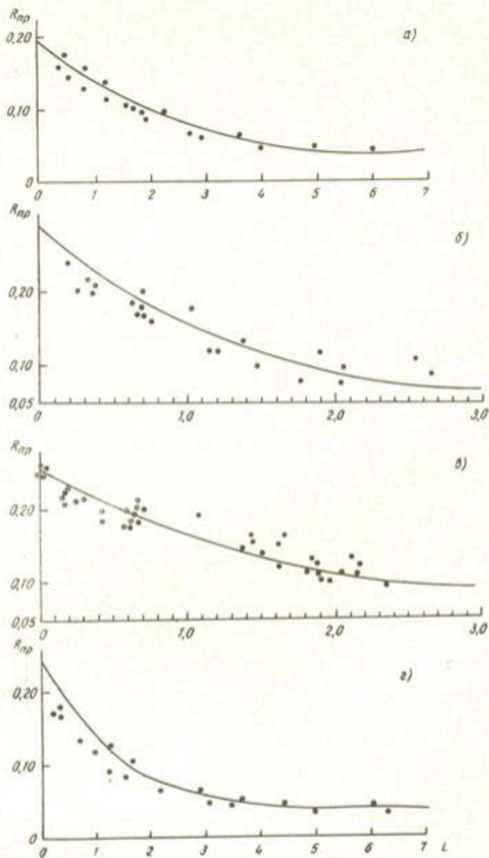
Рис. 3. Связь коэффициента яркости посевов сельхозкультур с индексом листовой поверхности: а — хлопчатник (108-ф), б — свекла (Уладовская 752), в — кукуруза (ВИР-42), г — пшеница (Красная Звезда 8702).
