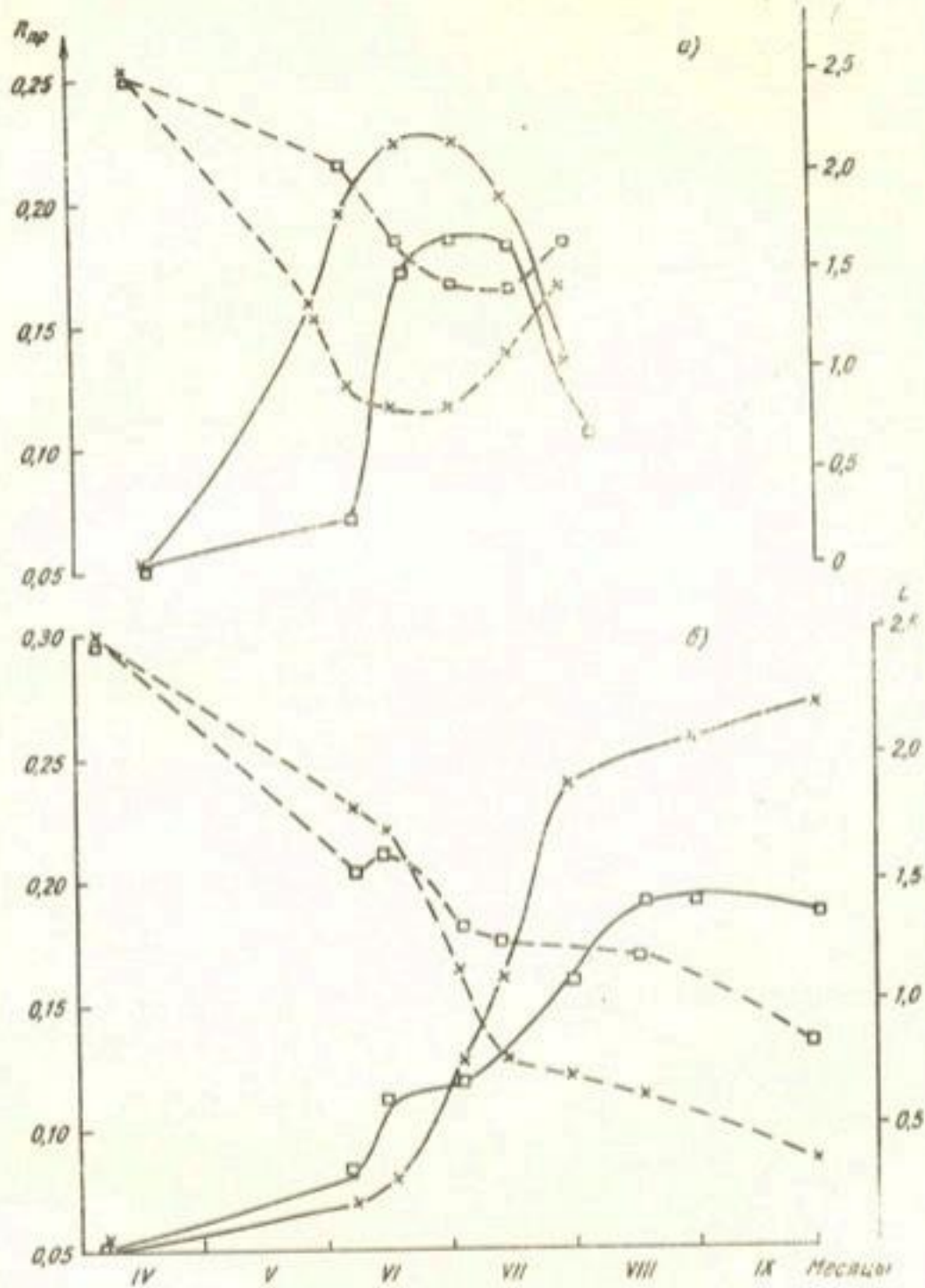
Рис. 2. Сезонный ход коэффициентов яркости R_{лр} в области спектра с \lambda_{эфф} = 628 нм и индекса листовой поверхности посевов кукурузы и сахарной свеклы. а—Кукуруза (Вир-42), б—сахарная свекла (Уладовская-752)
