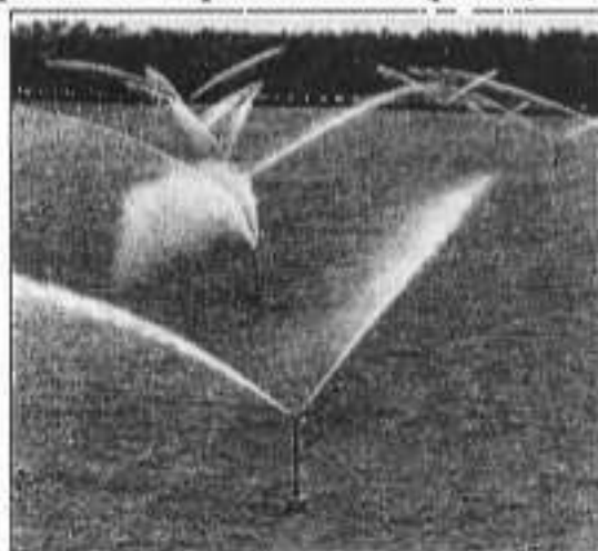
Рис. 46. Синхронно-импульсное дождевание
