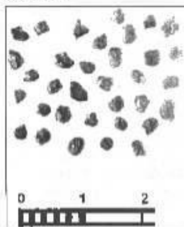
Рис. 10. Темно-серые марганцево-железистые орштейны из гор. A2 дерново-подзолистых сульфатных неглеевых почв
