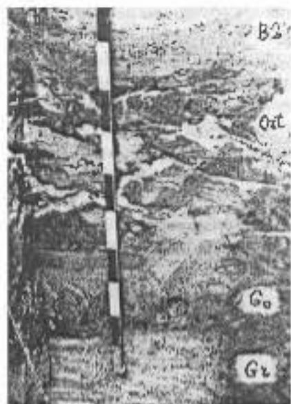
Рис. 6. Положение ортандового горизонта в профиле дерново-подзолистой естественной почвы, заболоченной глинистыми грунтовыми водами. Ортандовый горизонт залегает над валунами Окско-Менчёрского полого
