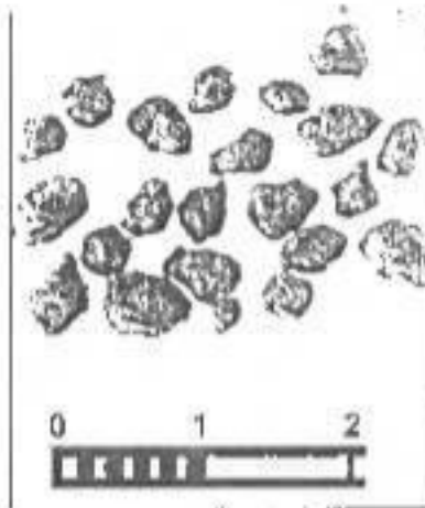
Рис. 11. Бурые железистые орштейны из гор. A2 дерново-подзолистых сульфатных глееватых почв
