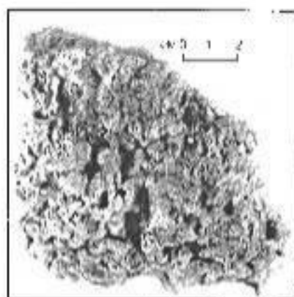
Рис. 7. Рудяковый панцирь (рудяковый отдельности) из дерново-слабоподзолистой глеевой рудяковой почвы, заболоченной сильно-окисленными грунтовыми водами. Окско-Мещерские леса
