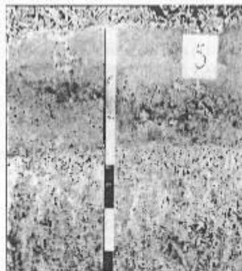
Рис. 10. Темно-серые марганцево-железистые орштейны из гор. A2 дерново-подзолистых сульфатных неглеевых почв
