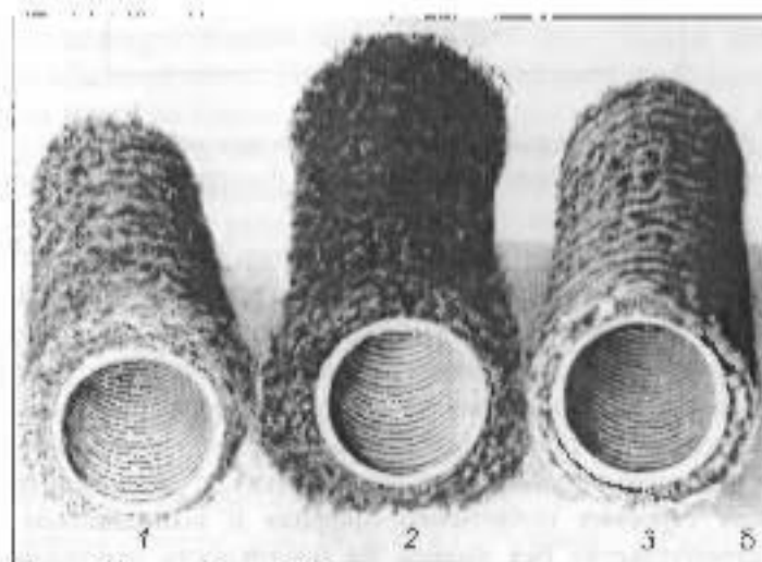
Рис. 27, а — трубчатые перифитические и б — пластмассовые дрени с объемными фильтрами из коксового волокна (1), торфа (2) и соломы (3)
