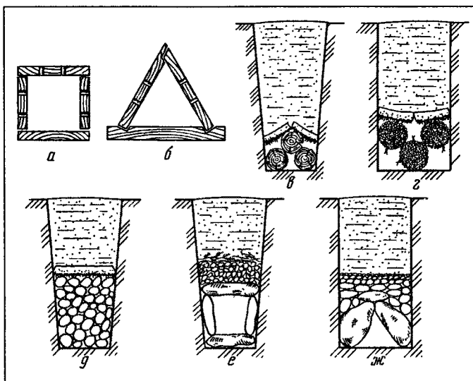
Рис. 29. Виды деревянного и каменного дренажей, выполненных вручную: а, б — деревянные дощатые дрена; в — жердевая дрена; г — фашинная дрена; д, е, ж — каменные дрена.
