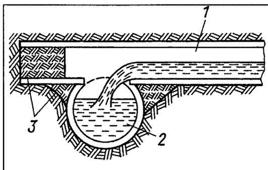
Рис. 28. Сопряжение керамической дрены с коллектором: 1 — керамическая дрена; 2 — коллектор; 3 — глинистая заглушка
