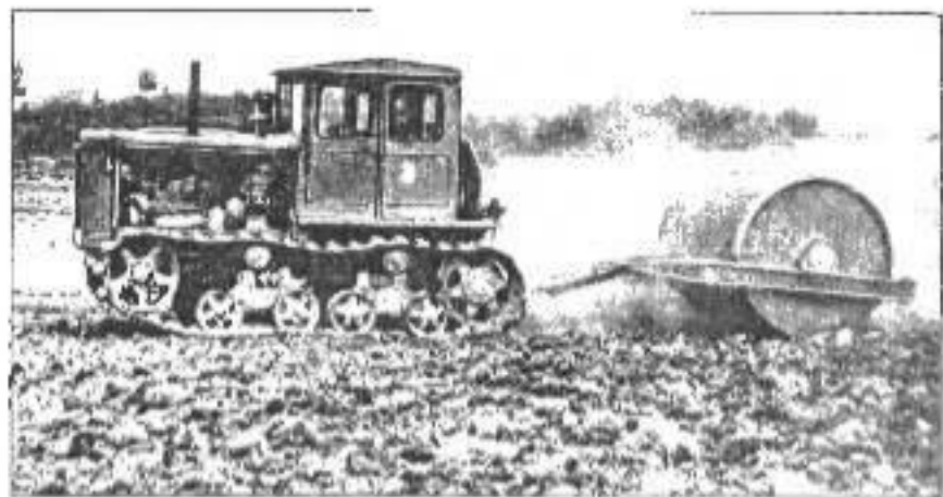
Рис. 45. Прикатывание торфяных почв водонепроницаемым катком для восстановления гидрологической связи пахотного и подпахотного горизонтов в осушенных торфяных почвах
