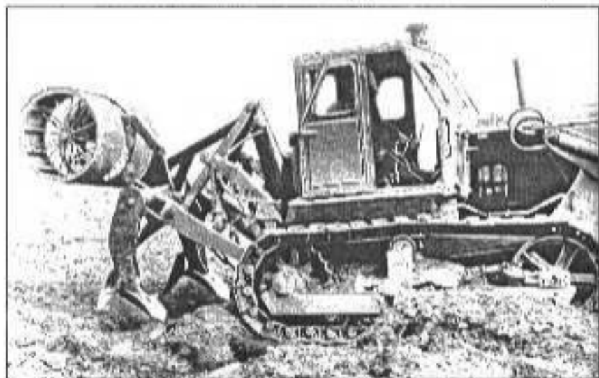
Рис. 34. Рыхлитель-кротователь универсальный РУ.65.2,5. Рыхлитель пассивного действия
