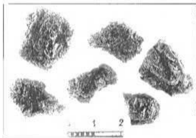
Рис. 13. Черные угловатые гумус-алюминиевые конкреции из гор. А1 дерново-степных почв
