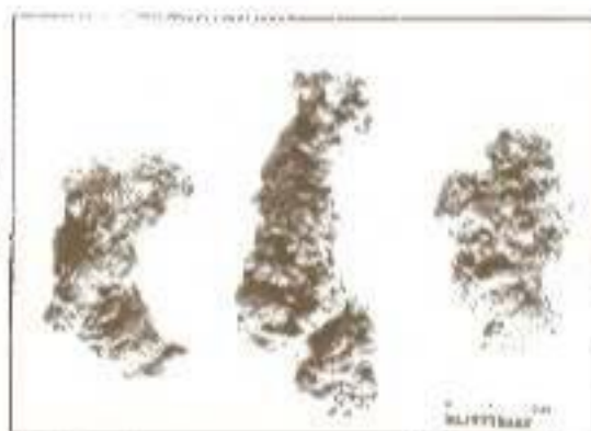
Светлые угловатые известковые конкреции. Индикатор на заболачивание почвы жесткими грунтовыми водами
