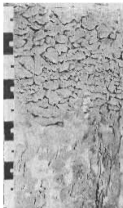
Рис. 8. Железистые коры в профиле луговых сильноокисленных глеевых почв. Окско-Метлицкое поле
