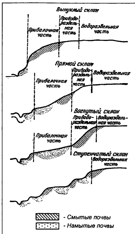
Рис. 56. Расположение смытых и намытых почв по профилю склонов различной формы (по Сусу, 1959)
