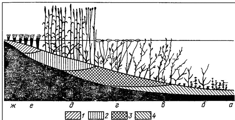
Рис. 17. Заболачивание в результате зарастания водоема (по Сукачеву, 1926). Условные обозначения: 1 — осоковый торф; 2 — тростниковый торф с примесью камыша; 3 — торфянистый сапропель; 4 — смешанно-водорослевый сапропель
