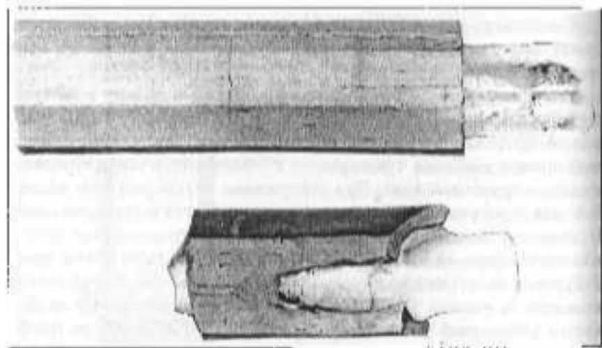
Рис. 32. Закупорки и разрушение керамической дренажа ледовыми пробками. Бийская низменность, Западная Сибирь (фото Н. Н. Логина)
