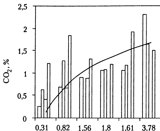
Рис. 8.1. Концентрация \text{CO}_2 в почвенном воздухе разных почв
