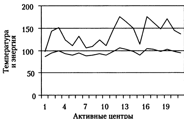
Рис. 13.1. Характеристика активных центров по температуре (1 °С) и энергии (2 Дж) удаления аммиака
