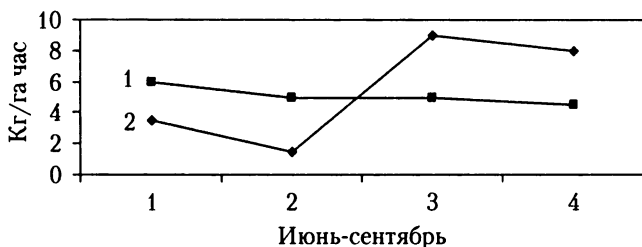
Рис. 8.3. Выделение \text{CO}_2 из дерново-подзолистой почвы в дубо-ельнике осокововолосистом в еловой (1) и дубовой парцеллах (2)
