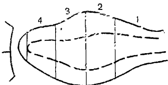
Рис. 19. Схема работ по выполаживанию оврагов, разработанная А. Г. Рожковым
