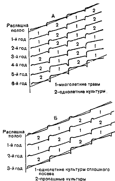
Рис. 15. Схема формирования напашных террас при чересполосном освоении склонов:
