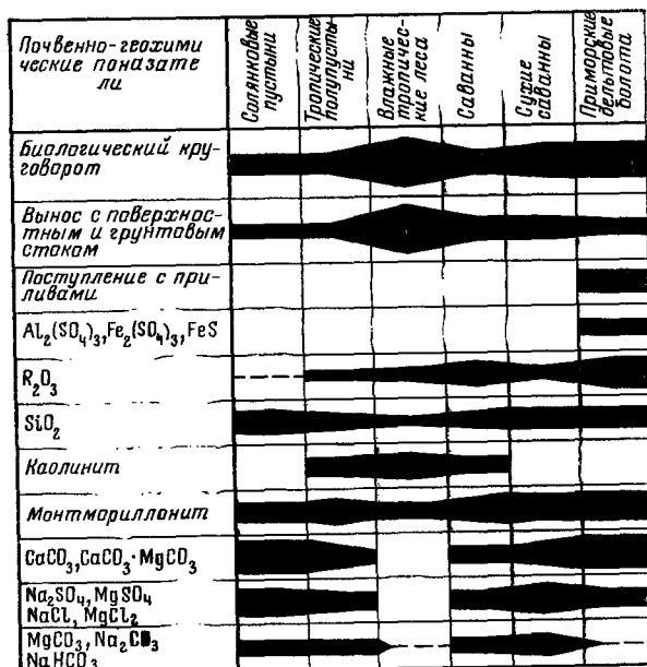
Рис. 63. Диаграмма почвенно-геохимических особенностей дренированной части континента типа Африки и Южной Америки (Глазговская, 1967, с добавлениями и изменениями автора)
