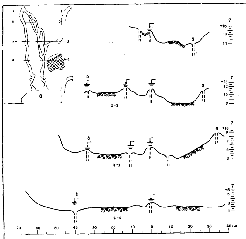
Рис. 104. Поперечные профили через дельтовую область (3—4) и нижнее течение (1—2) рек, впадающих в Тайландский залив (Masahiko, 1966)
