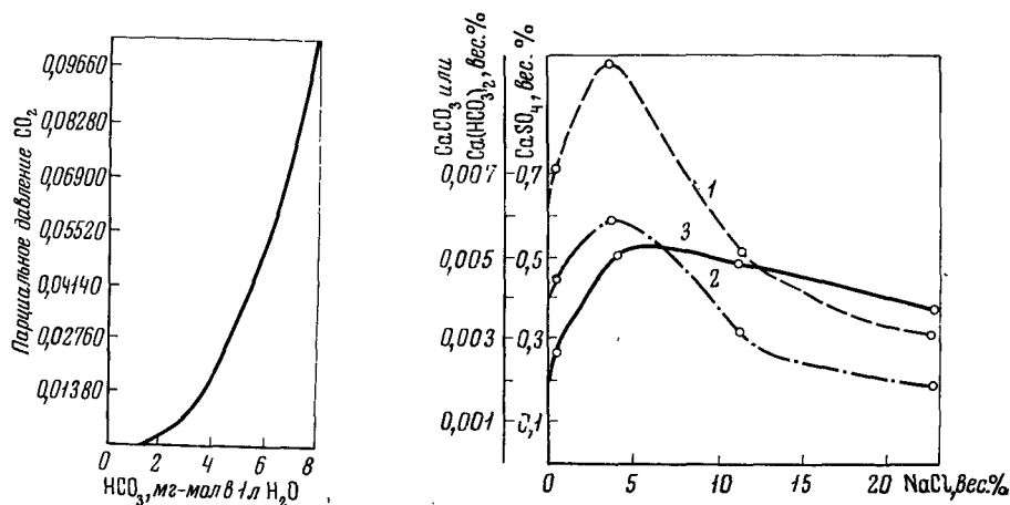
Рис. 34. Растворимость \text{CaCO}_3 в зависимости от парциального давления \text{CO}_2 в атмосфере при 25^\circ\text{C}
