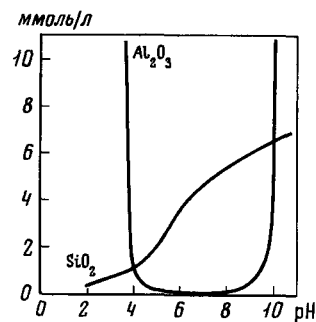
Рис. 36. Растворимость кремнезема и глинозема в зависимости от величины pH (Correns, 1949)
