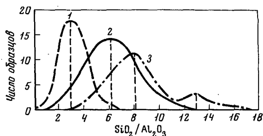
Рис. 41. Отношения \text{SiO}_2/\text{Al}_2\text{O}_3 в илнстой фракции, мелкозем и породах в ортоэлювии холодных гумидных областей (Таргульян, 1967)
