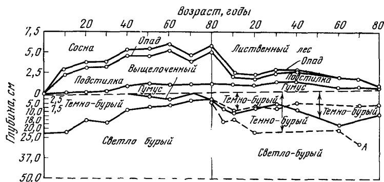
Рис. 78. Изменение характера почвы на пашне, затем под сосной и далее под лиственными насаждениями (Гриффи и др., по Йенни, 1948)
