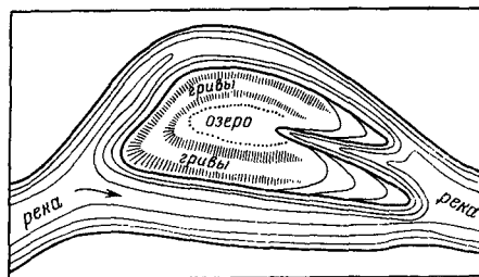
Рис. 96. Схема образования острова (Плюснин, 1938б)
