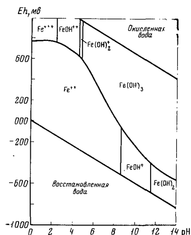
Рис. 38. Поля устойчивых водных систем (Иетт, Сгоррег, 1959)
