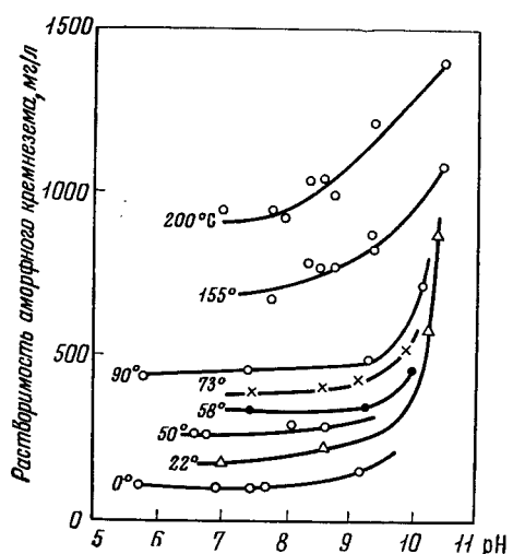
Рис. 42. Влияние pH и температуры на растворимость аморфного кремнезема (Osumoto а. о., 1957)
