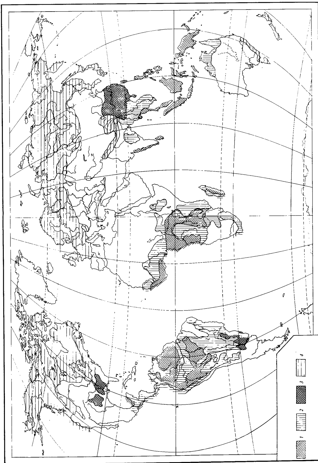
Рис. 79. Схема распространения формации кислых каолинитово-гидролюбивых почв
