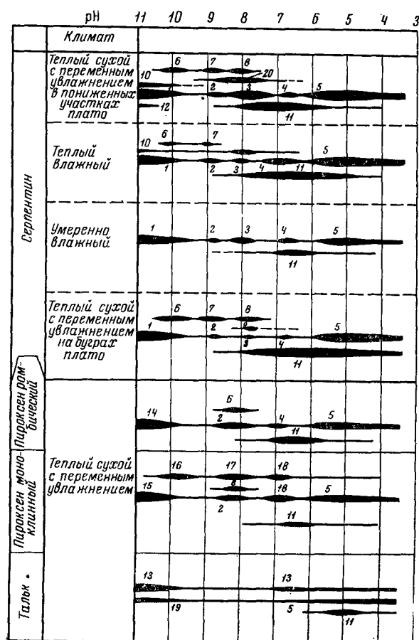
Рис. 30. Схема возможных стадий выветривания главных минералов ультраосновных пород в зависимости от рН (Гинзбург, 1947)
