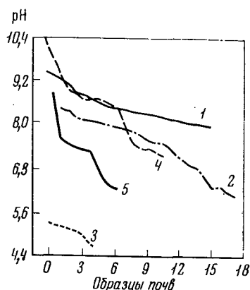
Рис. 110. Варьирование pH в верхнем горизонте луговых почв восточных областей КНР (Ковда, 1959)
