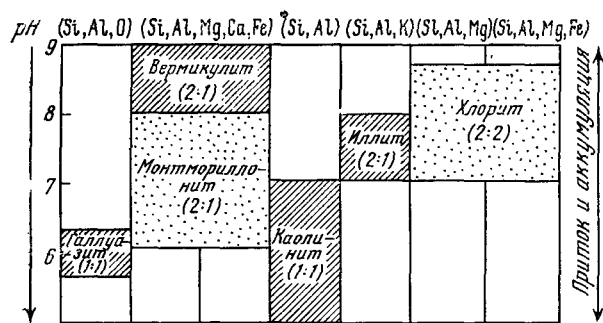
Рис. 26. Условия формирования вторичных минералов (Degens, 1965, с изменениями автора)
