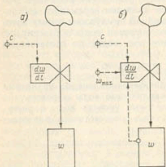
Рис. 12. Схема связей для систем заполнения водой резервуара.
