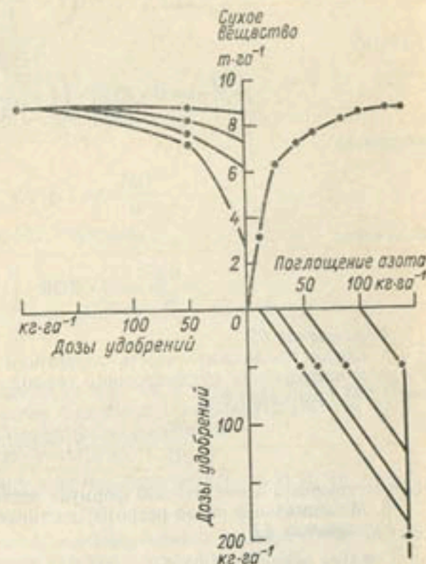
Рис. 93. Рассчитанные связи между дозами удобрений, поглощением азота и урожаем сухого вещества для четырех уровней доступности азота в неудоженной почве.
