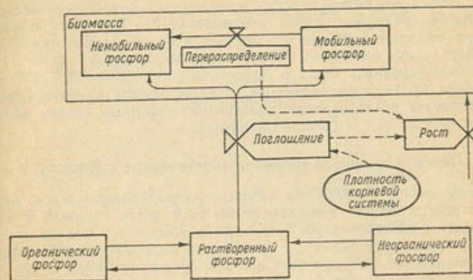
Рис. 5. Схема основных связей системы на четвертом уровне продуктивности, где дефицит фосфора P является главным лимитирующим фактором.
