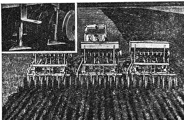
Рис. 21. Сеялка-культиватор СЗС-2,1.
