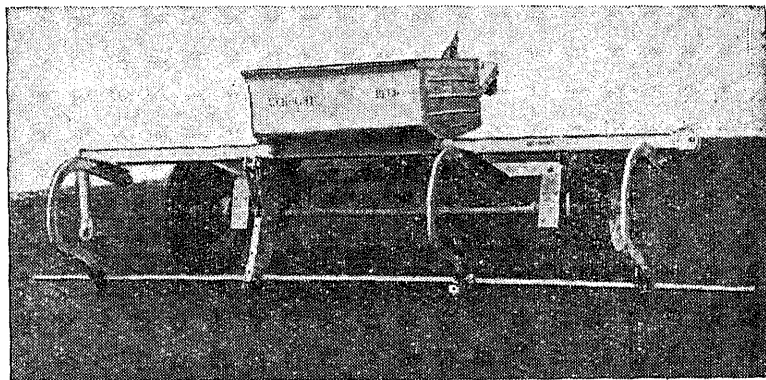
Рис. 15. Культиватор штанговый КШ-3,6.
