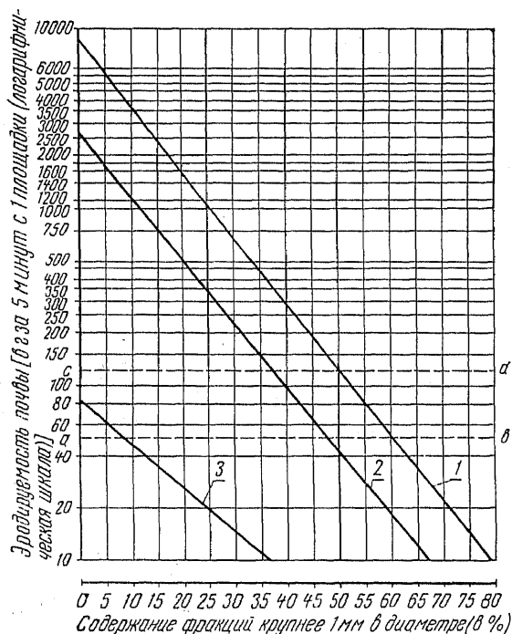
Рис. 3. Изменение эродруемости почвы в зависимости от комковатости поверхности при различной скорости воздушного потока в ПАУ-2 на высоте 50 см:
