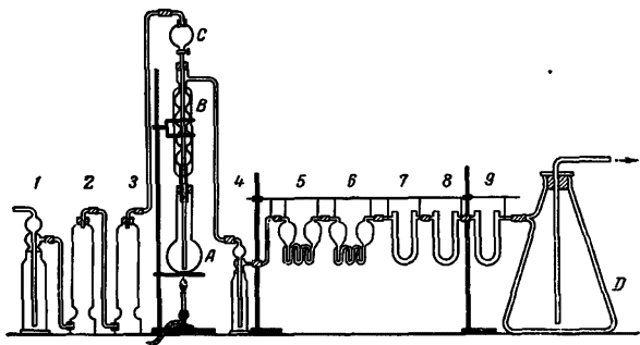
Рис. 2. Аппаратура для определения углерода по методу мокрого сжигания
