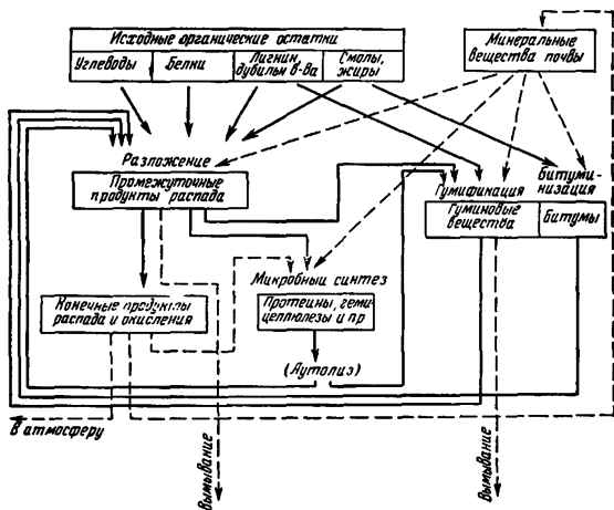
Схема процессов превращения органического вещества в почвах
