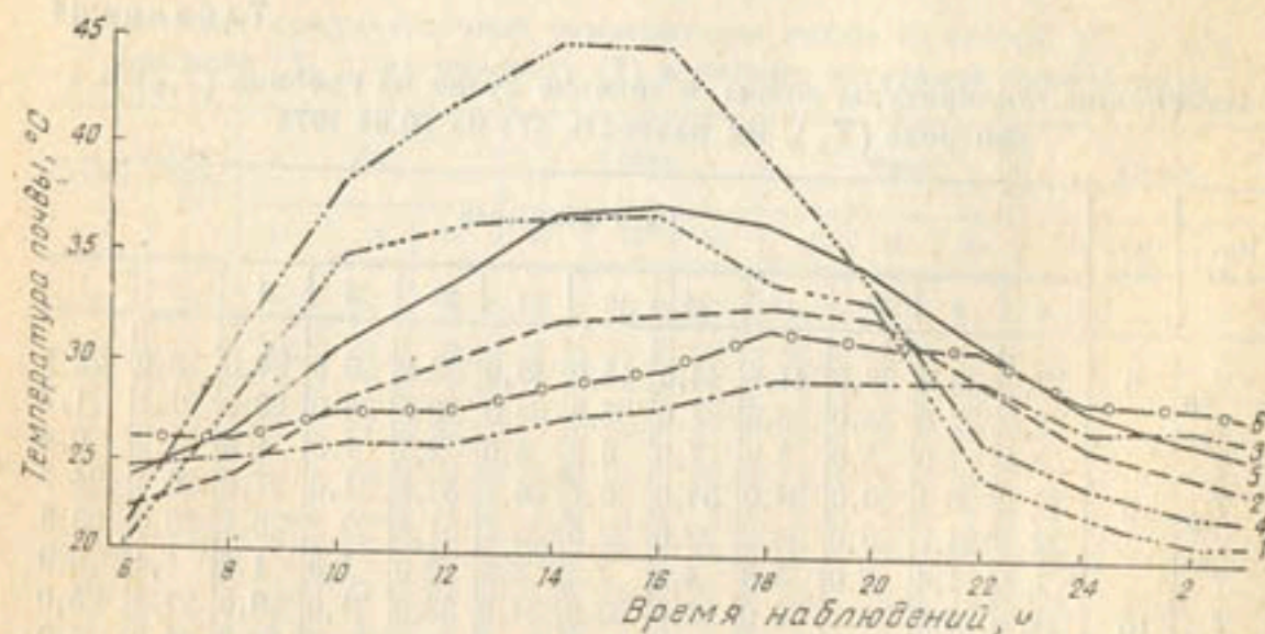
Рис. 7. Динамика температуры почвы в течение суток на гладком поле (1, 2, 3) и грядках (4, 5, 6).
