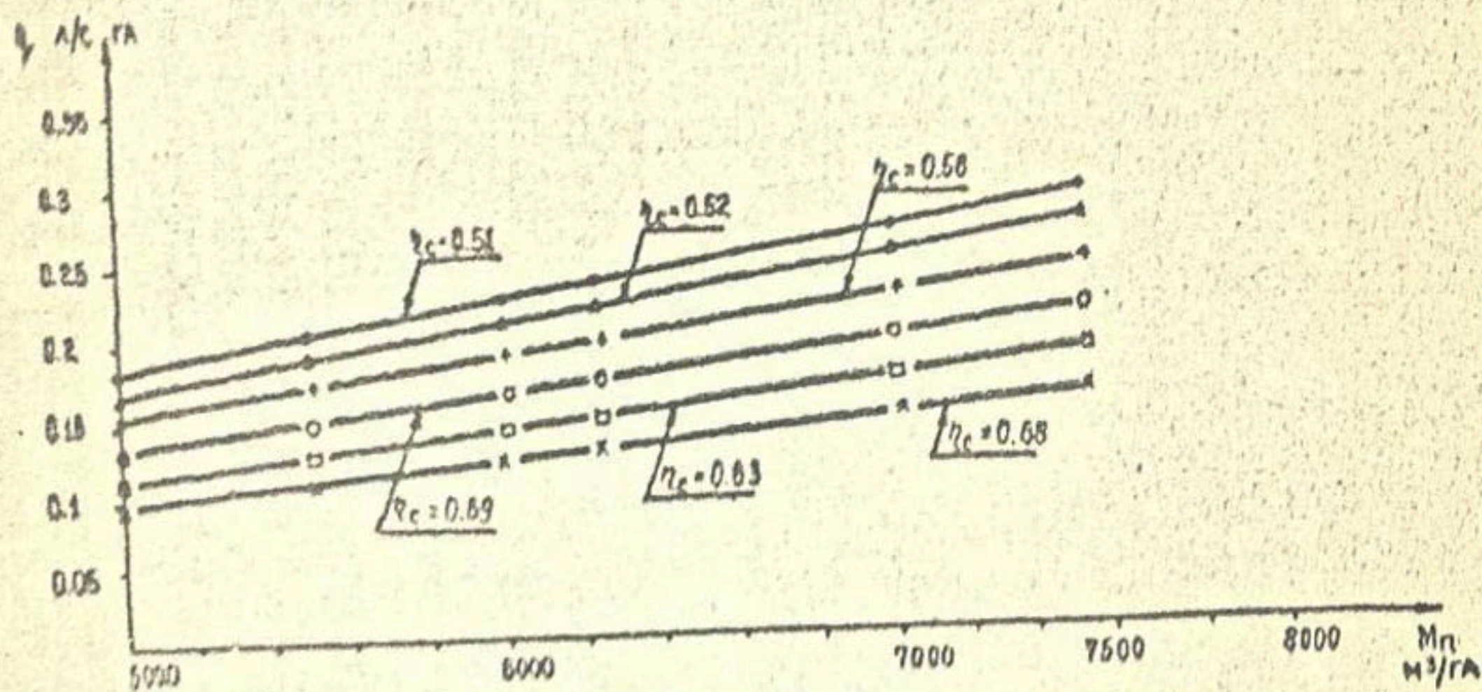
Рис. 7. Зависимость вегетационного дренажного модуля от оросительного модуля при различных \eta_c системы Нигиаринского района.
