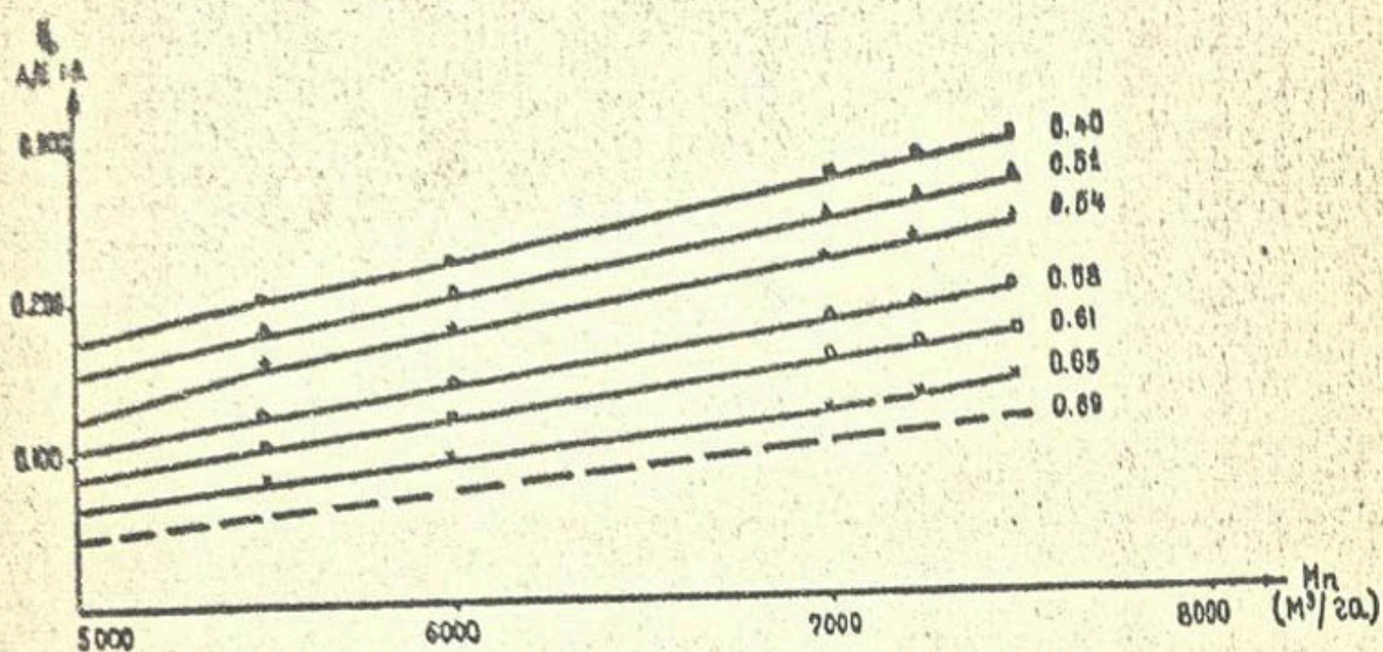
Рис. 2 Зависимость вегетационного аренажного модуля от оросительной нормы при различных К.П.Д системы по Богатскому району.
