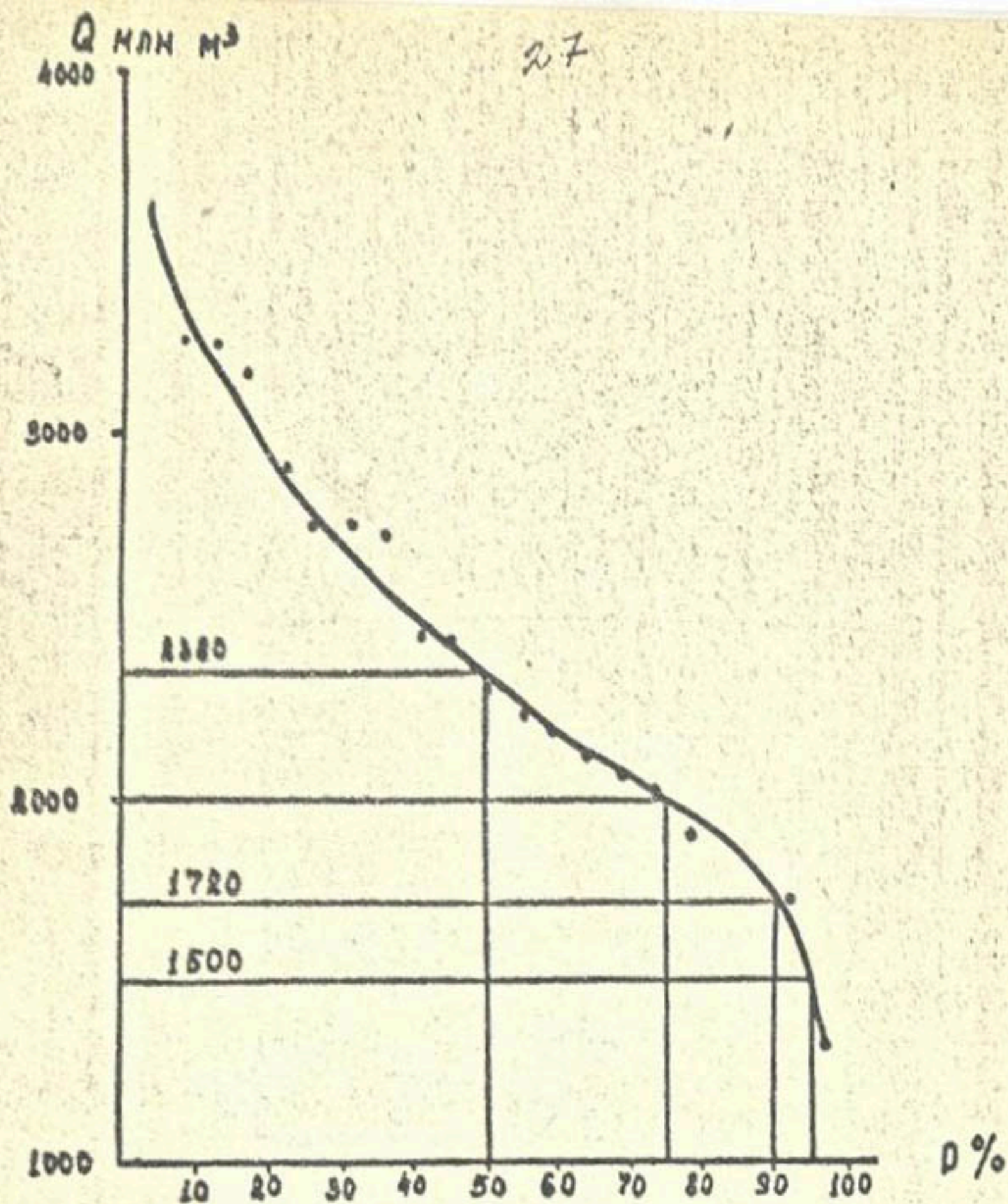
Рис. 1 Эмпирическая кривая обеспеченности годового стока КДС (млн.м³) по Хорезмской области. за 1966 - 1986 г.
