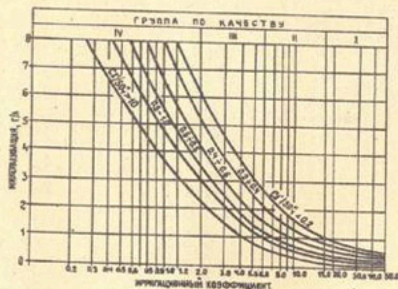
Рис. 3.1. Зависимость ирригационного коэффициента от общей минерализации при различных соотношениях Ca^{2+}/SO_4^{2-} .
