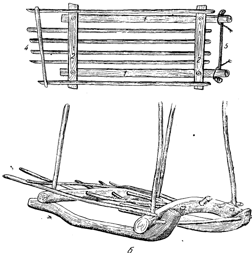
Рис. 6. Сани-волокуша «чигина»: 1 — кашкорак; 2 — болиштак; 3 — поия; 4 — раучу; 5 — бинникаш
