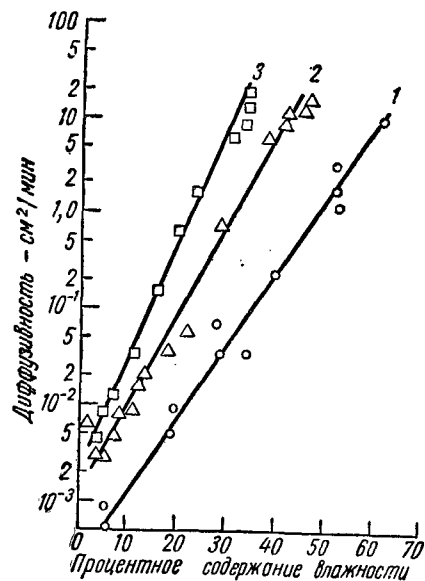
Рис. 65. Зависимость диффузивной проводимости влаги разных почв от их влажности (по Ричардсу): 1 — почва из Китая (Chino); 2 — почва из Индии (Indio); 3 — почва из Пахаппа (Pachappa)
