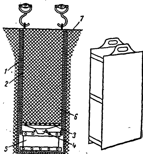
Рис. 85. Поперечный разрез испарителя в собранном виде:
