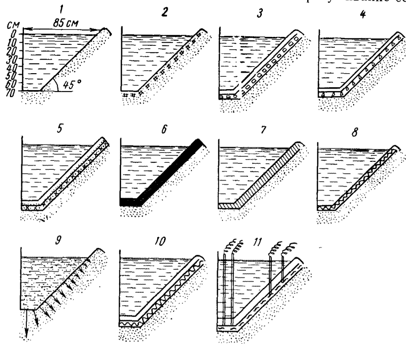
Рис. 43. Схема поперечного сечения через 11 вариантов опытных колодцев с противofильтрационной одеждой (кроме № 1)
