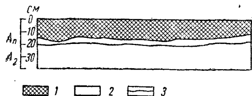
Рис. 19. Характер проникновения дождевой воды в супесчаную почву. Собакино-опытное, Московской обл. (зарисовка автора с натуры в профиль):
