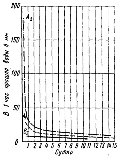
Рис. 14. Динамика водопроницаемости различных генетических горизонтов дерново-подзолистой суглинистой почвы. Собакино-опытное, Московской обл. Пашня (данные автора)
