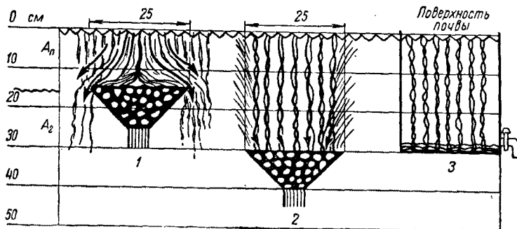
Рис. 31. Поступление фильтрующейся воды в ворончатые открытые лизиметры:
