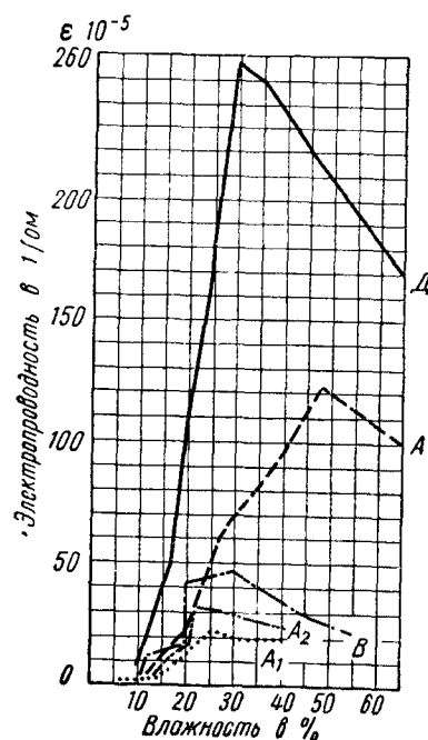
Рис. 101. Электропроводность почв в обратных омах. Дерново-подзолистая тяжелосуглинистая почва: гор. А 1 , А 2 , В; чернозем обыкновенный, гор. А и материнская порода — Д (лёссовидный суглинок) с глубины 370—400 см
