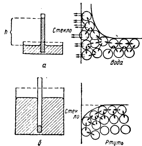
Рис. 52. Смачивание и несмачивание жидкостями твердых тел (по А. Митчерлиху): а — капиллярное всасывание; б — капиллярное давление
