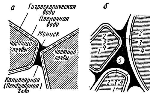
Рис. 66. Различные стадии увлажнения почвы. Гигроскопическая, пленочная и пендулярная (а) и фуникулярная (б) вода:
